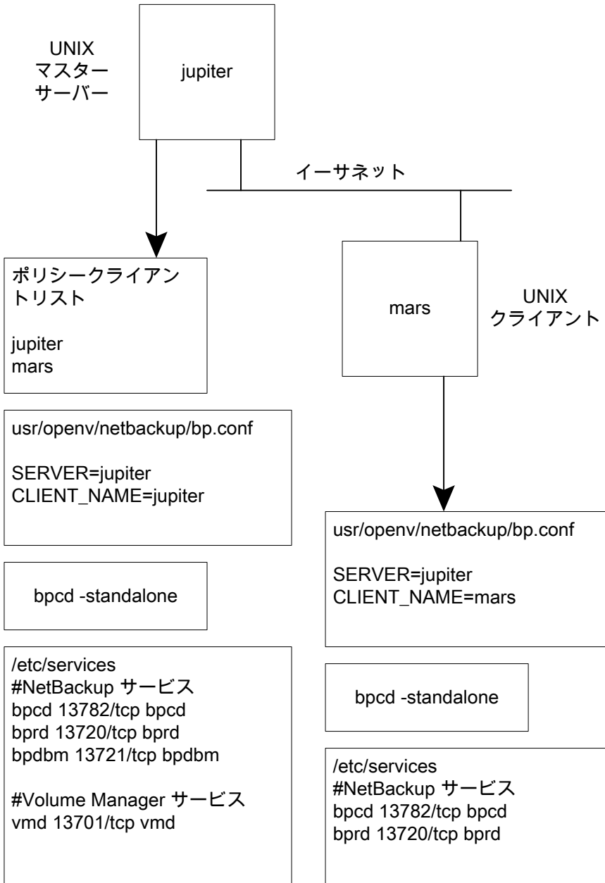
図 2-1 UNIX プライマリサーバーおよびクライアント
