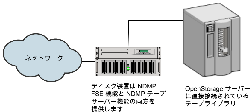
図 2-1 すべての NDMP 機能を提供する OpenStorage サーバー
