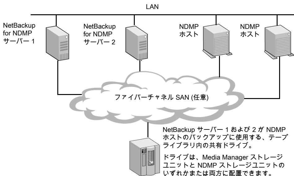
図 20-1 Shared Storage Option を使用した NDMP バックアップ
