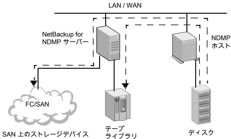
図 13-4 Media Manager デバイスへの NDMP バックアップ (リモート NDMP)
