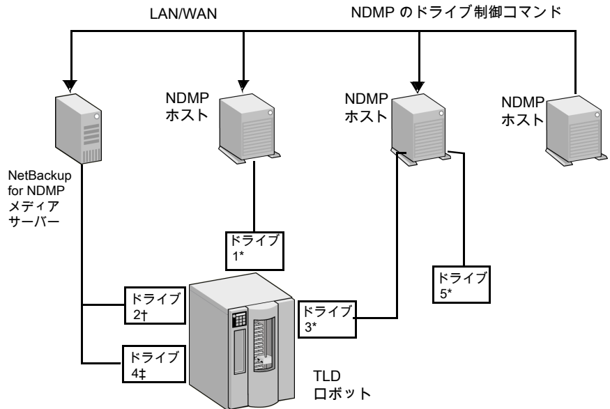
図 13-5 NDMP および非 NDMP のストレージユニット
