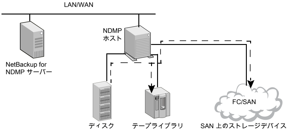
図 13-2 NDMP ローカルバックアップとリストア
