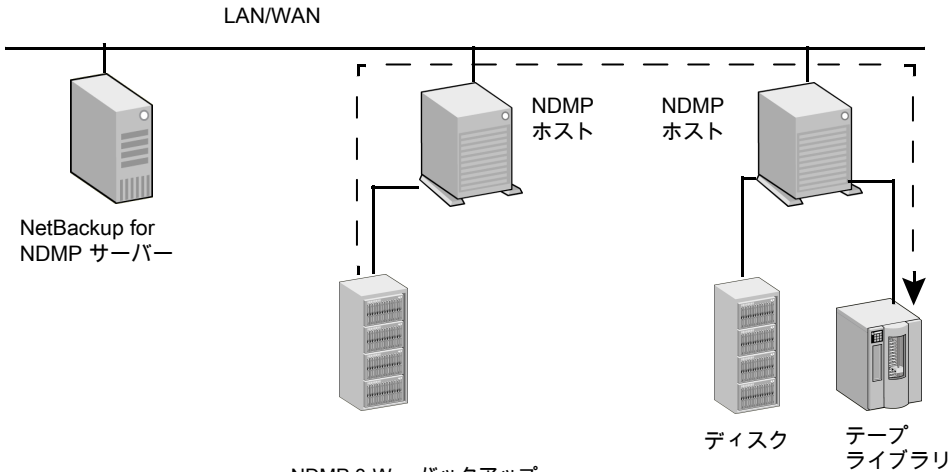
図 13-3 NDMP 3-Way バックアップとリストア
