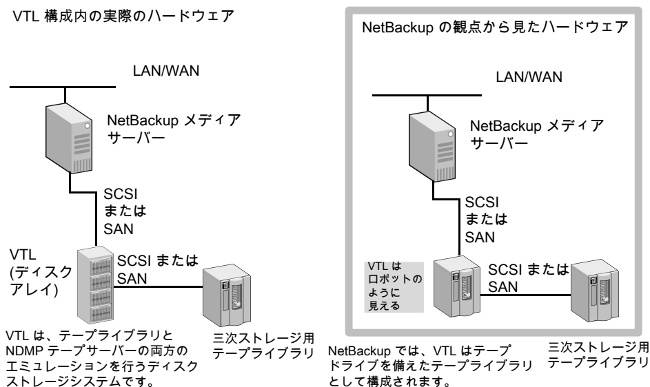
図 17-1 VTL を使用した NDMP ダイレクトコピーの概要
