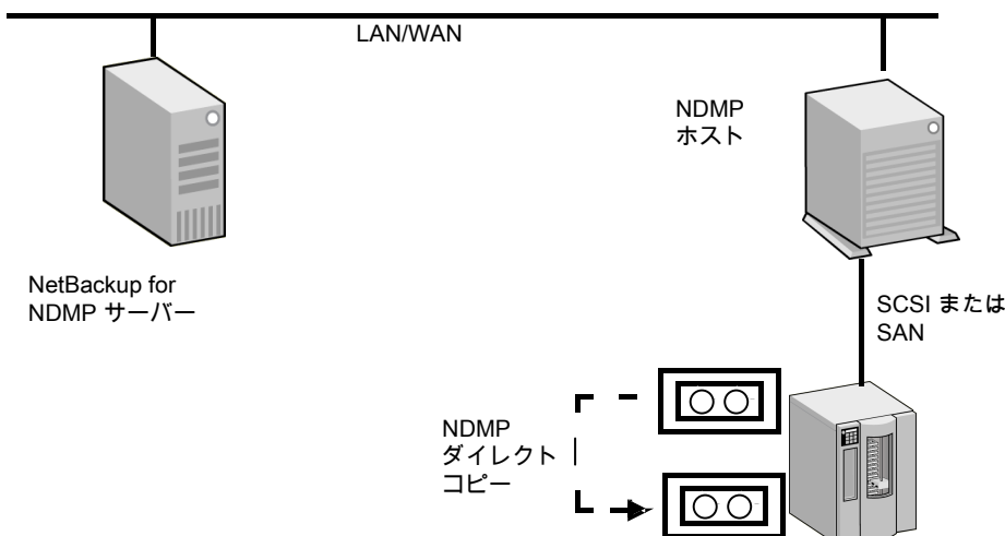
図 17-3 NDMP ホストにアクセス可能なテープドライブ間の NDMP ダイレクトコピー
