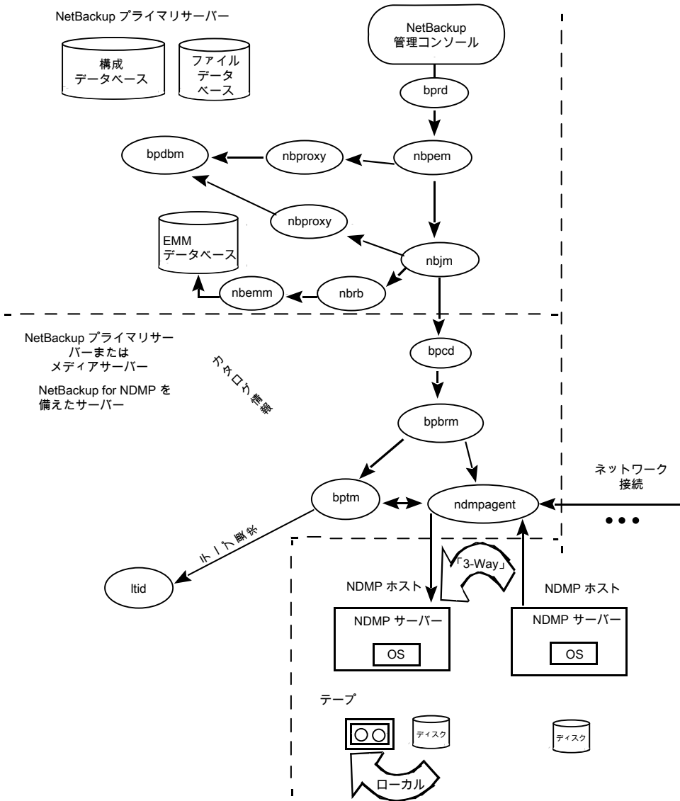
図 13-8 NetBackup のバックアップ処理
