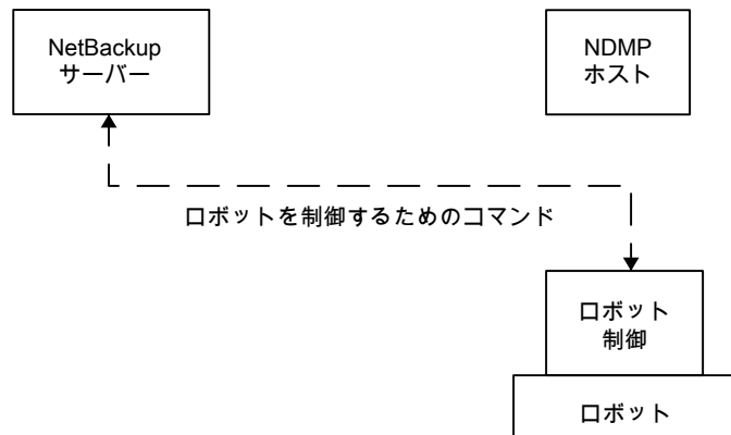
図 13-7 NetBackup サーバーに接続されたロボット制御
