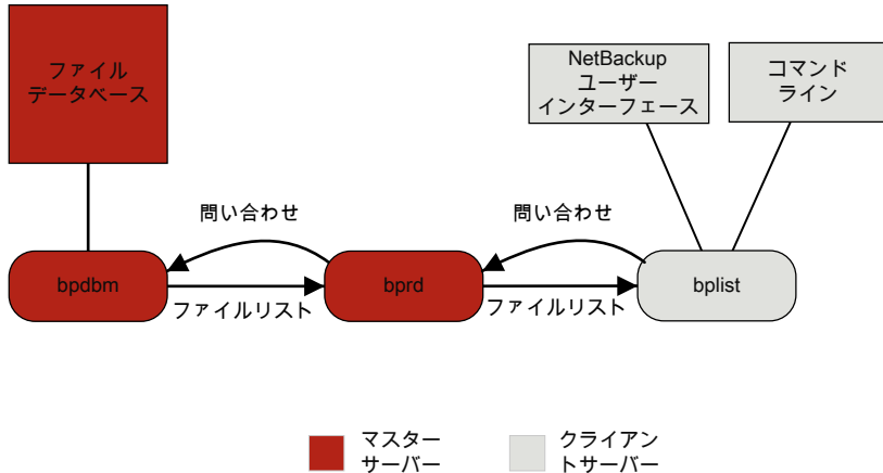
図 4-3 リストアの処理 - UNIX クライアント
