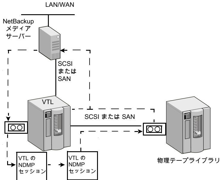
図 16-2 VTL を使用した NDMP ダイレクトコピーのデータの流れおよび制御
