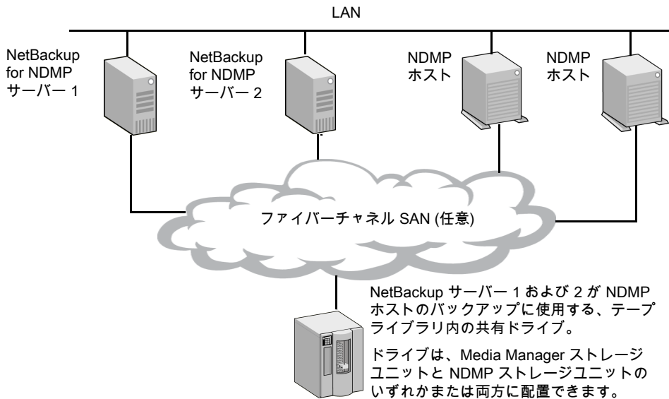
図 19-1 Shared Storage Option を使用した NDMP バックアップ
