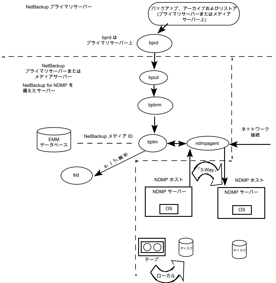
図 12-9 NetBackup のリストア処理
