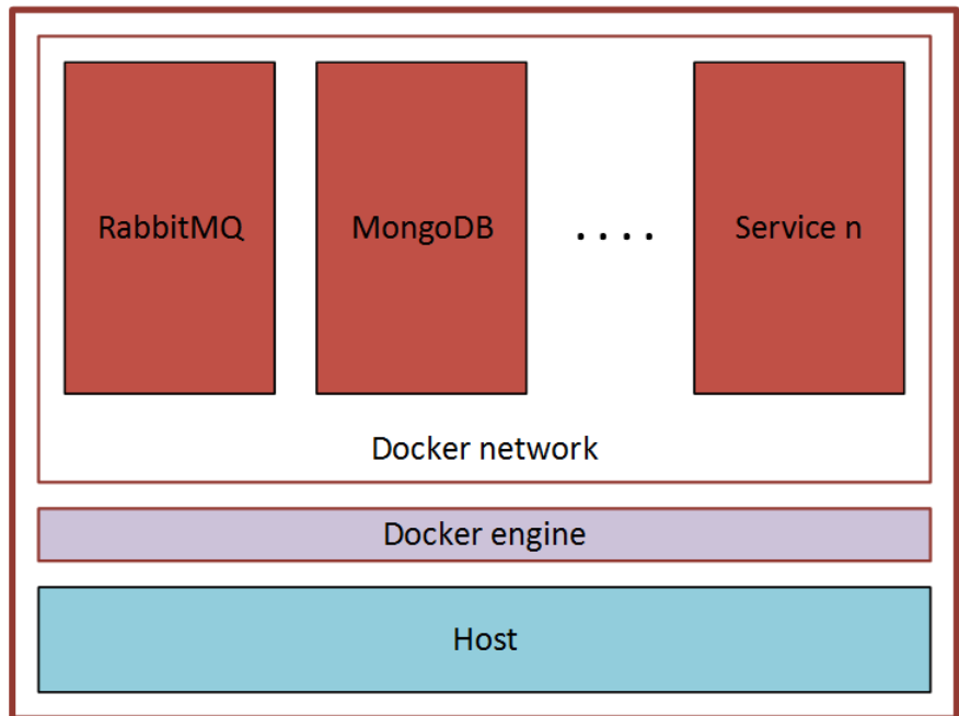
図 1-1 NetBackup Snapshot Manager のマイクロサービスモデル
