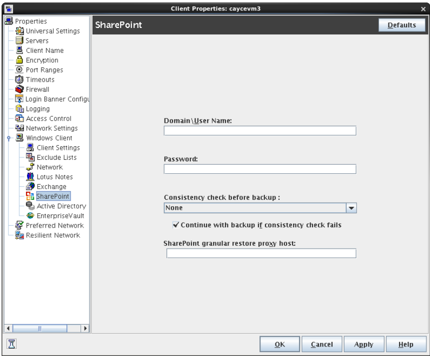
図 4-1 [SharePoint] ダイアログボックス
