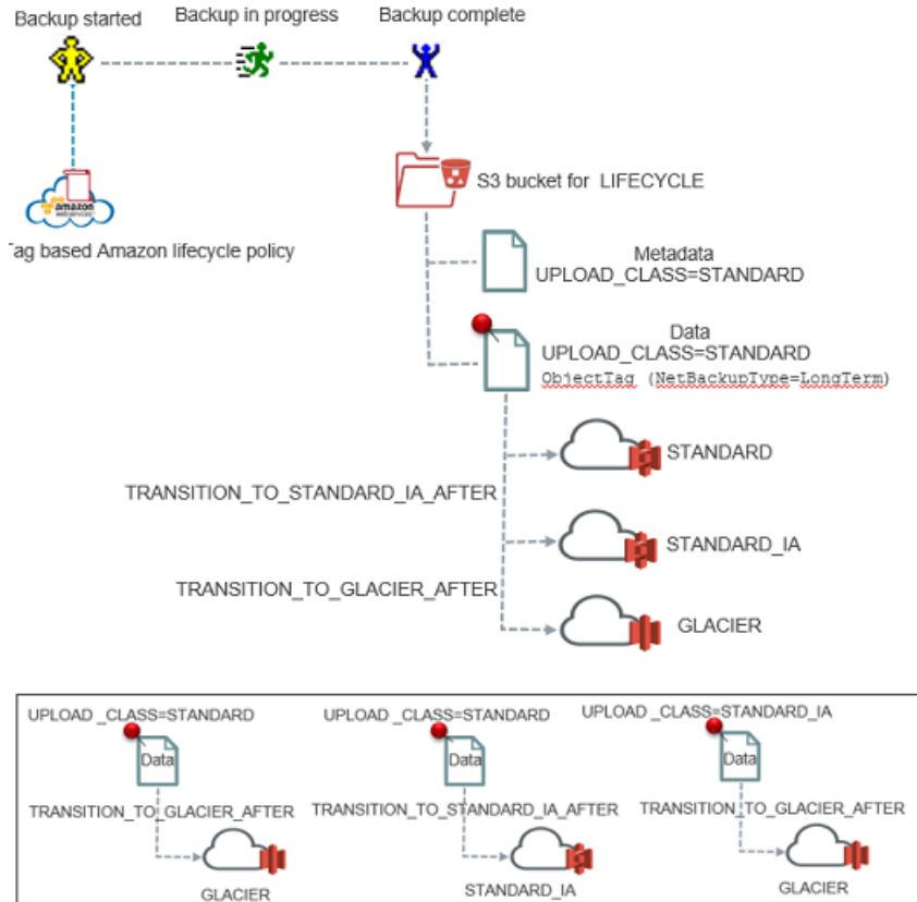
図 2-9 指定可能な構成の Amazon S3 Intelligent Tiering (LIFECYCLE) ストレージクラスのバックアッププロセス
