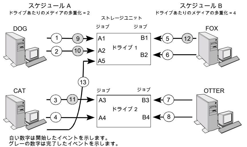
図 21-13 多重化処理のシナリオ
