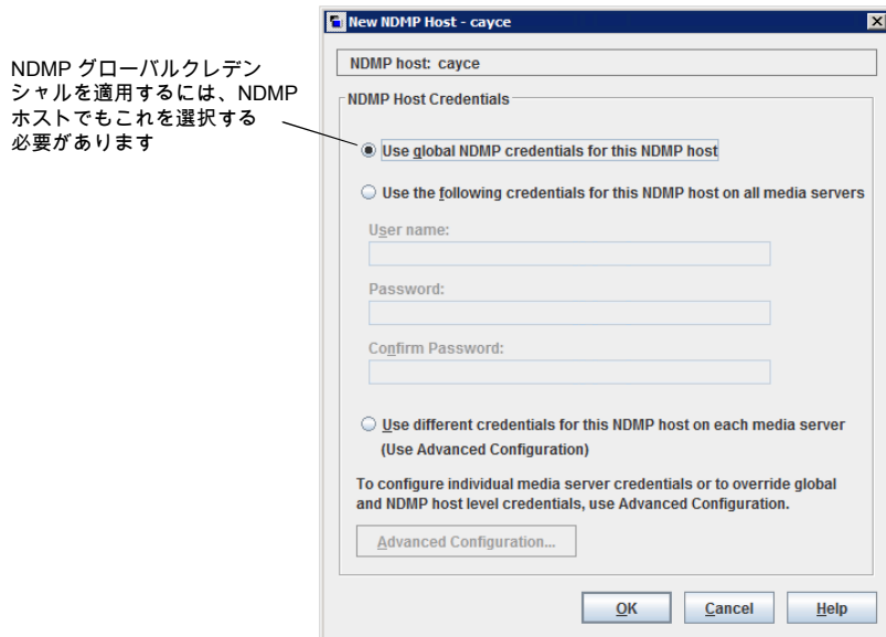
図 3-32 [NDMP ホストの追加 (Add NDMP Host)]ダイアログボックス
