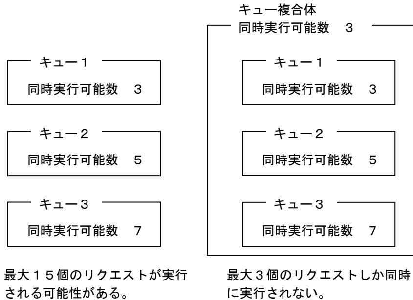
図 5-4 キュー複合体の利用イメージ
