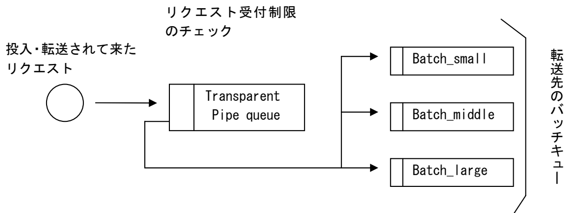
図 5-5 透過型パイプキューの処理
