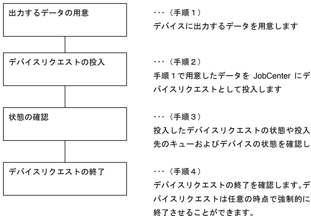
図 3-2 バッチリクエストの操作手順
