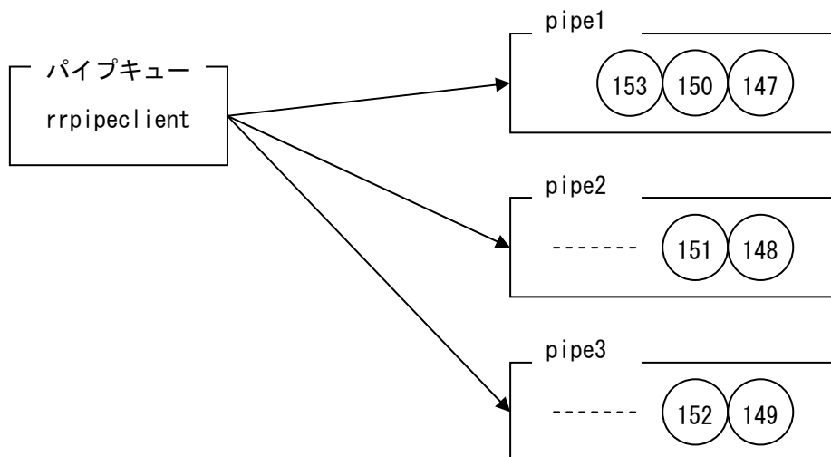
図 6-5 ラウンドロビン方式のリクエスト転送イメージ
