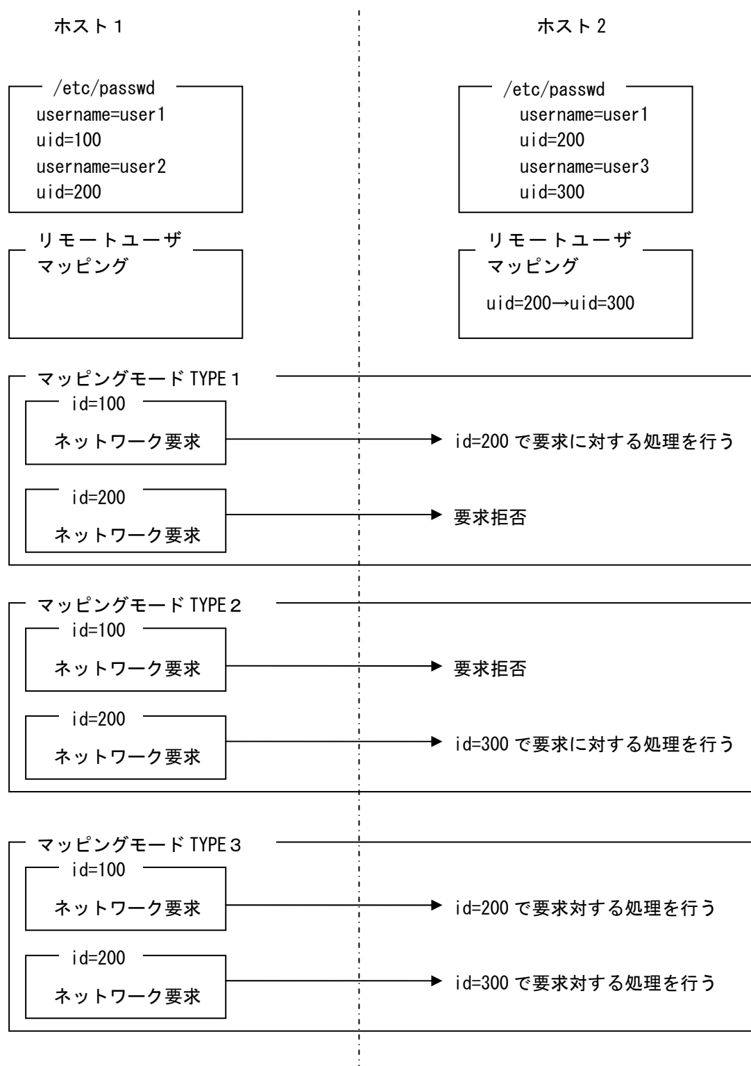
図 6-4 マッピングモードとユーザマッピングの例
