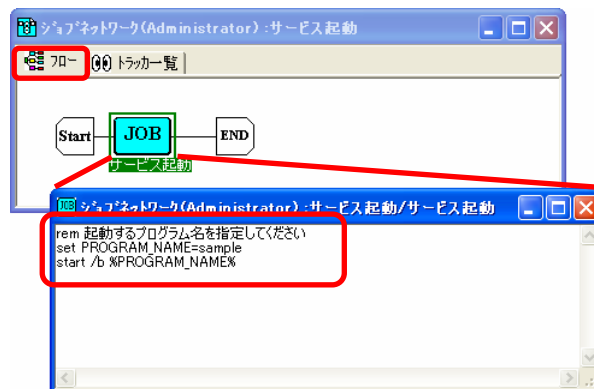
図 4-5 単位ジョブのバッチファイル（Windows）の例
