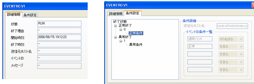
図 4-63 トラック上のイベント受信部品をダブルクリックした時の表示例
