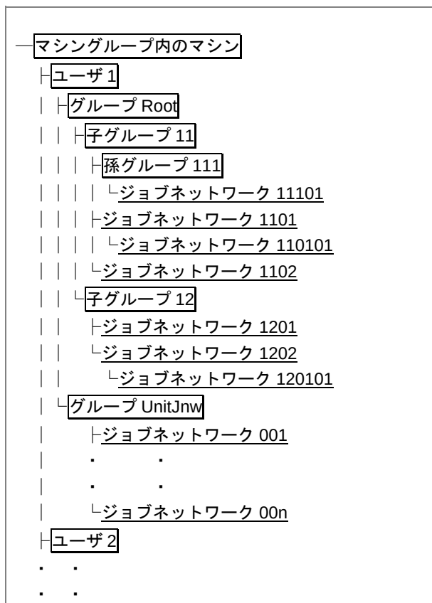
図 5-15 ツリー表示の階層イメージ
