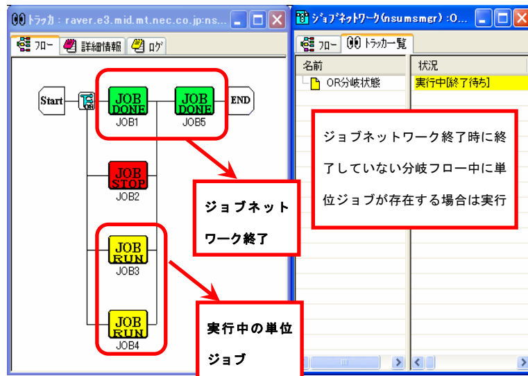
図 4-41 ジョブネットワーク終了時に実行中の単位ジョブがある場合のトラッカ状態例
