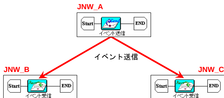
図 4-50 スター型連携モデル例
