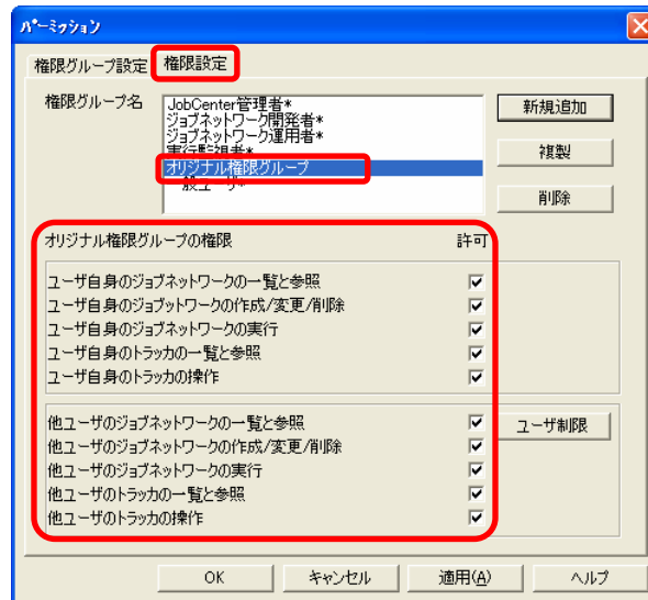
図 9-8 選択した権限グループに許可する権限を選択画面例
