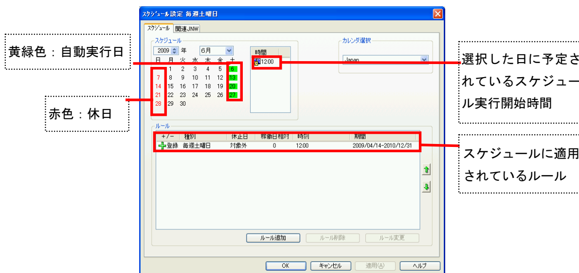
図 3-24 「スケジュール設定」画面例
