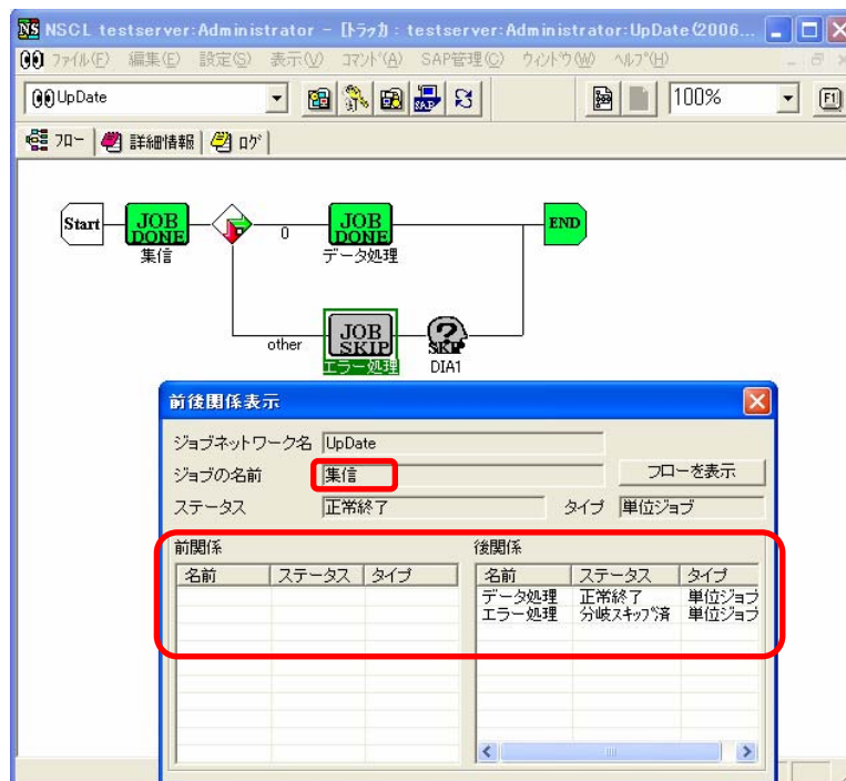
図 5-66 前関係の「集信」をダブルクリックしたときの結果表示例
