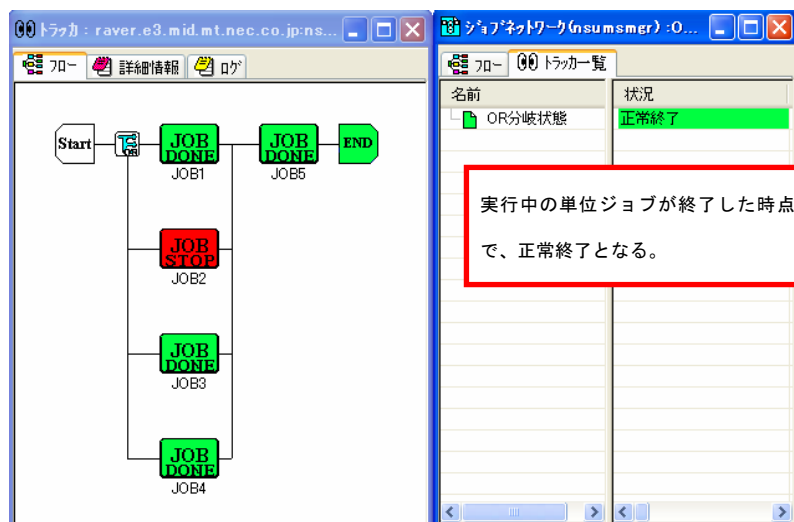
図 4-42 すべての単位ジョブが終了した場合のトラッカ状態例
