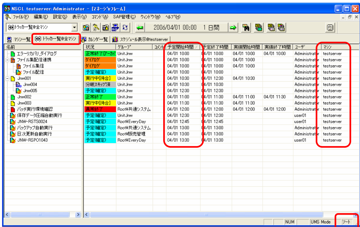
図 5-22 ソート表示（マネージャフレームのトラッカー一覧@全マシン）画面例
