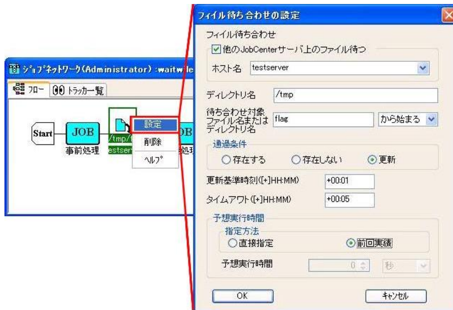
図 4-47 ファイル待ち合わせ設定画面例
