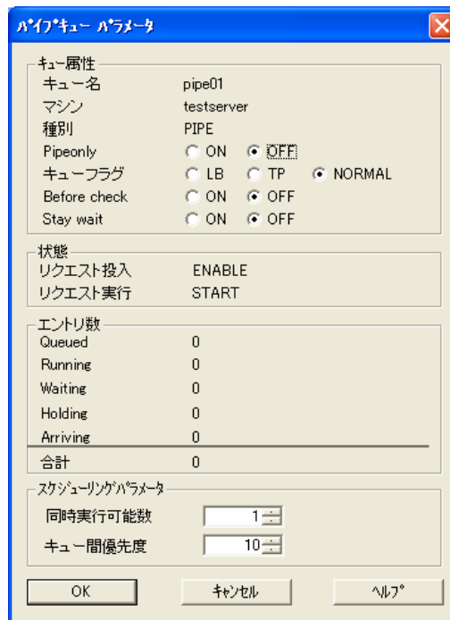
図 6-15 パイプキューパラメータの設定画面例
