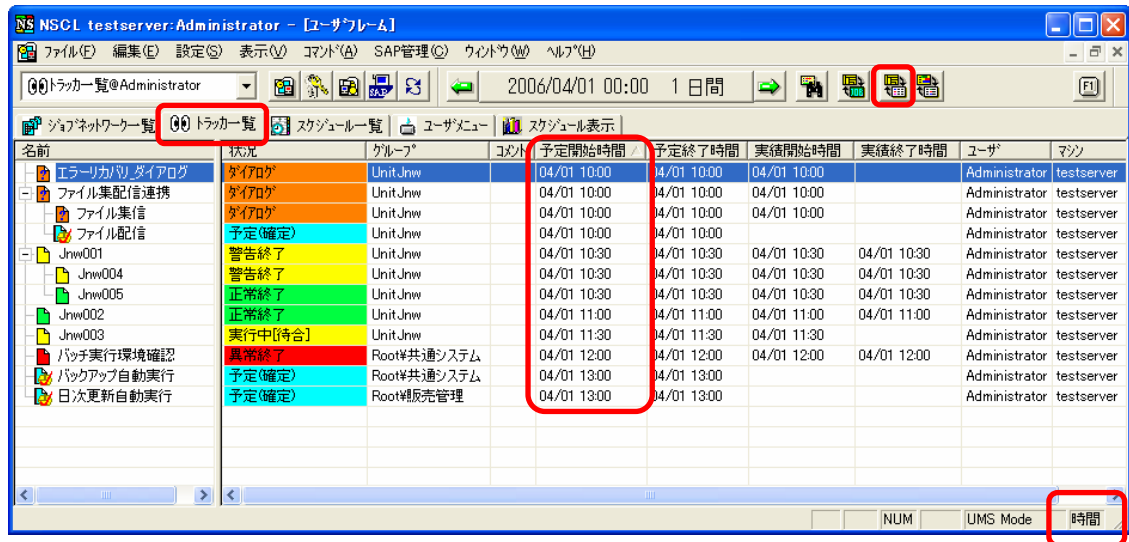
図 5-20 時間表示（ユーザフレームのトラッカー一覧）画面例
