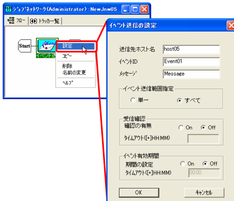
図 4-52 イベント送信の設定画面例
