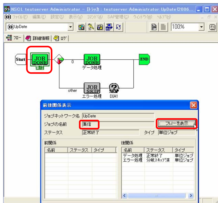
図 5-68 [フローを表示] ボタンをクリックしたときのフォーカスの移動結果例
