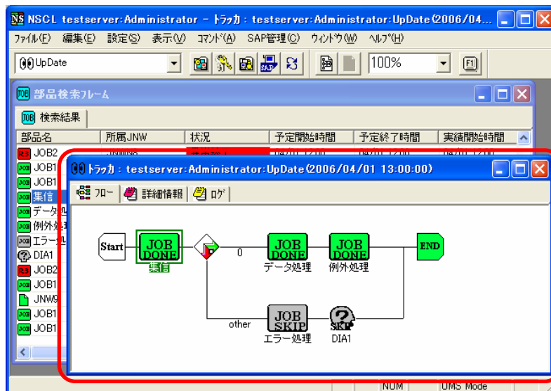
図 5-61 [ジョブネットワークトラッカ] ウィンドウ画面例
