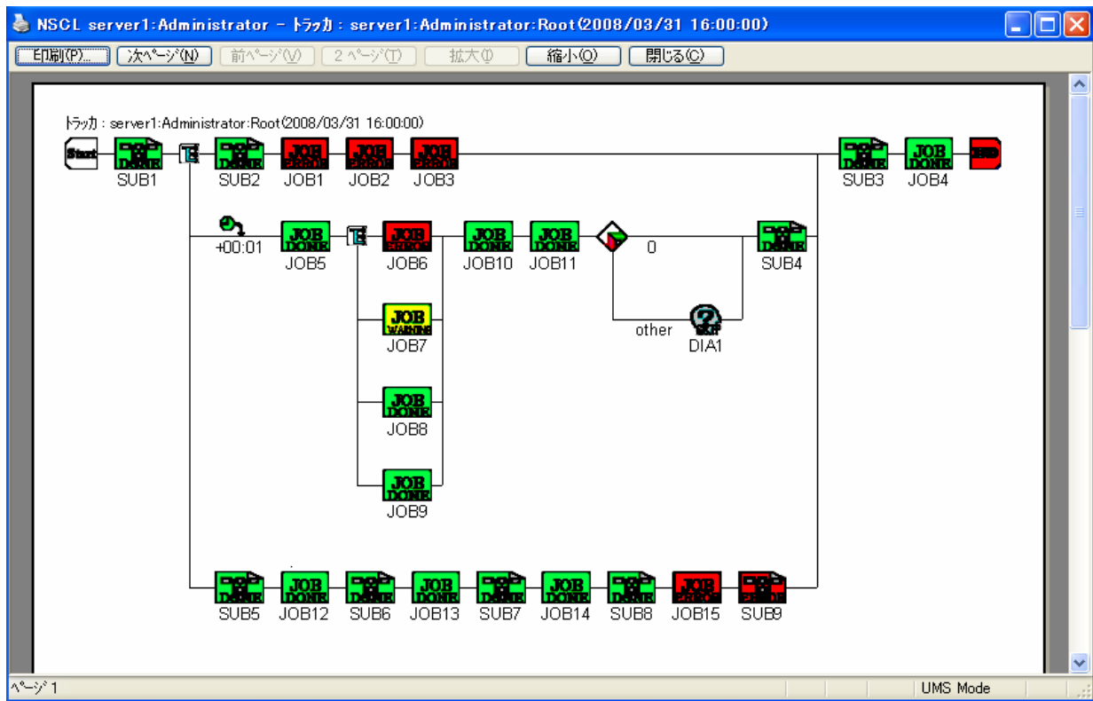
図 5-51 トラッカフロー印刷のプレビュー画面
