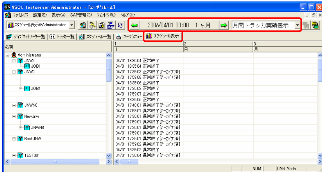
図 5-78 月間トラッカ実績表示画面例
