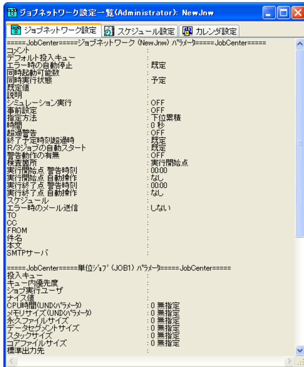
図 3-51 設定一覧画面例
