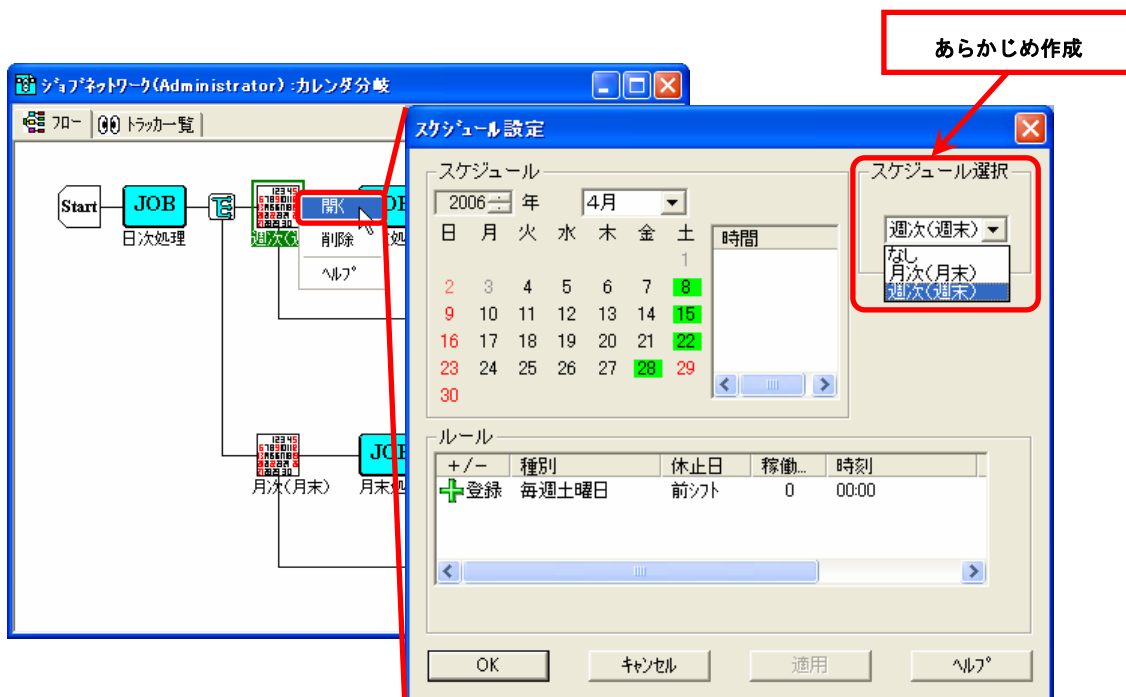
図 4-33 スケジュール設定画面例
