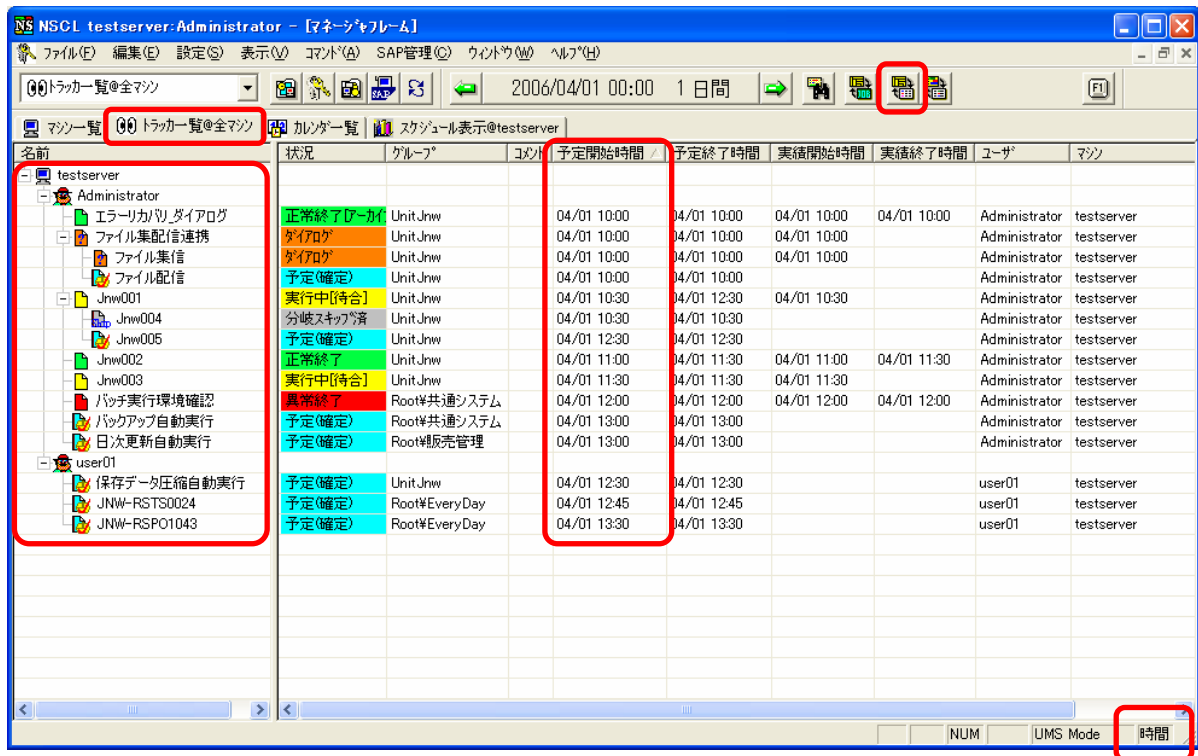
図 5-21 時間表示（マネージャフレームのトラッカー一覧@全マシン）画面例
