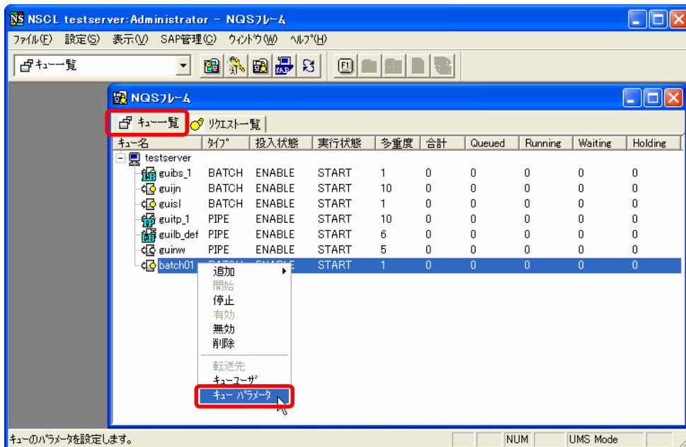
図 6-10 バッチキューの「キューパラメータ」選択画面例
