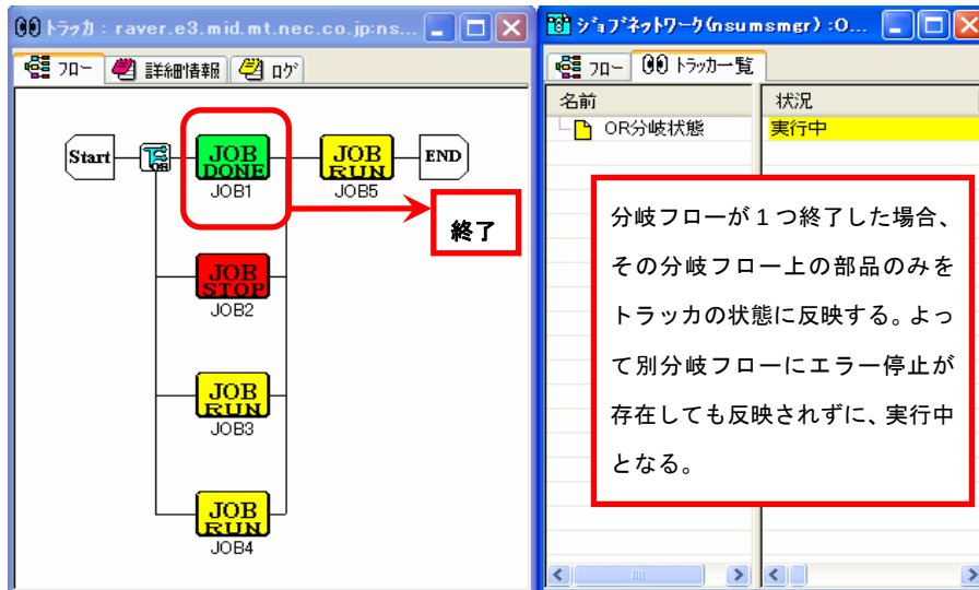
図 4-39 OR 分岐が 1 つ終了した場合のトラック状態例
