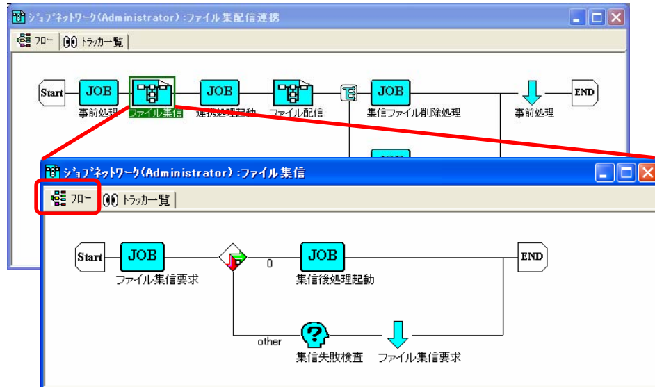
図 4-23 サブジョブネットワークの参照例
