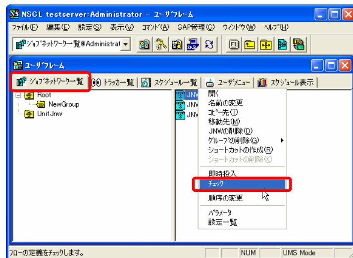
図 3-16 [チェック] 選択画面例
