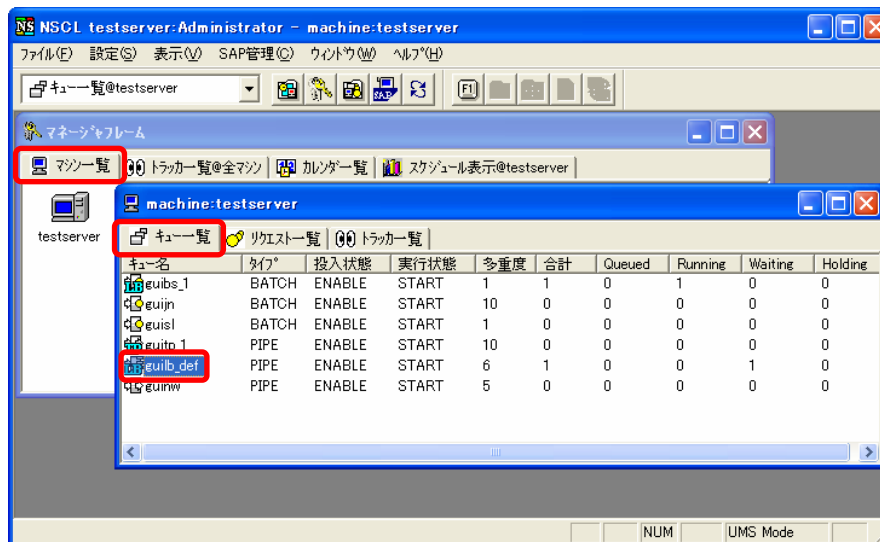
図 7-6 参照したいキューの選択（マネージャフレーム）画面例
