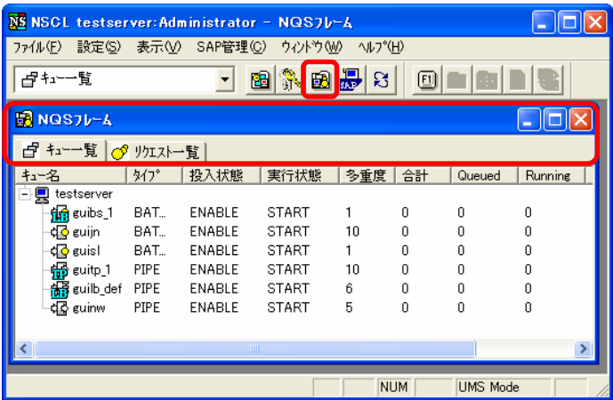
図 2-14 NQS フレーム画面例
