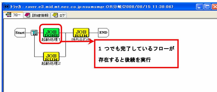
図 4-36 OR 分岐の動作例
