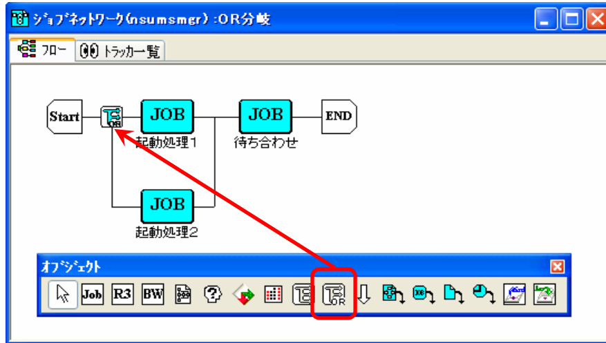
図 4-35 OR 分岐オブジェクト配置例
