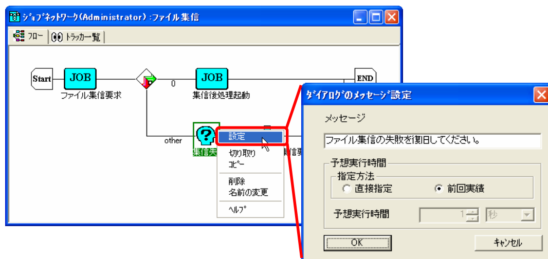
図 4-43 ダイアログオブジェクトの設定画面例
