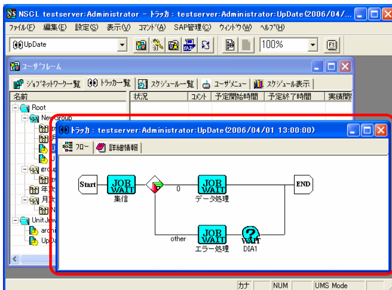
図 5-46 部品追加を行うトラッカのフロー画面例
