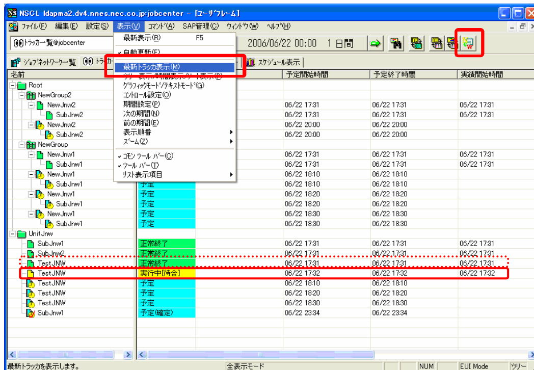
図 5-11 最新トラック表示モード実行開始画面例
