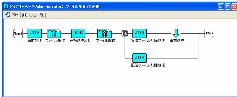
図 5-50 「ジョブネットワーク」ウィンドウの「フロー」画面例
