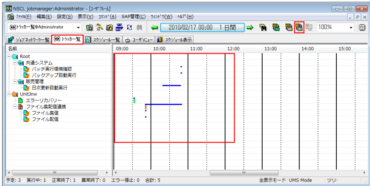
図7.6 ユーザフレームのトラッカー一覧（グラフィックモード）画面例
