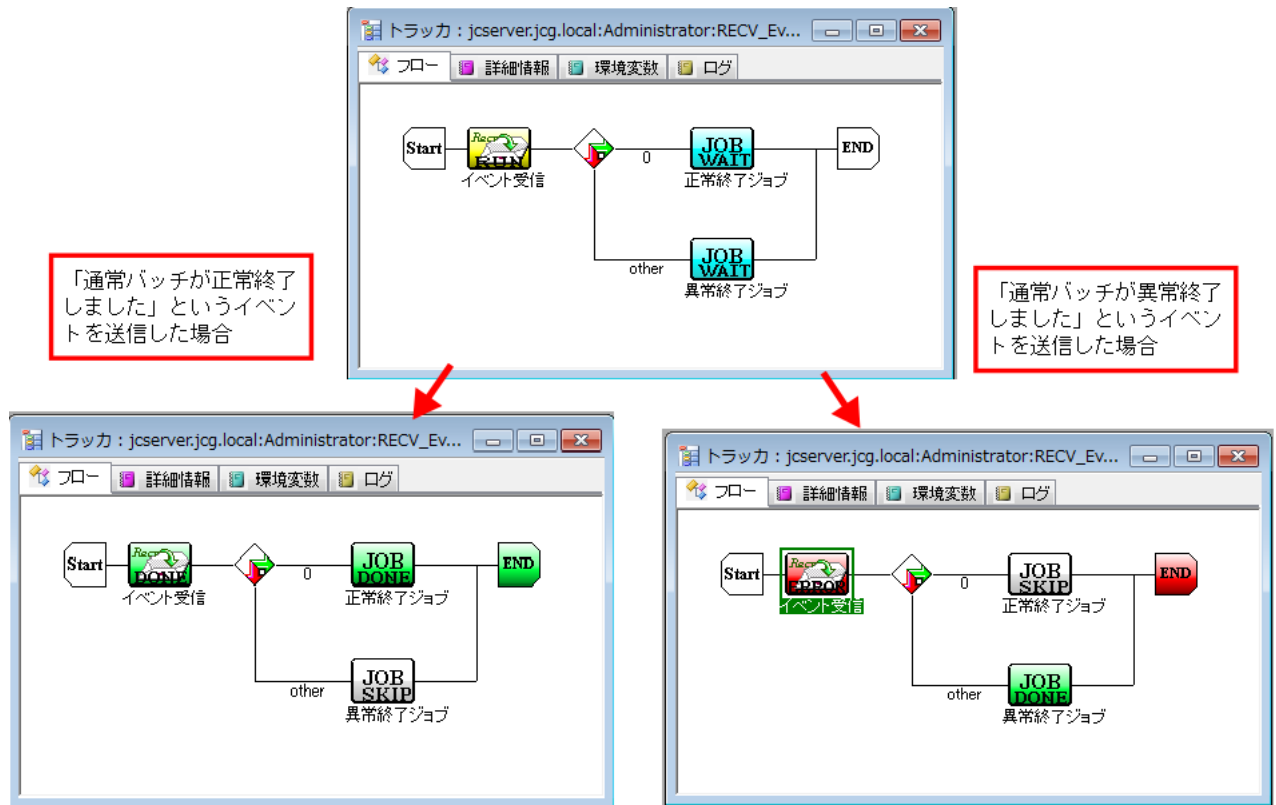
図4.65 条件成立時の動作例
