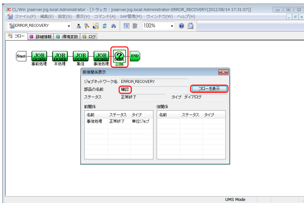
図7.80 [フローを表示] ボタンをクリックしたときのフォーカスの移動結果例
