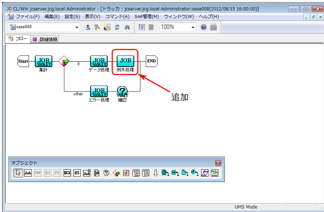
図7.57 部品オブジェクト追加画面例
