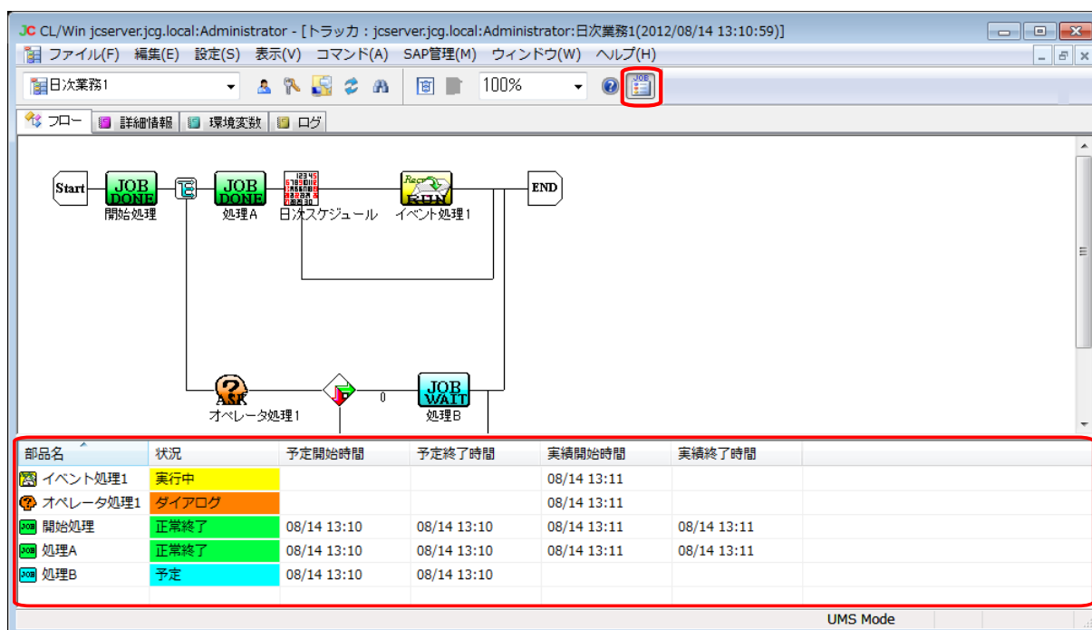
図7.42 ジョブ一覧画面の表示例
