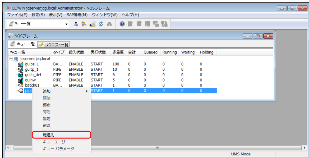
図9.19 転送先キューの指定画面例
