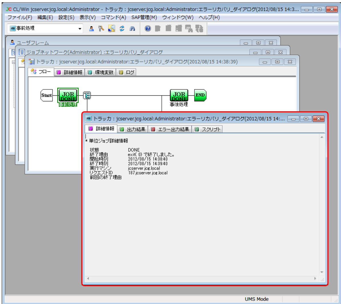
図7.65 「単位ジョブトラッカ」ウィンドウ画面例
