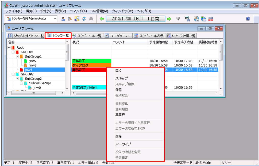
図14.3 トラッカを直接操作した画面例
