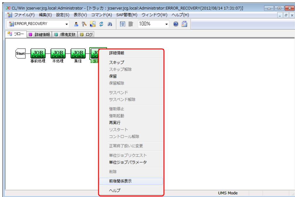
図7.76 単位ジョブトラッカアイコン操作画面例（前後関係表示）
