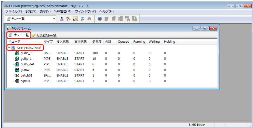
図10.3 [NQSフレーム] – [キュー一覧] 画面例
