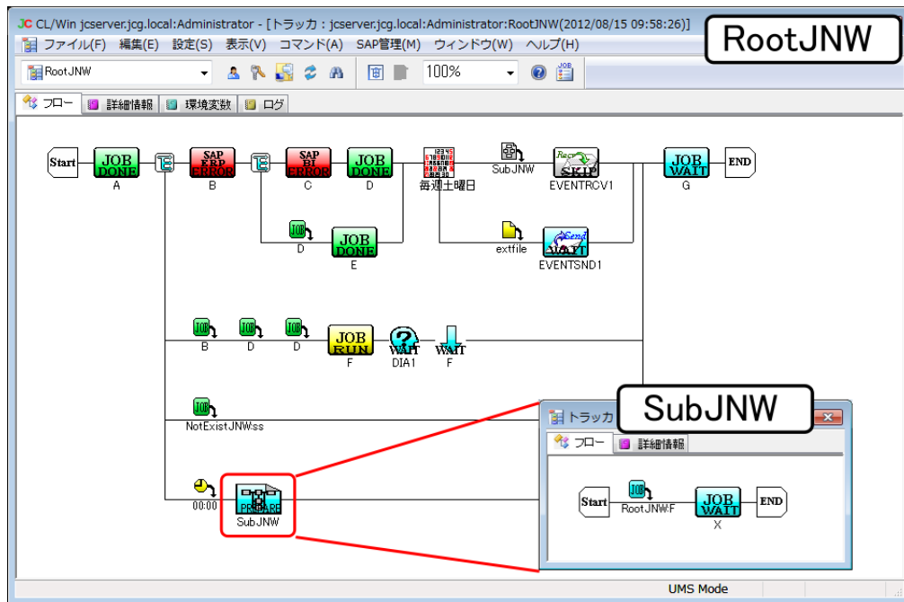
図7.81 サブジョブネットワークを含むジョブネットワークの前後関係のフロー例
