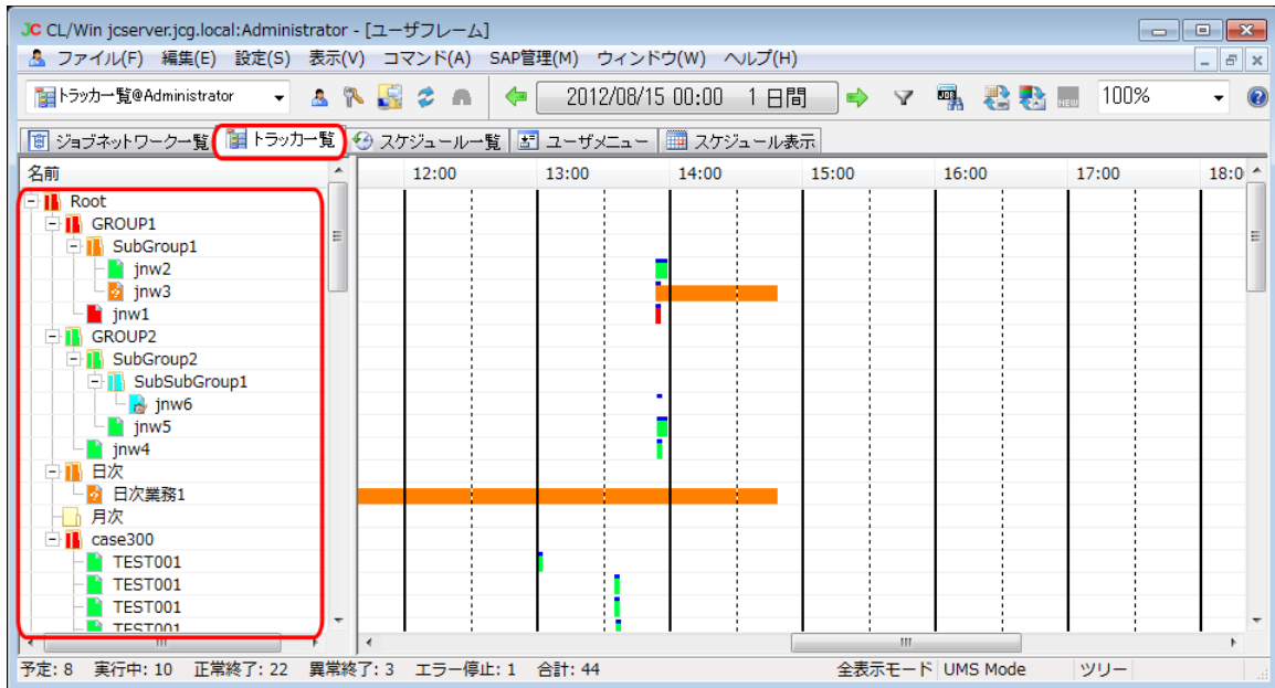
図7.16 ユーザフレームのトラッカー一覧のツリー表示画面例
