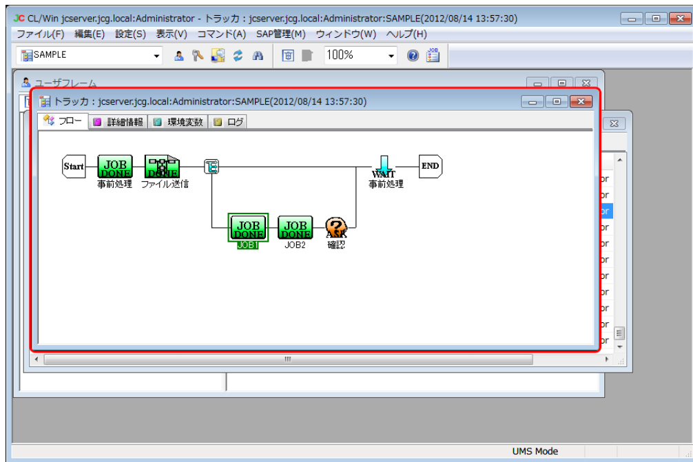
図7.73 [ジョブネットワークトラッカ] ウィンドウ画面例
