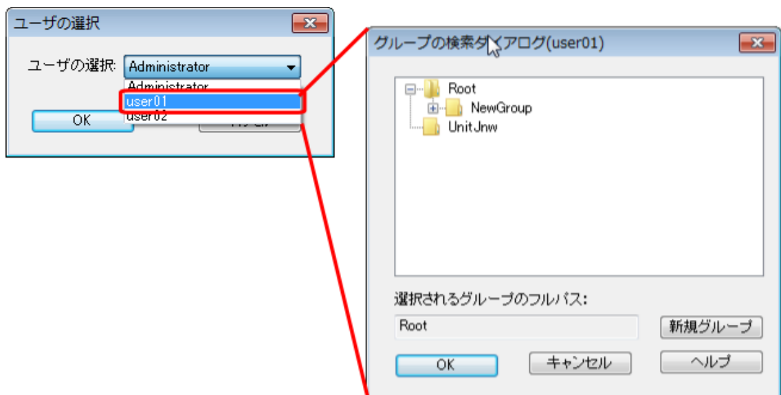
図3.31 ジョブネットワークおよびグループのコピー先指定例
