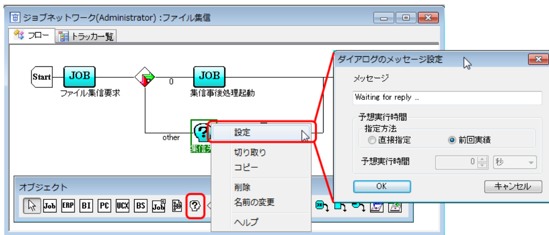
図4.43 ダイアログオブジェクトの設定画面例
