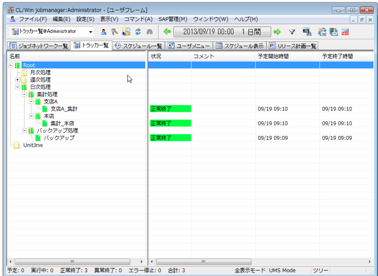
図7.19 トラッカの存在するグループのみ展開した画面例
