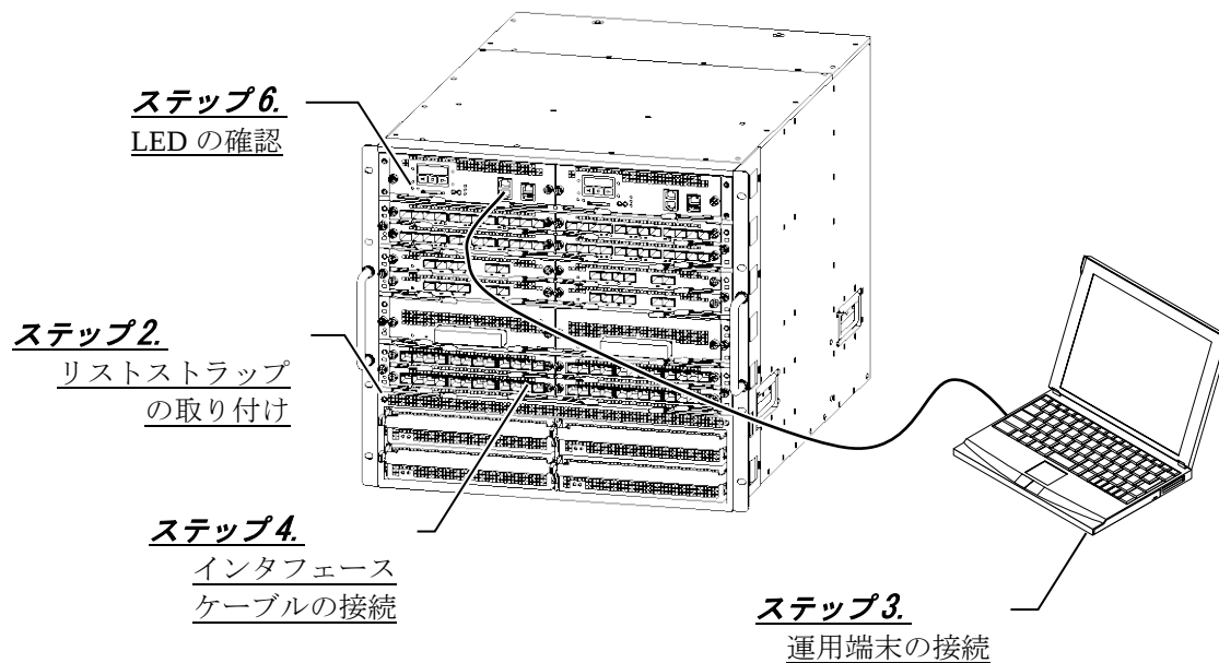
図2-7 IP8800/S8616（正面）概略図
