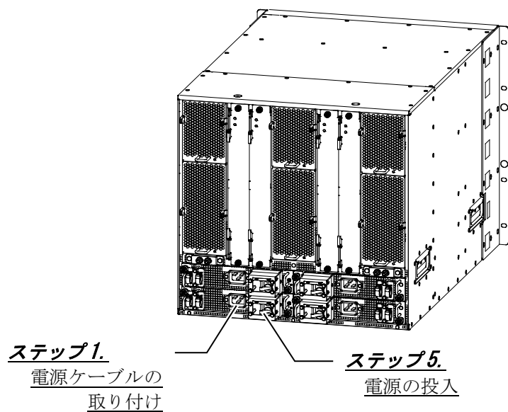
図2-6 IP8800/S8616（背面）概略図
