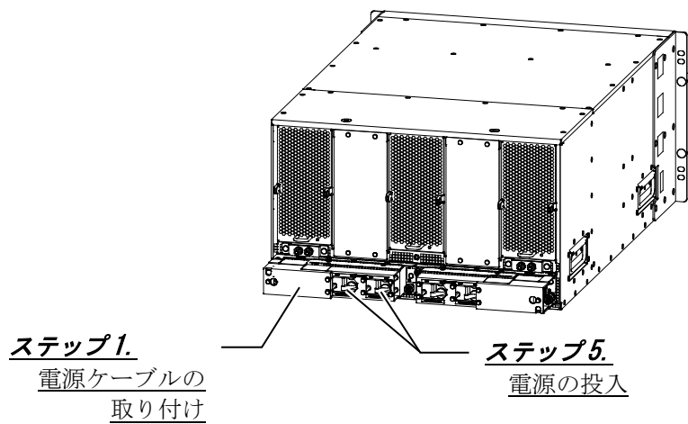
図2-4 IP8800/S8608（背面）概略図
