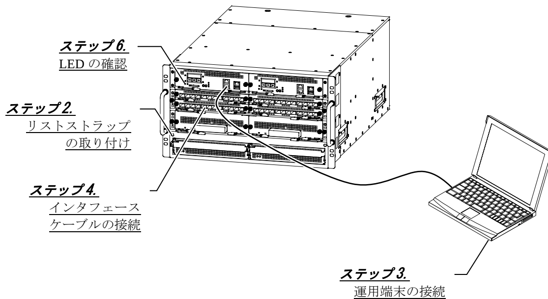
図2-4 IP8800/S8608（背面）概略図
