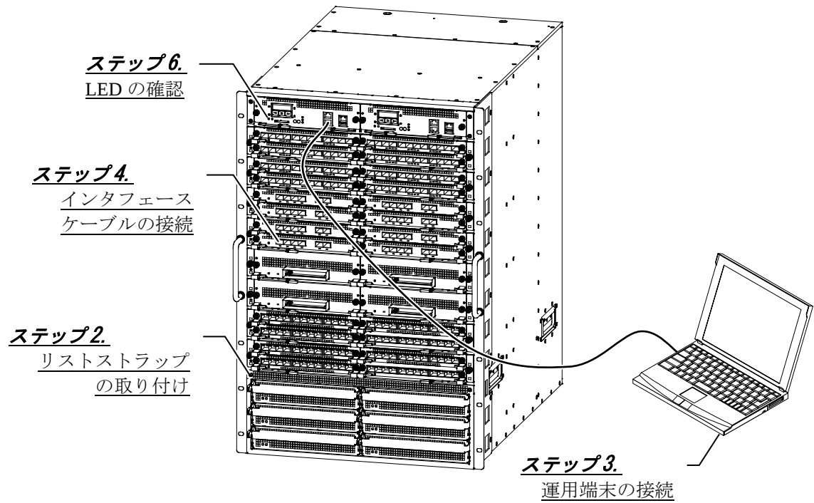
図2-10 IP8800/S8632（背面）概略図
