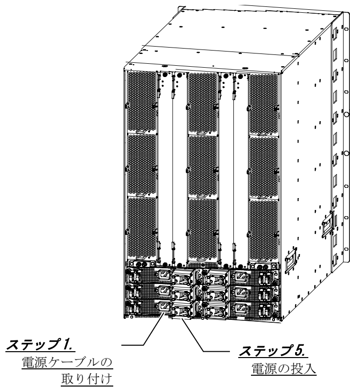
図2-10 IP8800/S8632（背面）概略図
