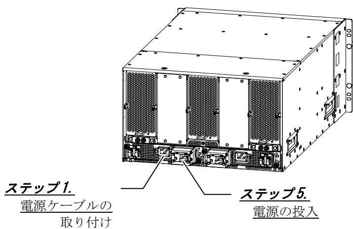
図2-2 IP8800/S8608（背面）概略図
