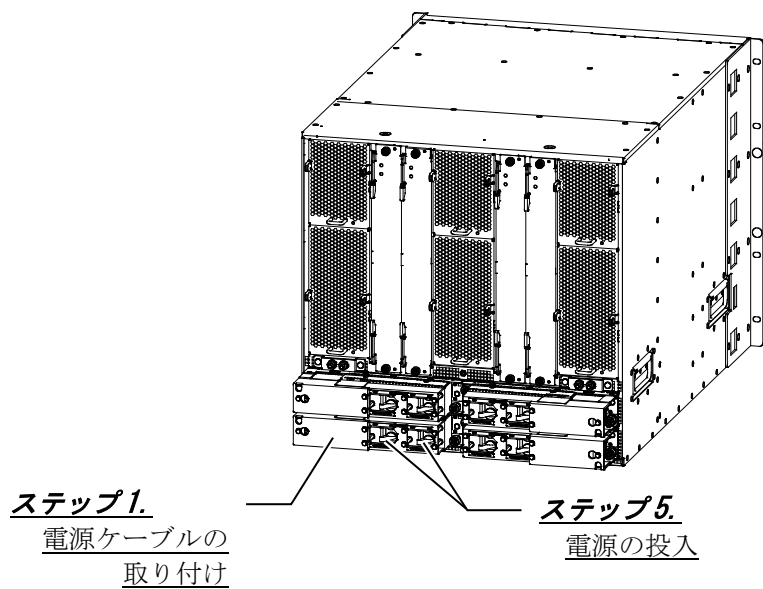
図2-8 IP8800/S8616（背面）概略図
