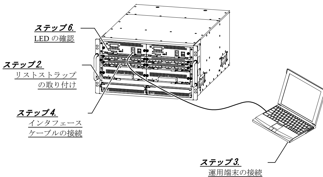
図2-1 IP8800/S8608（正面）概略図
