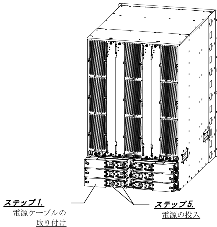
図2-12 IP8800/S8632 (背面) 概略図
