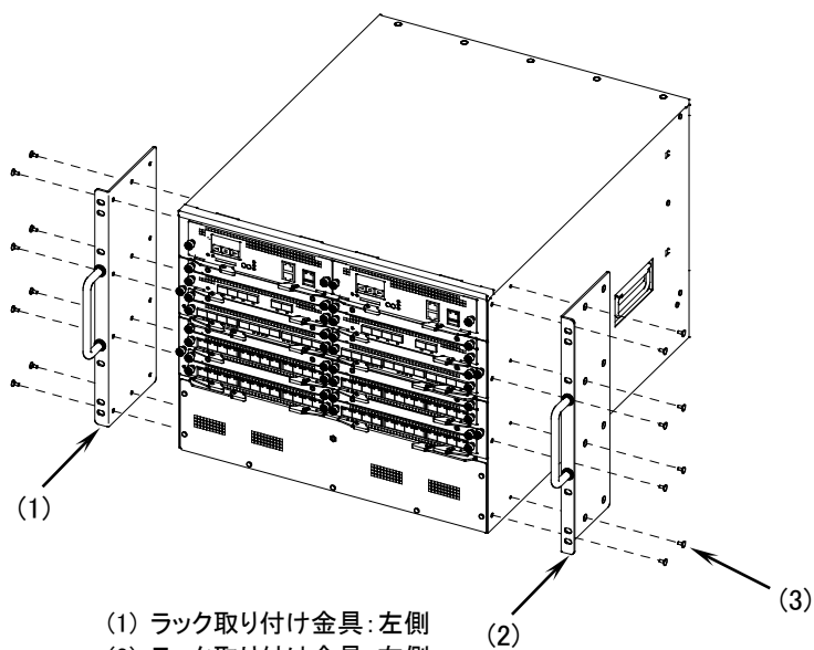
図4-3 ラック取り付け金具の取り外し
