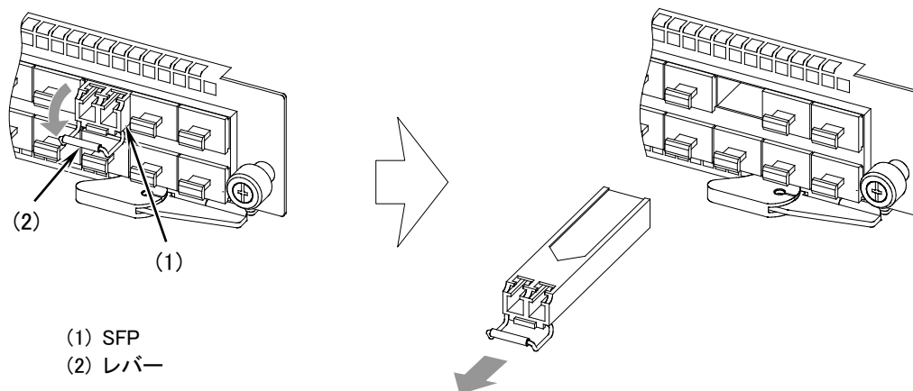
図4-33 SFP の取り外し（上側のポート）
