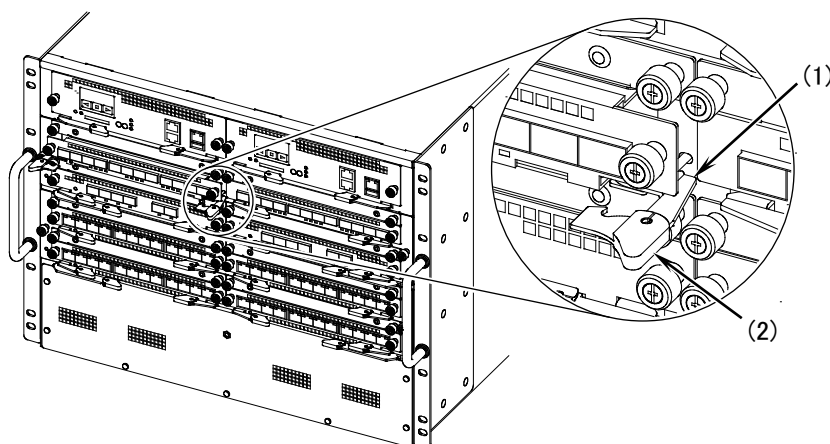
図5-39 ネットワークインタフェース機構の取り付け -2
