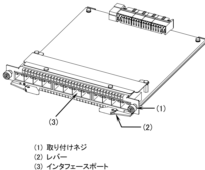
図1-28 外観
