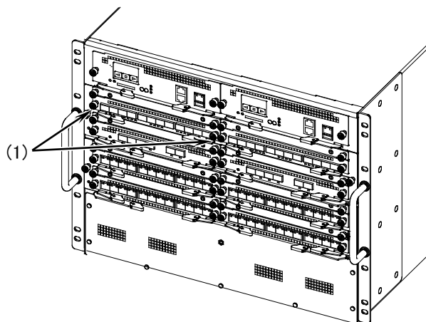
図5-41 ネットワークインタフェース機構の取り付け -4
