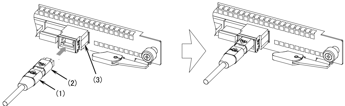
図4-48 光ファイバケーブル（MPO コネクタ）の取り付け
