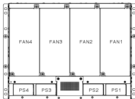
図1-8 装置背面側
