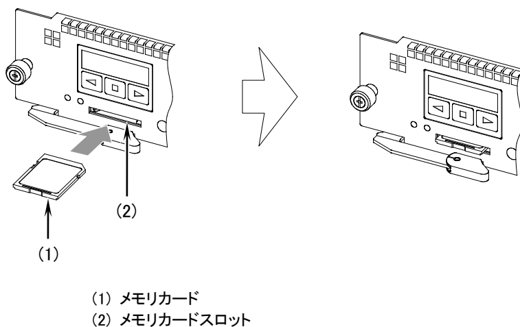
図4-27 メモリカードの取り付け
