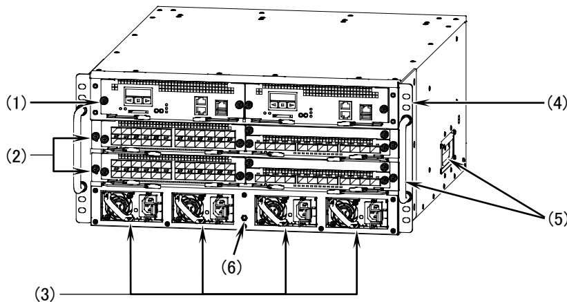
図1-1 正面外観
