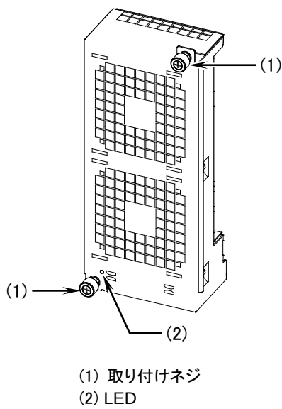
図1-10 外観
