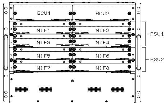
図1-7 装置正面側
