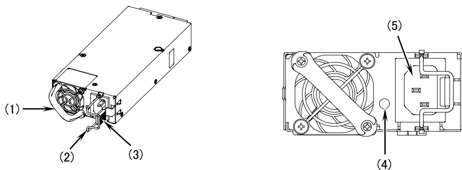
図1-11 外観および正面外観
