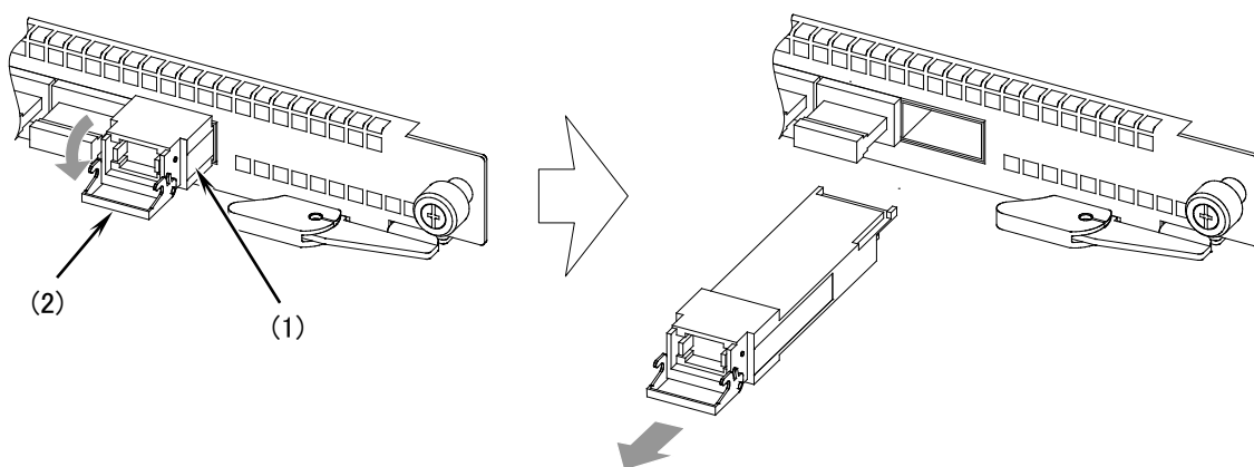
図4-37 QSFP+ の取り外し（レバータイプの場合）
