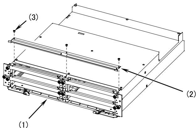
図5-27 PSU-E1A/E2A 用アダプタの取り付け
