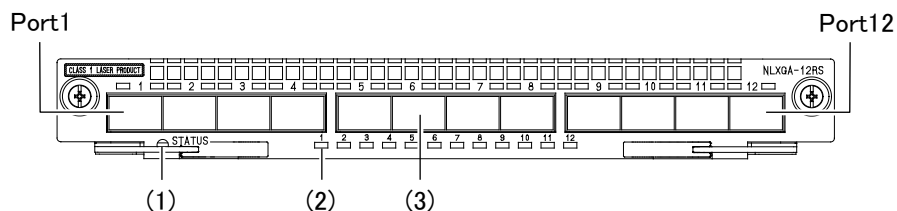
図1-39 正面外観
