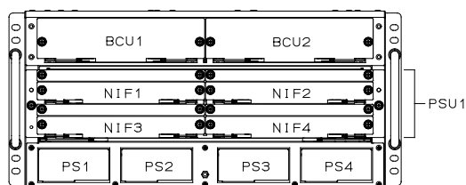
図1-4 装置背面側
