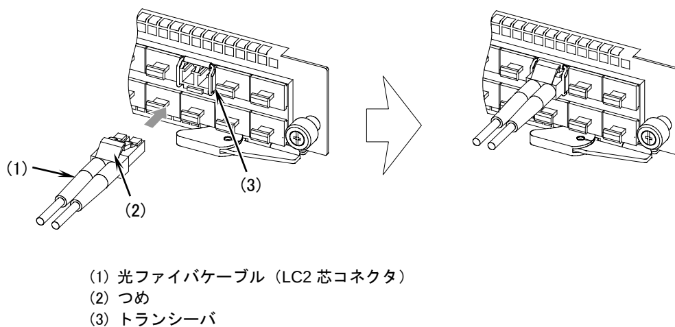
図4-44 光ファイバケーブル（LC2 芯コネクタ）の取り付け（上側のポート）
