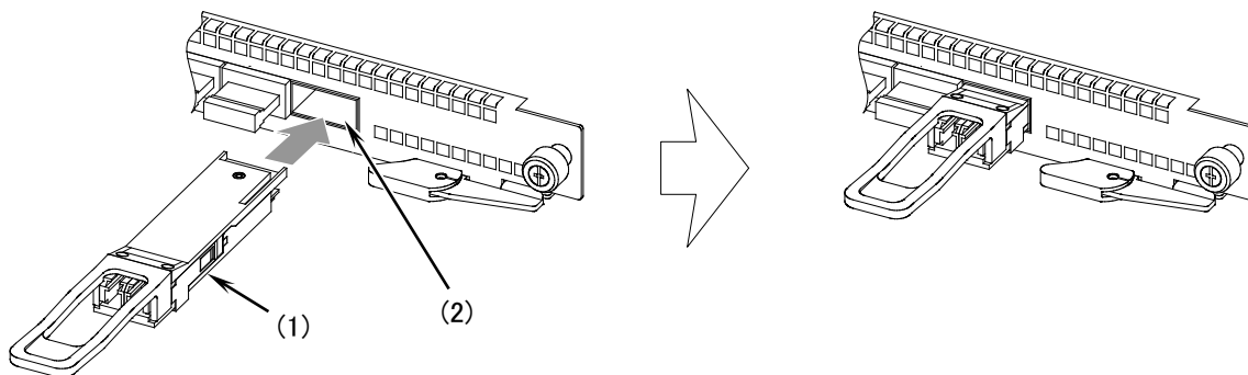
図4-36 QSFP+ の取り付け（プルタブタイプの場合）
