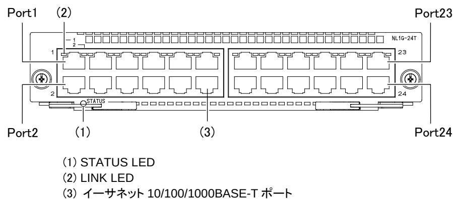
図1-34 正面外観
