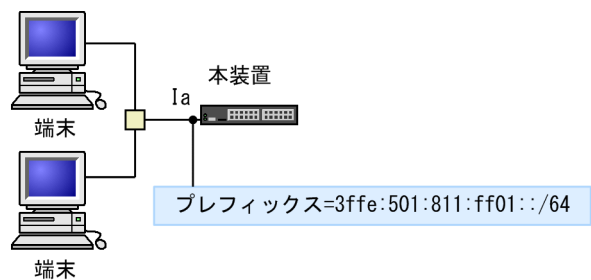
図 20-3 RA の使用例
