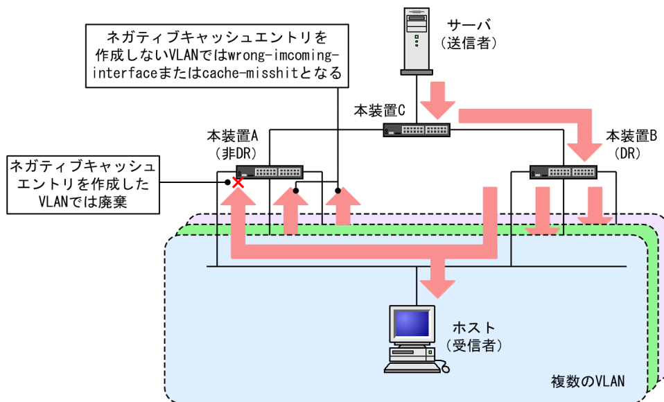
図 14-31 複数 VLAN 設定時のマルチキャストパケット廃棄処理
