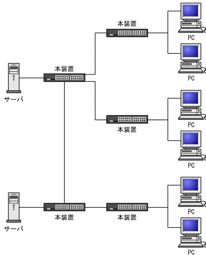
図 30-26 IPv6 PIM-SSM を使用する構成図
