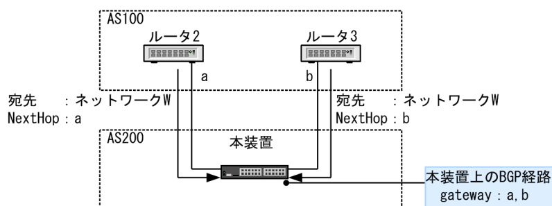
図 12-17 複数のピアから学習した BGP4 経路マルチパス化の概念
