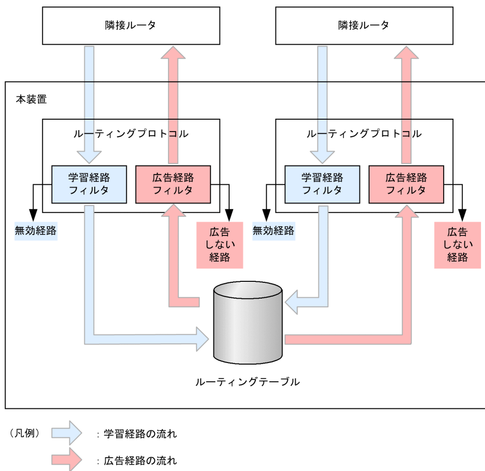
図 13-1 経路フィルタリングの概念図
