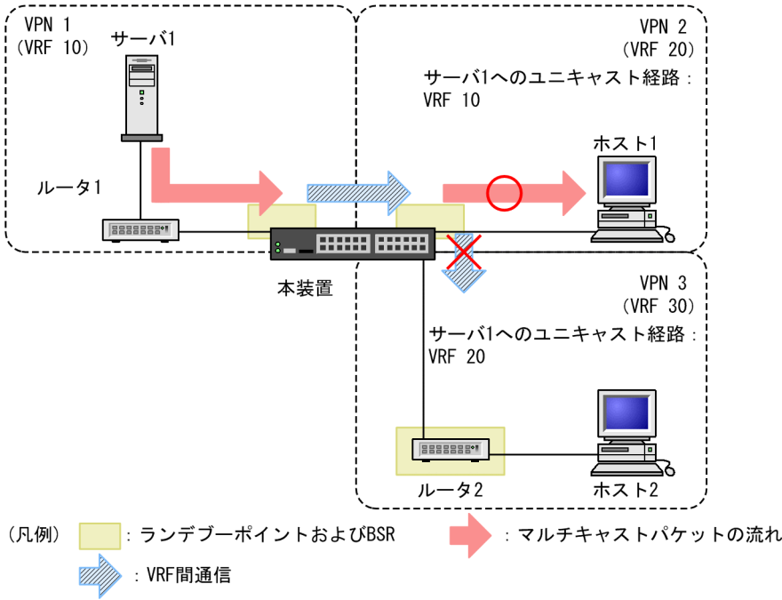
図 30-23 IPv6 マルチキャストエクストラネット使用時に装置内で VRF 中継を禁止している例
