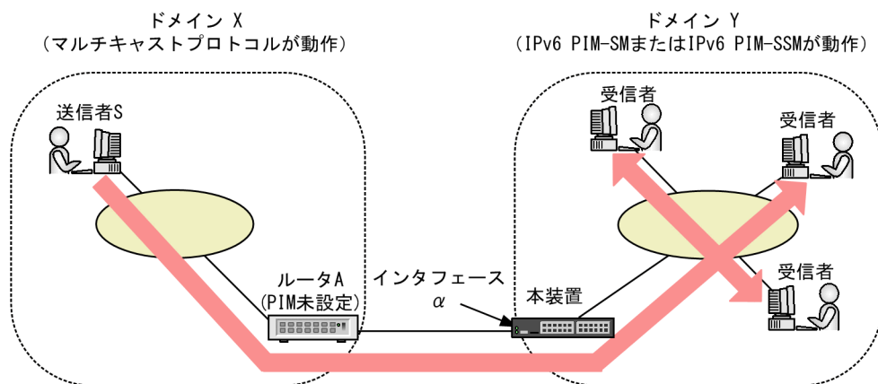
図 30-27 コンフィグレーションコマンド ipv6 pim direct を設定する場合の適応例
