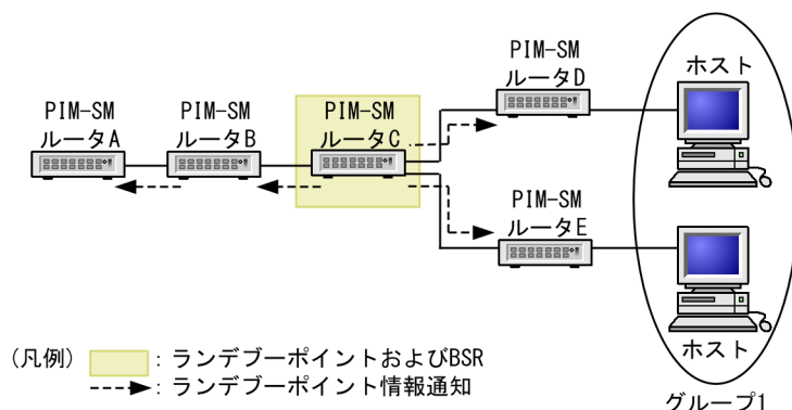
図 30-7 ランデブーポイントおよびブートストラップルータ (BSR)
