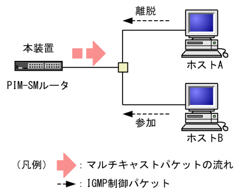
図 14-29 注意が必要な構成（ルータと複数ホストの接続）
