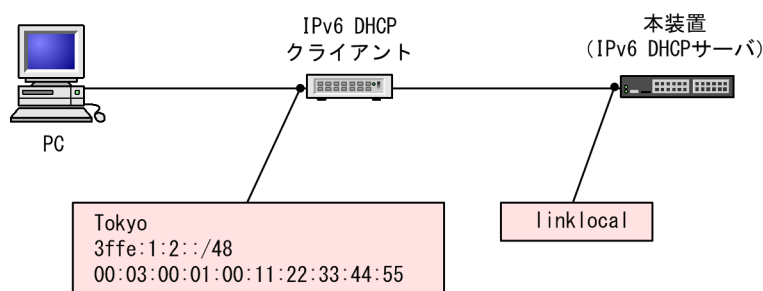
図 22-1 クライアントごとに固定プレフィックスを指定する構成
