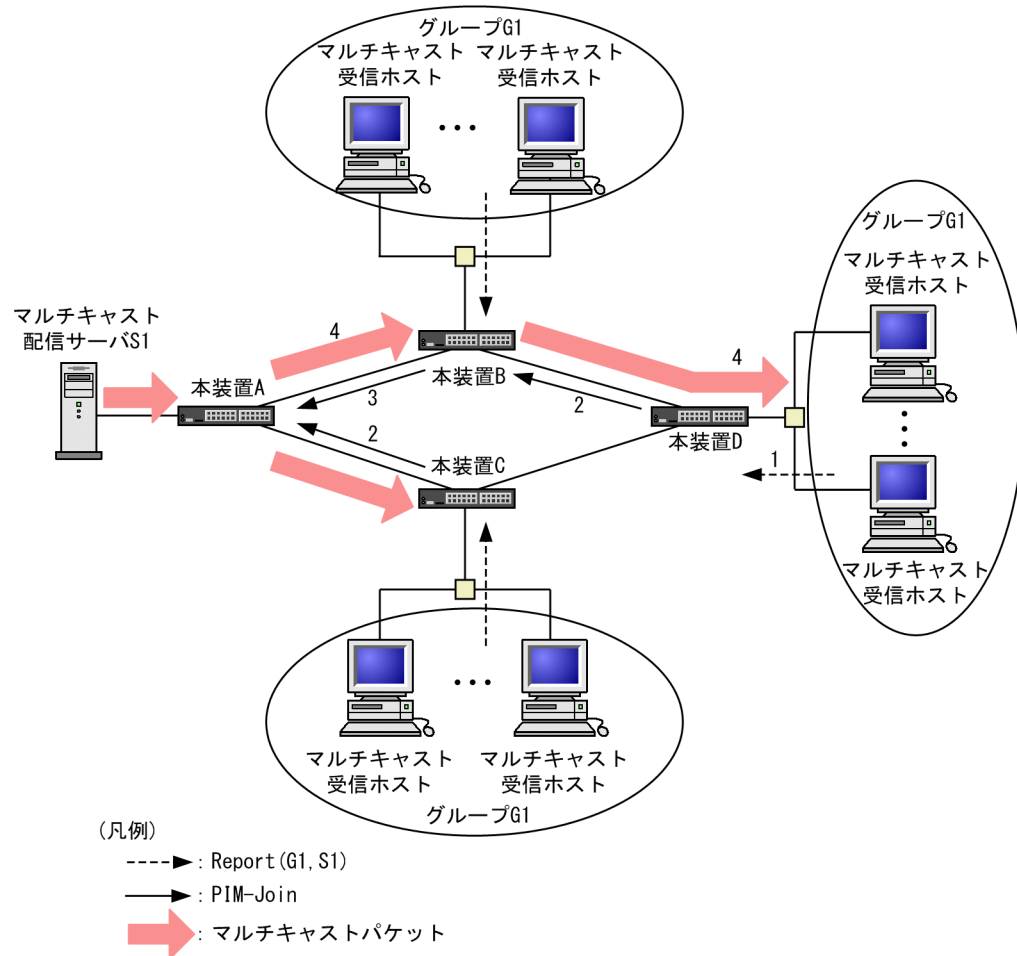
図 14-19 IGMPv3 使用時の IPv4 PIM-SSM 動作概要
