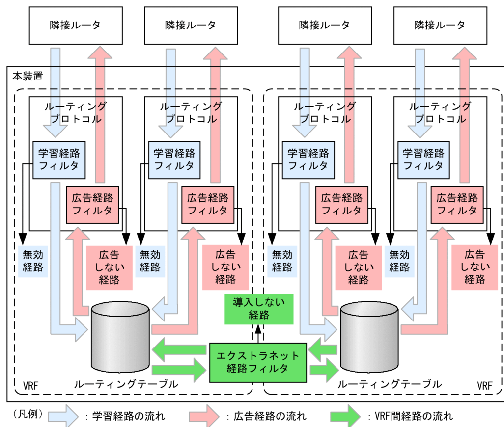
図 29-2 エクストラネットの経路フィルタリングの概念図
