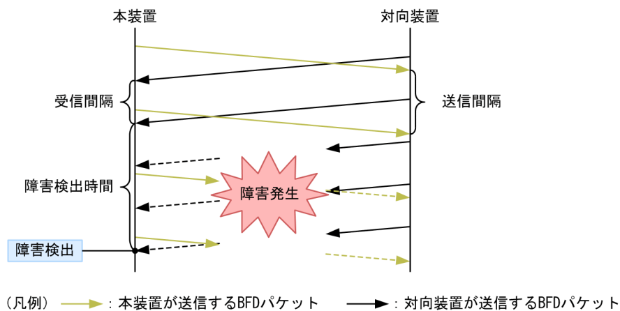
図 33-4 BFD セッションでの障害検出
