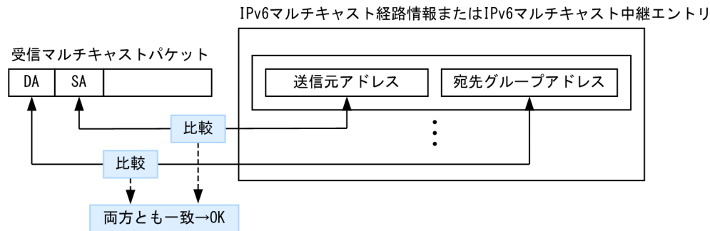
図 30-5 IPv6 マルチキャスト経路情報または IPv6 マルチキャスト中継エントリの検索方法
