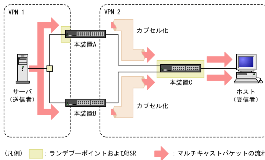
図 30-35 注意が必要な構成 (2 台以上の VRF 境界ルータで冗長構成を構築する場合)
