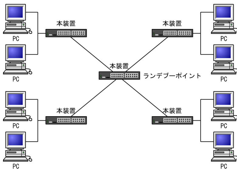
図 14-26 PIM-SM を使用する構成図
