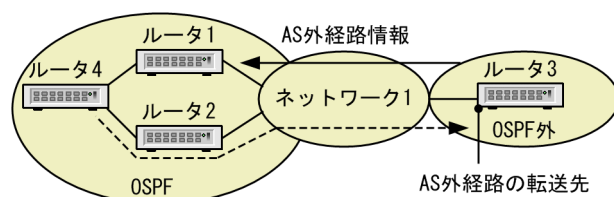
図 10-5 システム構成例（フォワーディングアドレスを目標とする場合）
