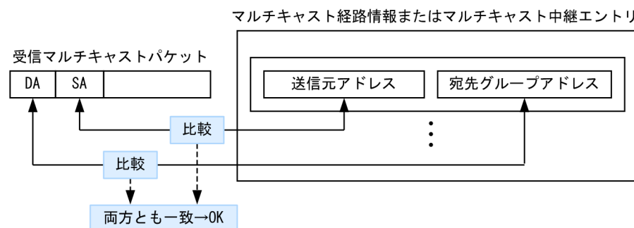
図 14-6 マルチキャスト経路情報またはマルチキャスト中継エントリの検索方法
