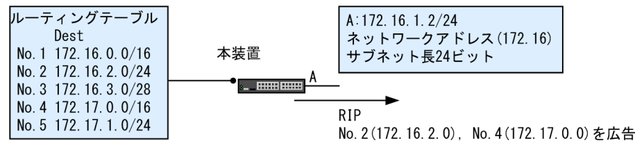
図 9-11 RIP で広告するナチュラルマスク経路およびサブネットマスク経路情報
