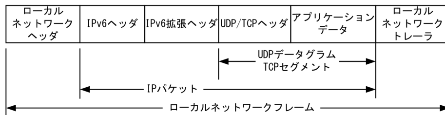
図 17-21 IPv6 パケットフォーマット
