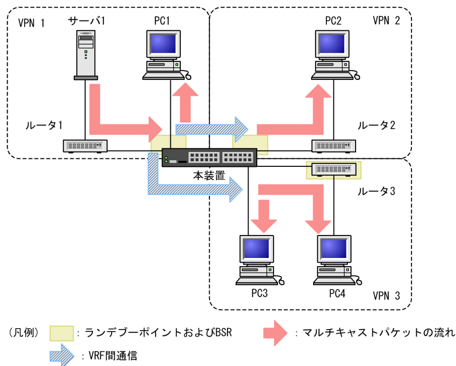
図 30-21 IPv6 マルチキャストエクストラネットの動作概要
