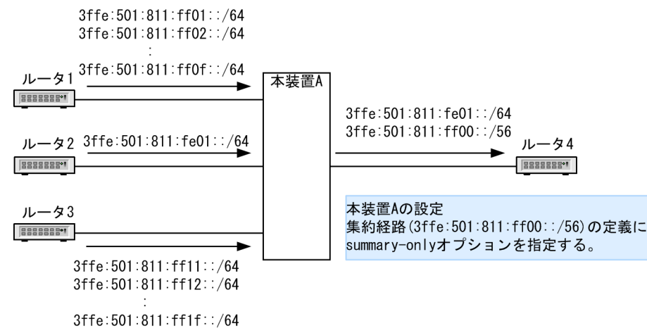
図 23-6 集約元経路の広告抑止の適用例
