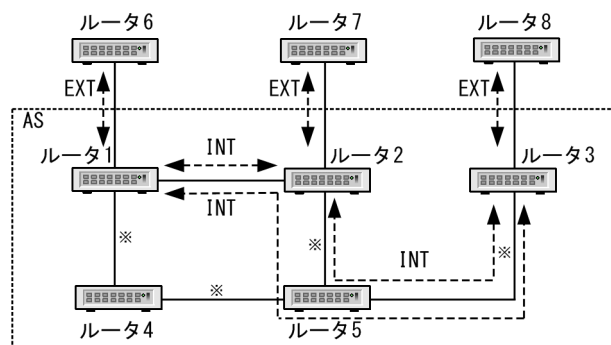
図 28-1 内部ピアと外部ピア
