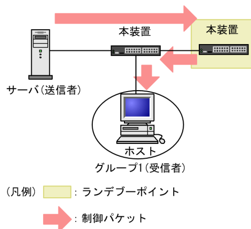
図 30-33 不適応な構成 (送信者とランデブーポイントの間に受信者が存在する場合)
