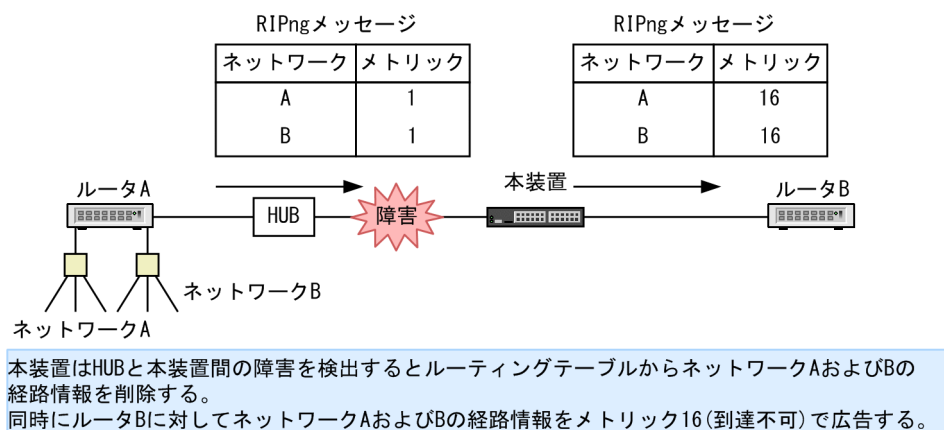
図 25-2 triggered update による経路情報の広告
