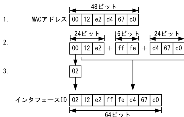
図 20-2 MAC アドレスからのインタフェース ID 生成
