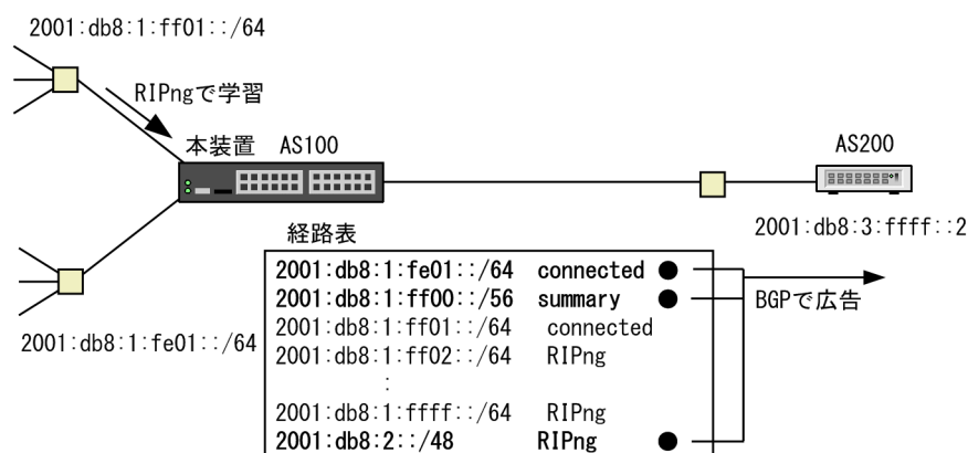
図 23-8 集約経路を BGP4+で広告する構成
