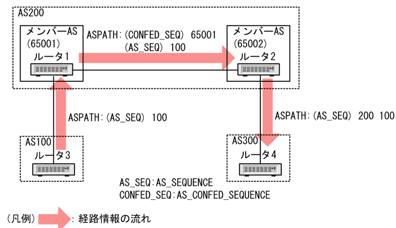
図 12-26 AS_PATH 属性の取り扱い
