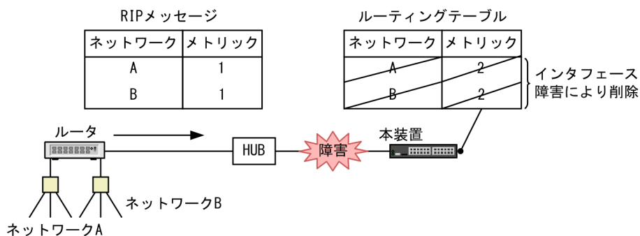
図 9-10 インタフェース障害による経路情報の削除
