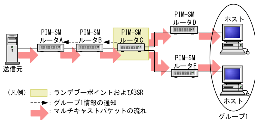
図 30-10 IPv6 マルチキャストパケット通信 (デカプセル化)
