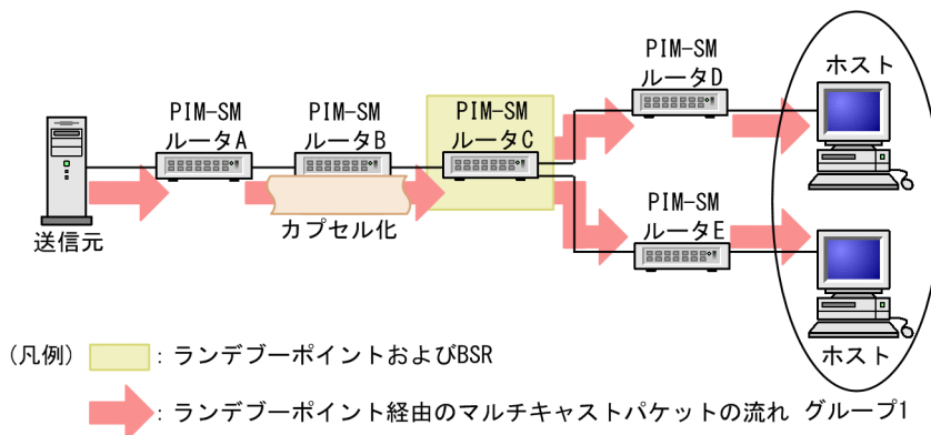
図 30-9 IPv6 マルチキャストパケット通信 (カプセル化)
