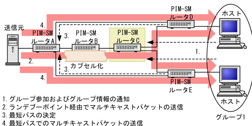
図 30-6 PIM-SM の動作概要
