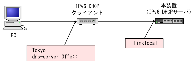
図 22-3 クライアントにオプション情報を配布する構成
