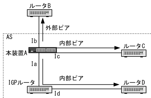
図 28-7 BGP4+ピアから学習した経路を広告する場合に通知する経路情報のネクストホップの設定例
