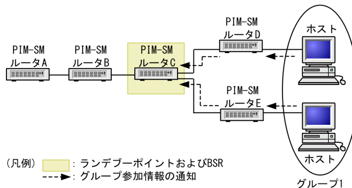
図 30-8 ランデブーポイントへのグループ参加情報の通知
