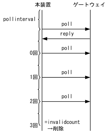
図 8-4 スタティック経路の動的監視による経路削除 (invalidcount=3 の場合)
