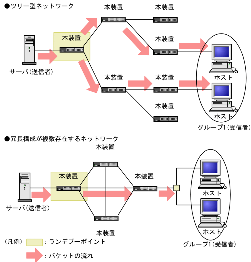
図 30-32 IPv6 PIM-SM 推奨ネットワーク構成
