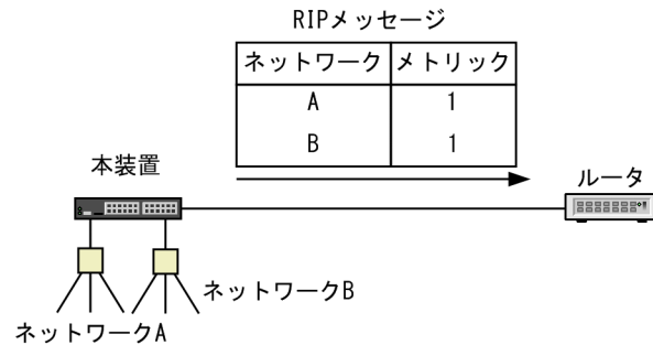
図 9-1 周期的な経路情報広告
