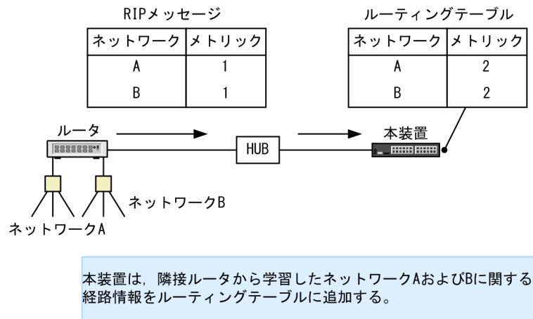
図 9-8 レスポンスパケット受信による経路情報の生成
