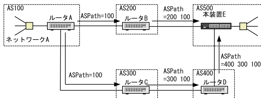
図 12-3 AS_PATH 属性による経路選択
