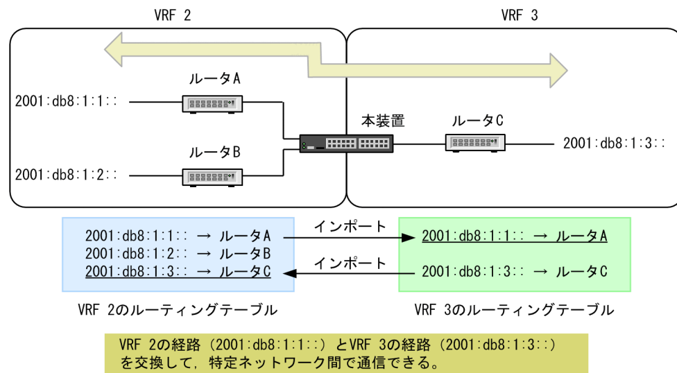
図 23-12 VRF 間の経路交換
