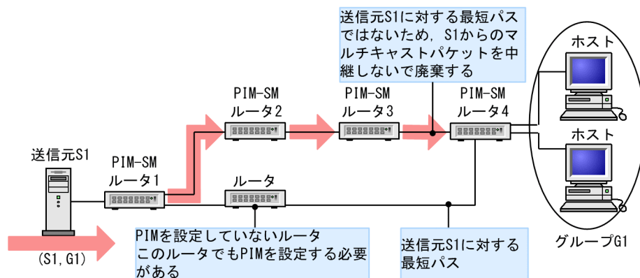
図 30-17 冗長経路時の注意事項
