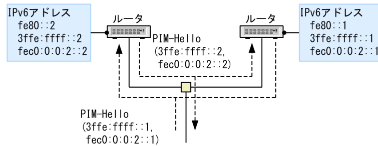
図 30-13 PIM-Hello メッセージによる隣接ルータアドレス受信
