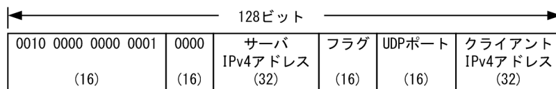
図 17-17 Teredo IPv6 アドレス
