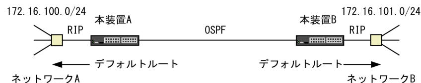
図 7-6 デフォルトルートの広告の例
