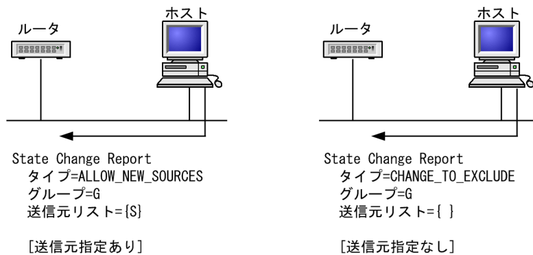
図 30-3 MLDv2 グループ参加・離脱動作
