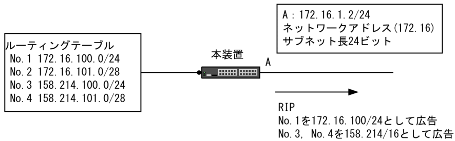
図 9-6 RIP-1 使用時の広告経路自動集約化
