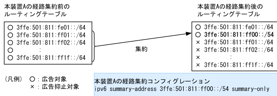
図 23-7 経路集約のコンフィグレーション例と経路集約前後の経路
