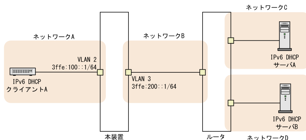
図 21-4 1 台の IPv6 DHCP リレーを経由するマルチキャスト送信時の構成
