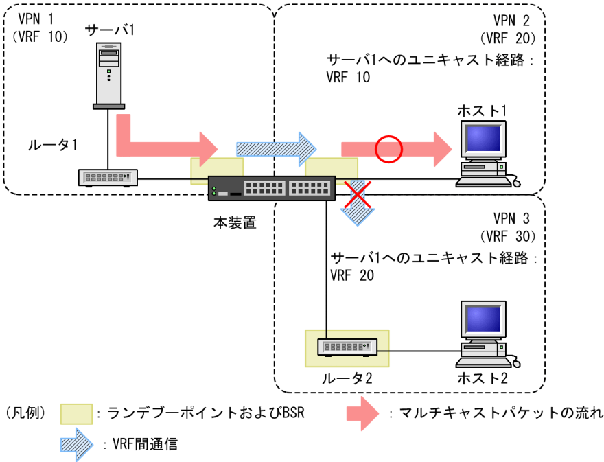
図 14-24 IPv4 マルチキャストエクストラネット使用時に装置内で VRF 中継を禁止している例
