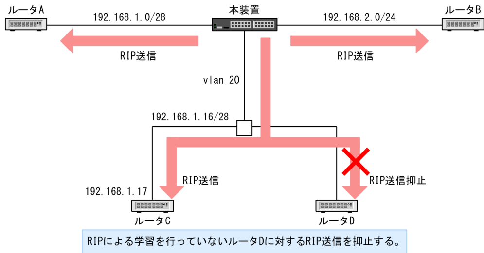
図 9-15 RIP パケット送信相手の限定
