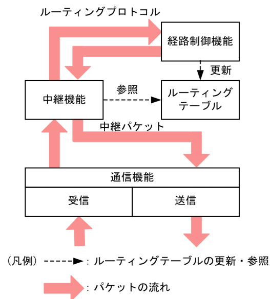
図 17-20 IPv6 ルーティング機能の概要
