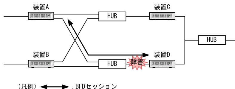
図 33-3 BFD セッションでの障害発生
