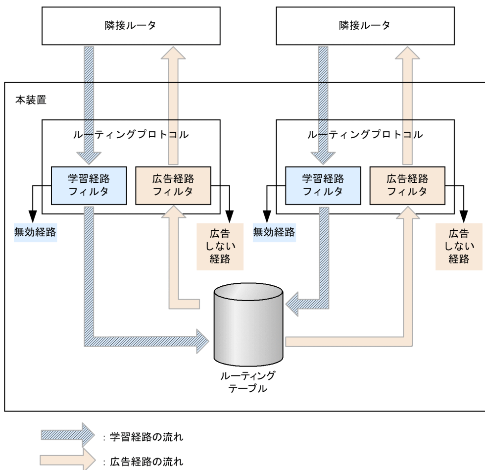
図 29-1 経路フィルタリングの概念図
