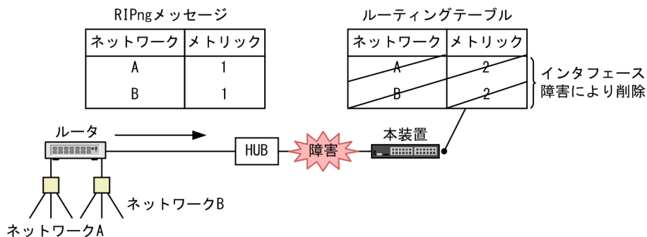
図 25-8 インタフェース障害による経路情報の削除
