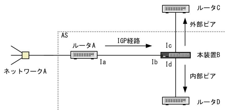
図 12-8 IGP 経路を BGP4 で広告する場合に通知する経路情報の NEXT_HOP 属性の設定例
