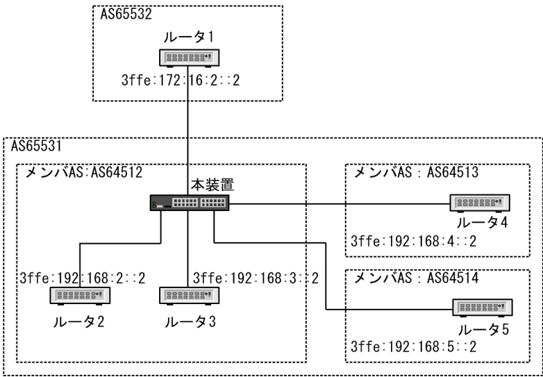
図 28-17 コンフェデレーション構成例
