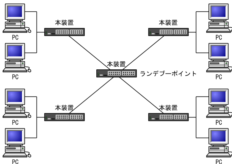
図 30-25 IPv6 PIM-SM を使用する構成図
