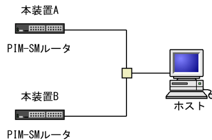
図 14-28 注意が必要な構成（複数ルータとホストの接続）
