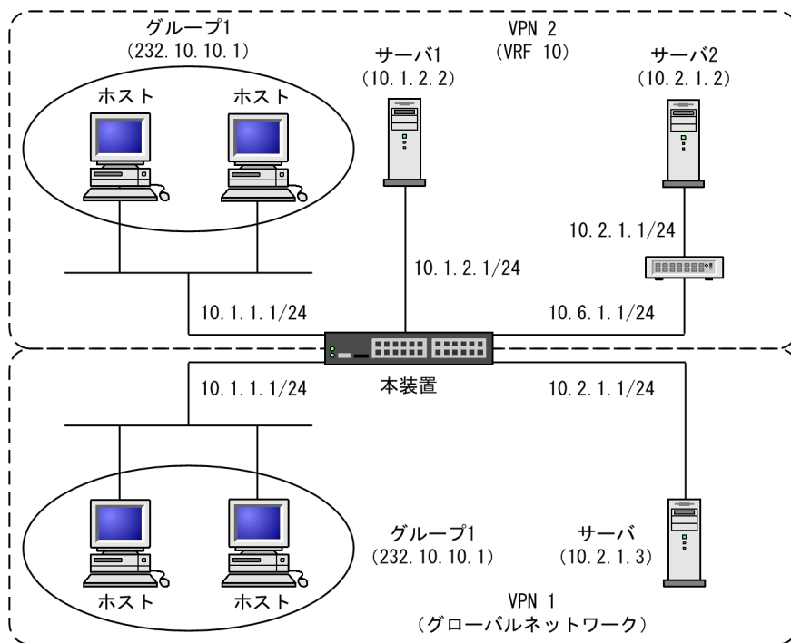
図 15-4 VRF での IPv4 PIM-SSM 構成例
