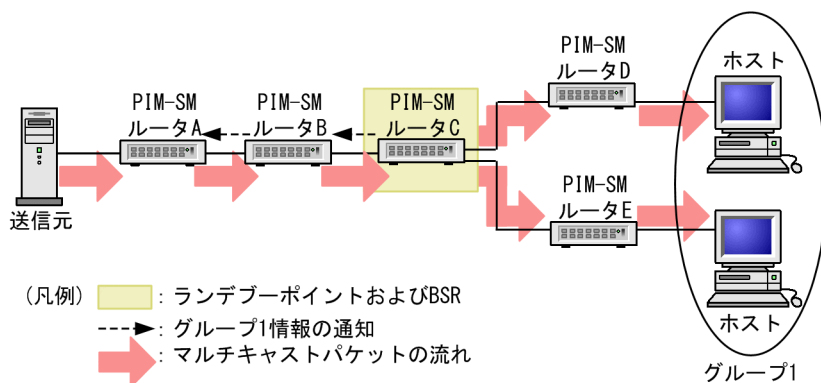
図 14-11 ランデブーポイント経由のマルチキャストパケット通信（デカプセル化）
