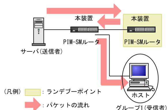
図 14-34 不適応な構成（送信者とランデブーポイントの間に受信者が存在する場合）
