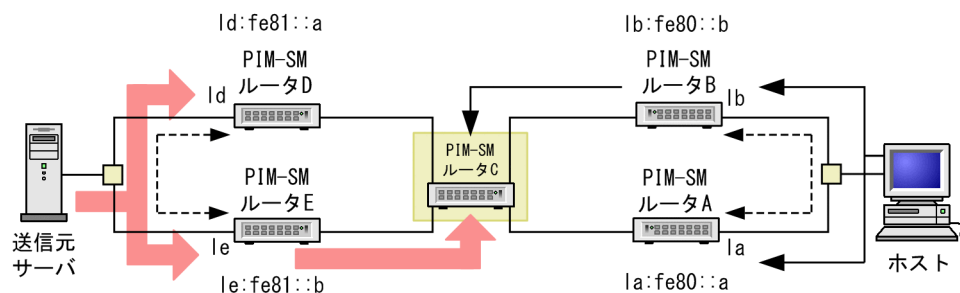
図 30-15 DR の動作
