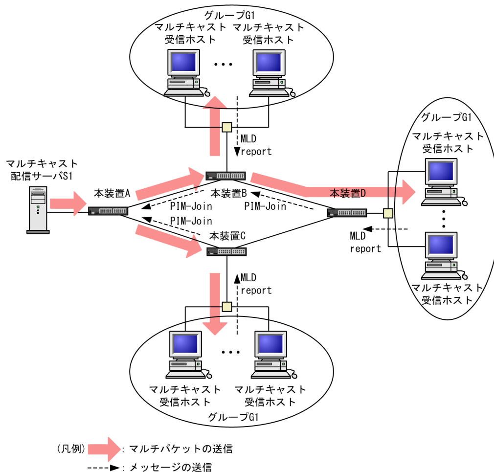
図 30-18 IPv6 PIM-SSM の動作概要（ホストが MLDv1 または MLDv2（EXCLUDE モード）の場合）
