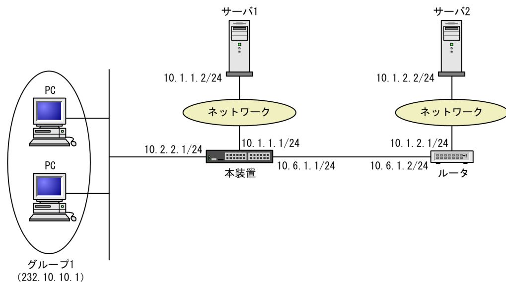
図 15-2 PIM-SSM 構成例
