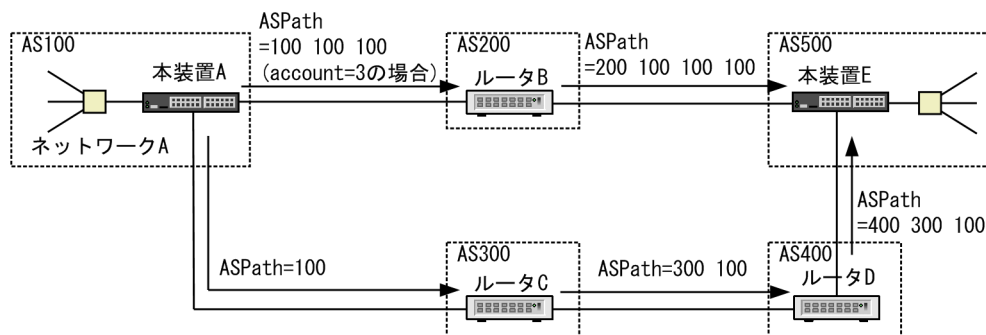
図 28-4 set as-path prepend count コマンドの使用例
