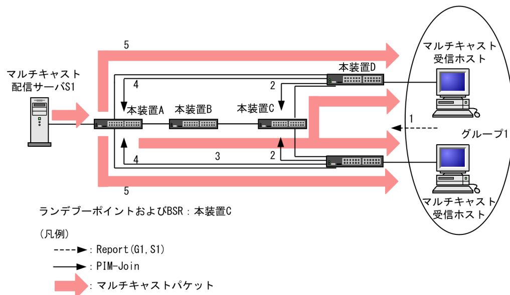
図 30-16 MLDv2 使用時の IPv6 PIM-SM 動作概要
