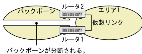
図 27-4 バックボーン分断に対する予備経路
