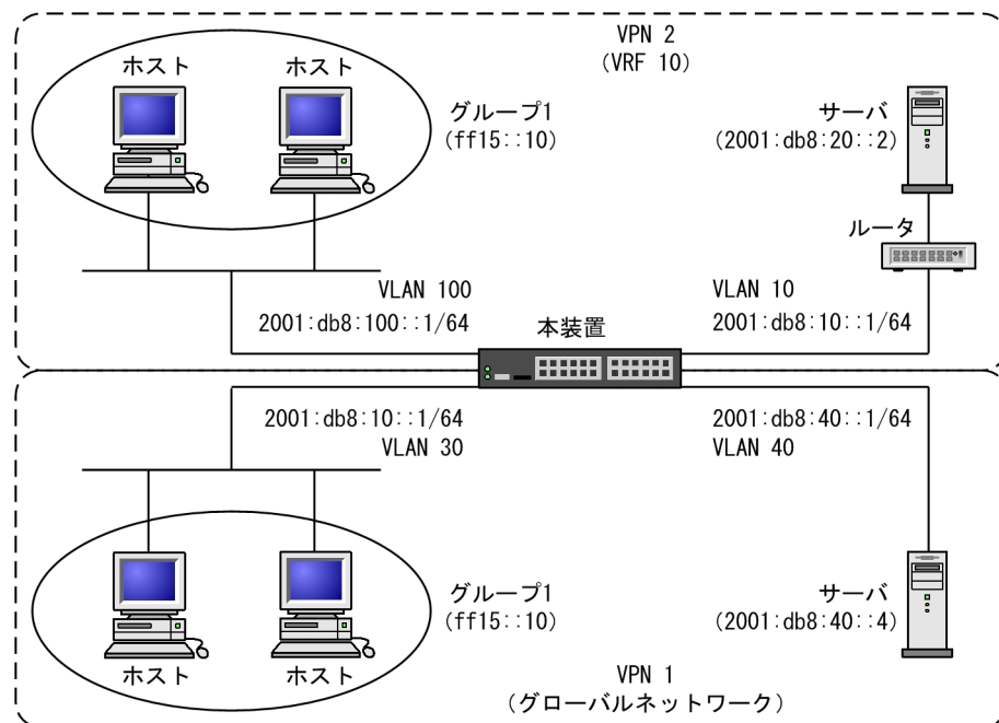
図 31-4 VRF での MLD 構成例
