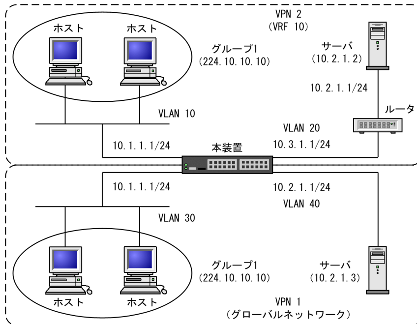
図 15-6 VRF での PIM-SSM 構成例（IPv4 マルチキャストエクストラネット）
