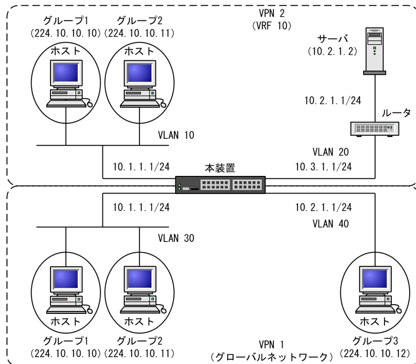
図 15-7 VRF での PIM-SM 構成例（PIM-SM VRF ゲートウェイ）
