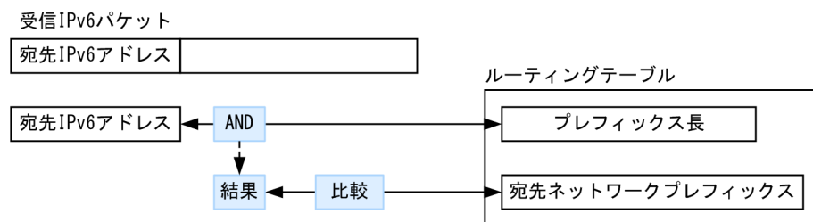
図 17-23 ルーティングテーブルの検索
