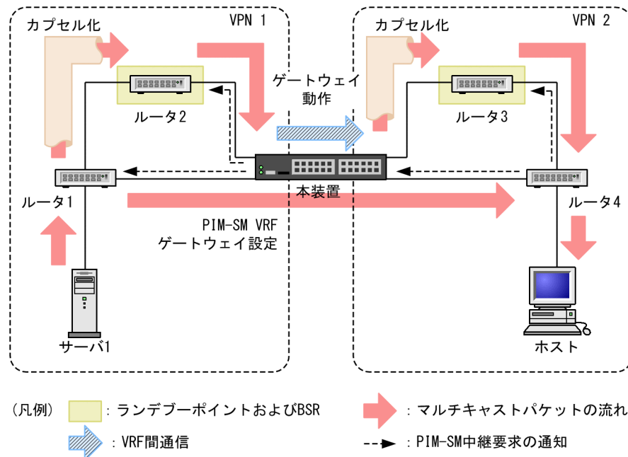
図 14-23 PIM-SM VRF ゲートウェイの動作概要
