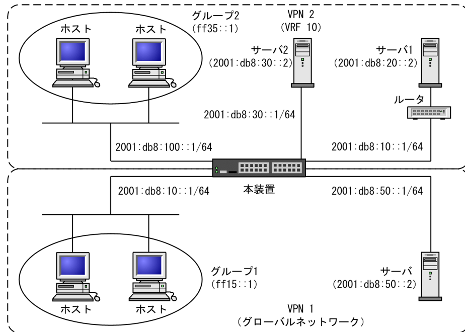
図 31-3 VRF での IPv6 PIM-SSM 構成例
