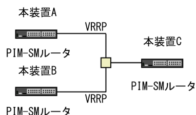
図 30-29 注意が必要な構成 (VRRP を設定した場合)
