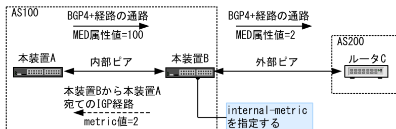
図 28-6 set metric-type internal の使用例
