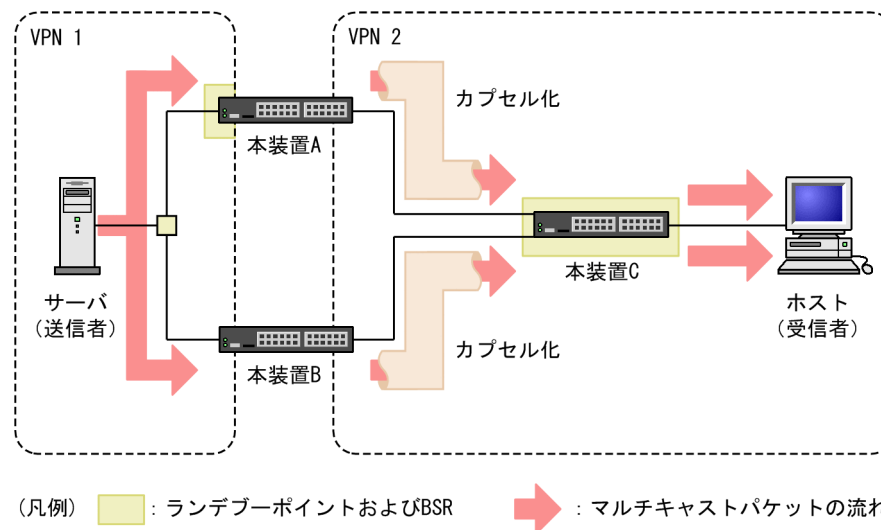
図 14-36 注意が必要な構成（2 台以上の VRF 境界ルータで冗長構成を構築する場合）
