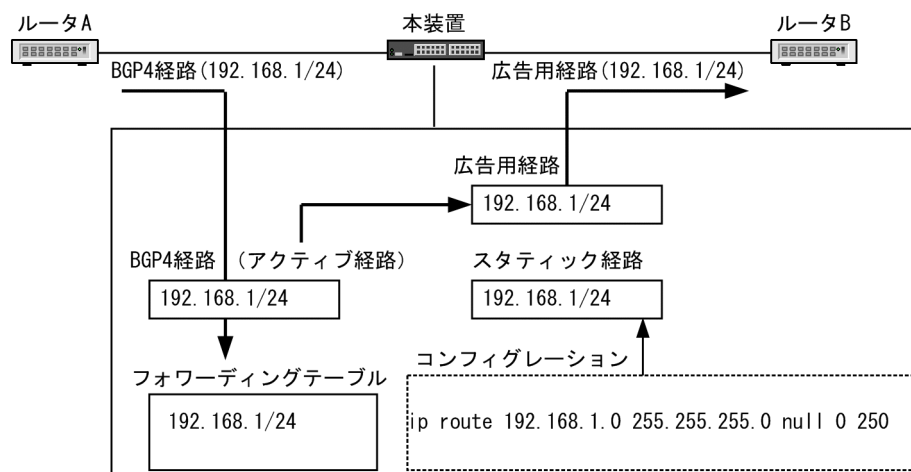
図 12-20 広告用経路生成と広告（通常の場合）
