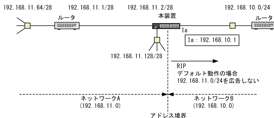
図 9-12 直結経路を広告しない構成例
