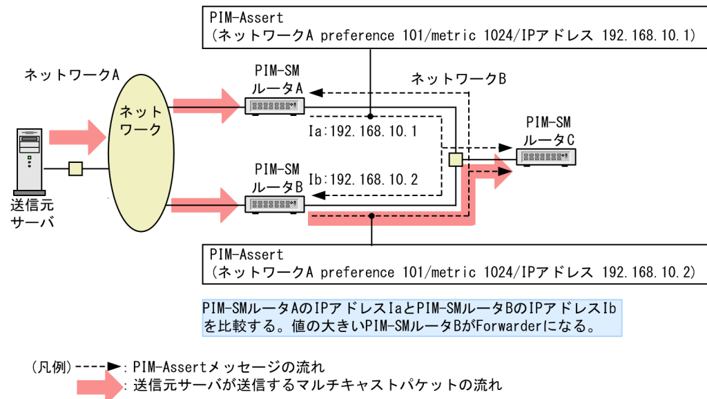
図 14-14 Forwarder の決定
