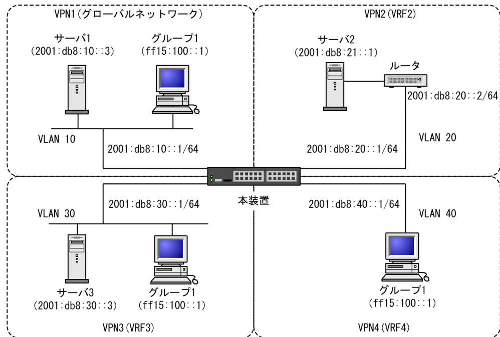
図 32-2 IPv6 マルチキャストエクストラネットの構成例
