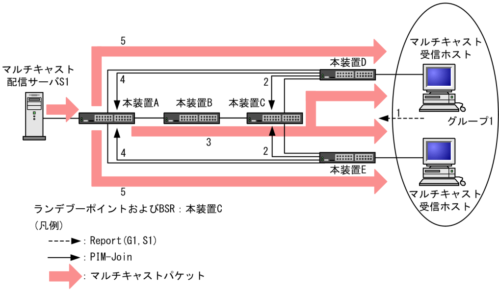
図 14-20 IGMPv3 使用時の IPv4 PIM-SM 動作概要
