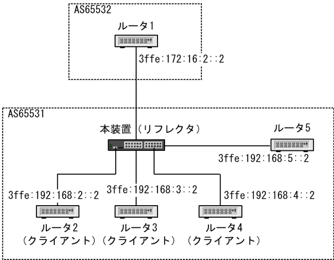
図 28-16 ルート・リフレクション構成例
