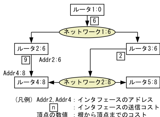
図 26-3 ルータ 1 を根とする最短木
