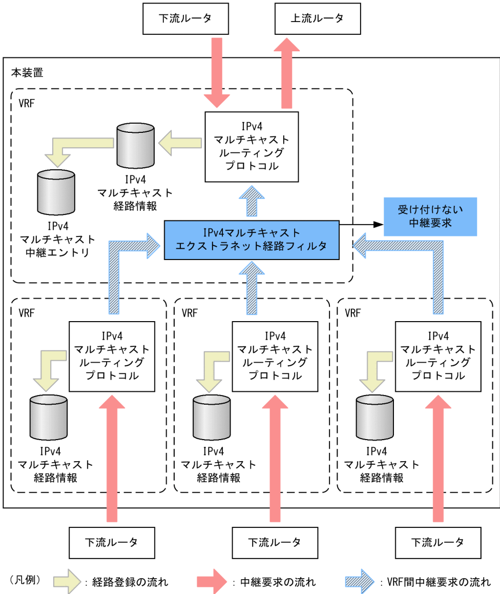
図 16-1 IPv4 マルチキャストエクストラネットの経路フィルタリングの概念図
