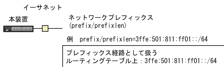
図 23-3 直結経路の取り扱い（ブロードキャスト型の場合）
