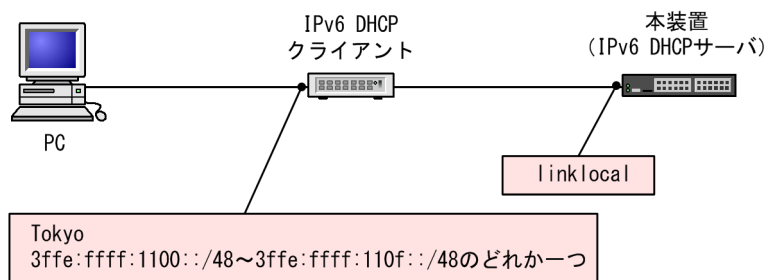
図 22-2 動的にプレフィックスを割り当てる構成
