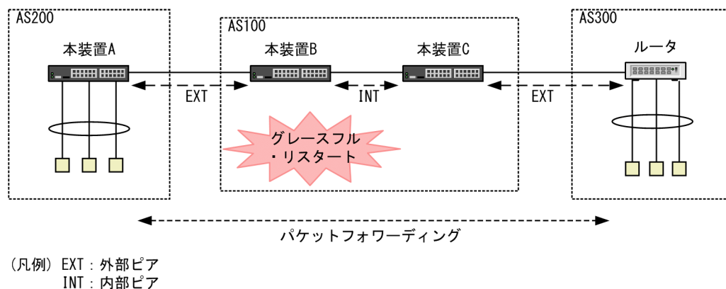
図 12-28 グレースフル・リスタートの例
