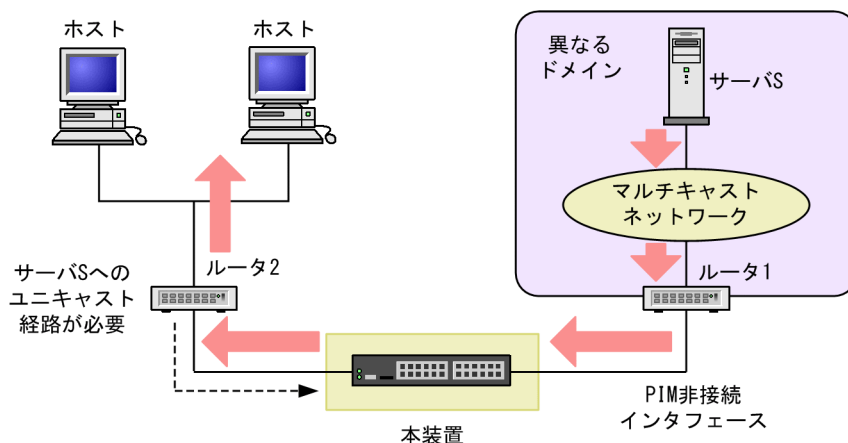
図 30-30 注意が必要な構成 (PIM 非接続インタフェース経由の中継)
