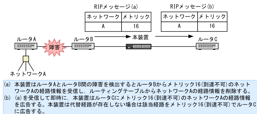
図 9-4 ルートポイズニング
