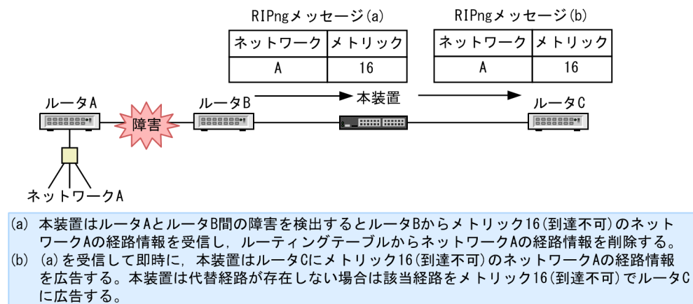
図 25-4 ルートポイズニング
