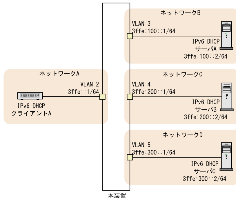
図 21-3 1 台の IPv6 DHCP リレーを経由するユニキャスト送信時の構成
