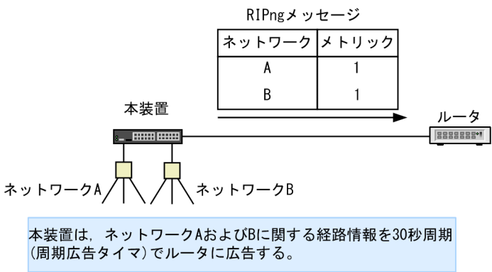
図 25-1 周期的な経路情報広告
