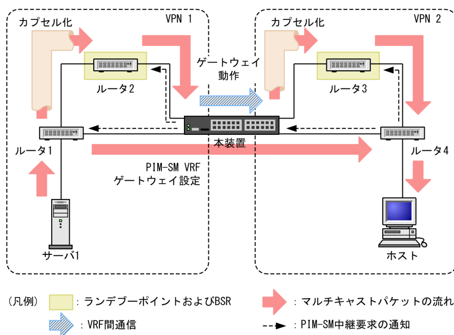
図 30-22 PIM-SM VRF ゲートウェイの動作概要
