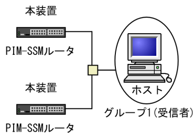
図 30-34 注意が必要な構成（複数ルータとホストの接続）
