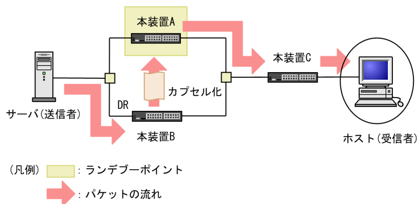
図 14-33 注意が必要な構成（複数ルータと送信者の接続）
