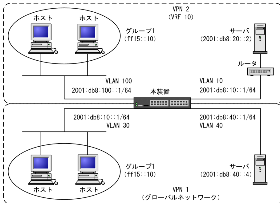
図 31-2 VRF での IPv6 PIM-SM 構成例
