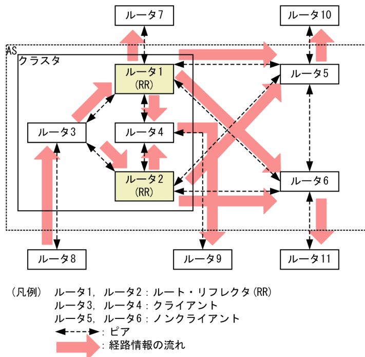
図 12-24 ルート・リフレクタの冗長構成の例
