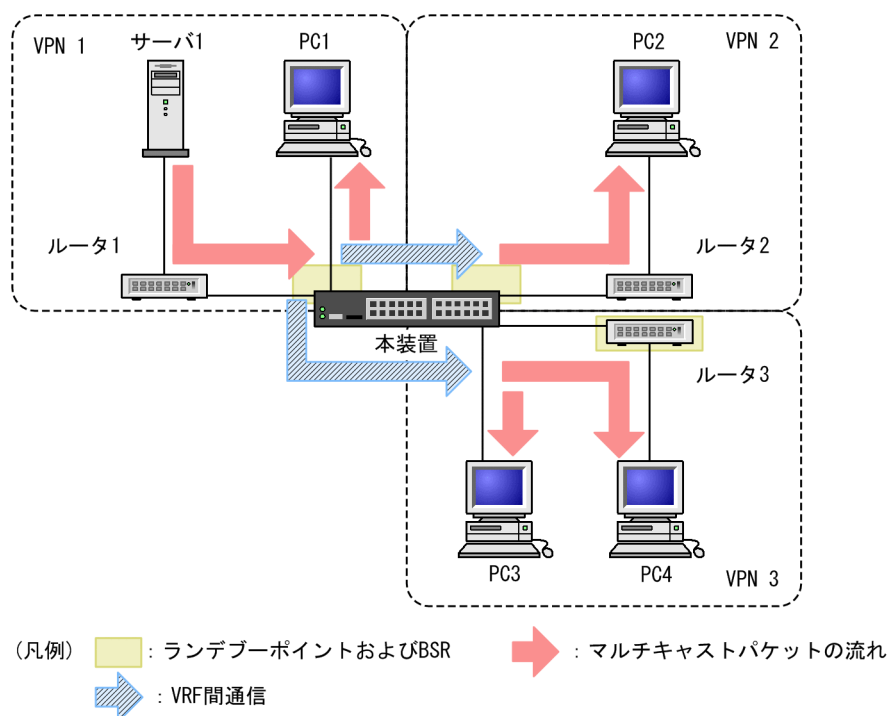
図 14-22 IPv4 マルチキャストエクストラネットの動作概要
