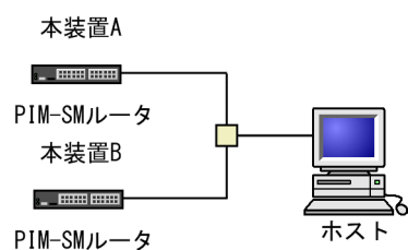
図 30-28 注意が必要な構成（複数ルータとホストの接続）
