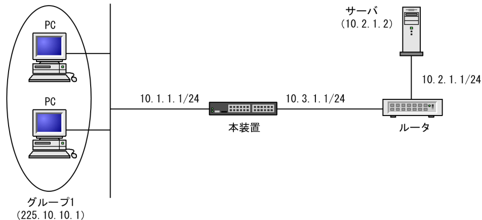
図 15-1 PIM-SM 構成例
