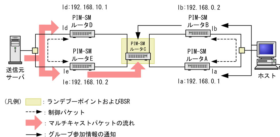
図 14-15 DR の動作
