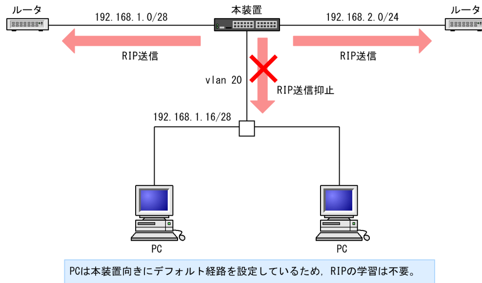
図 9-14 RIP パケットの送信抑止
