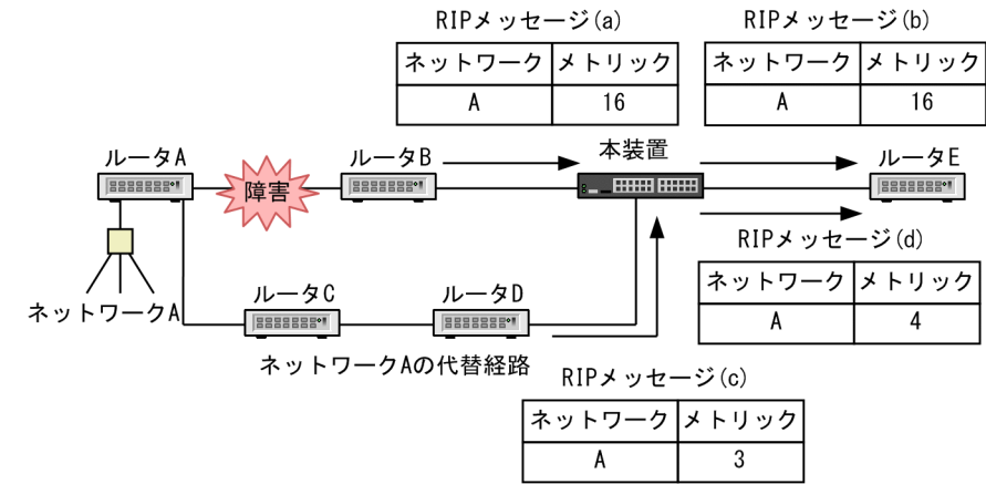
図 9-5 ルートポイズニング期間中の再学習
