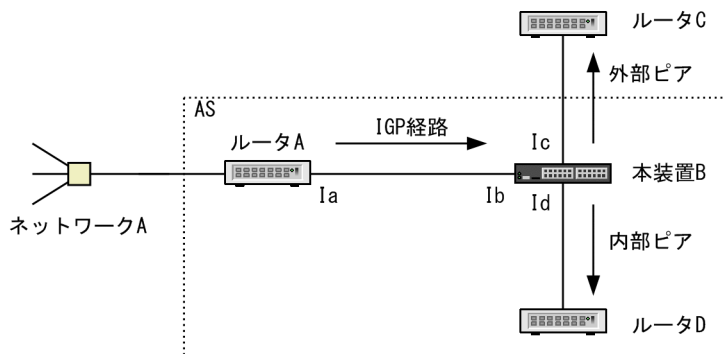
図 28-8 IGP 経路を BGP4+で広告する場合に通知する経路情報のネクストホップの設定例
