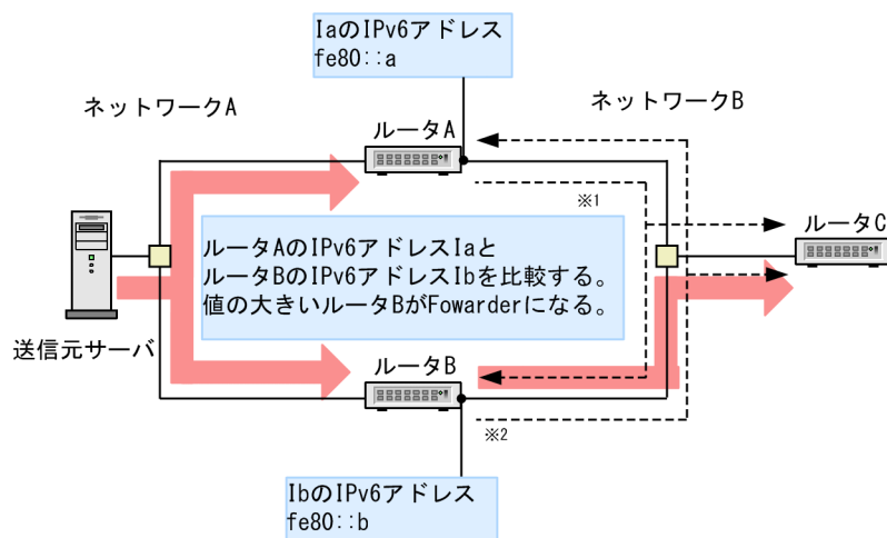
図 30-14 Forwarder の決定
