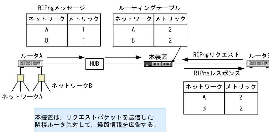
図 25-3 リクエストパケット受信による経路情報の広告
