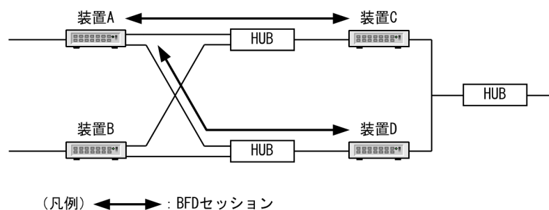
図 33-1 BFD の基本動作
