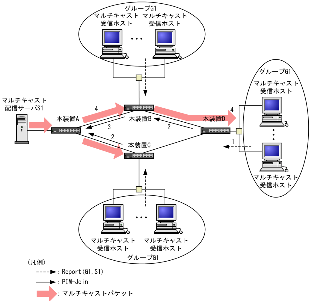
図 30-19 IPv6 PIM-SSM 動作概要（ホストが MLDv2（INCLUDE モード）の場合）
