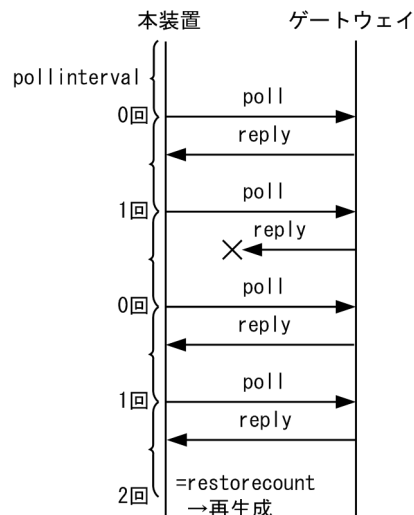
図 8-5 スタティック経路の動的監視による経路再生成 (restorecount =2 の場合)
