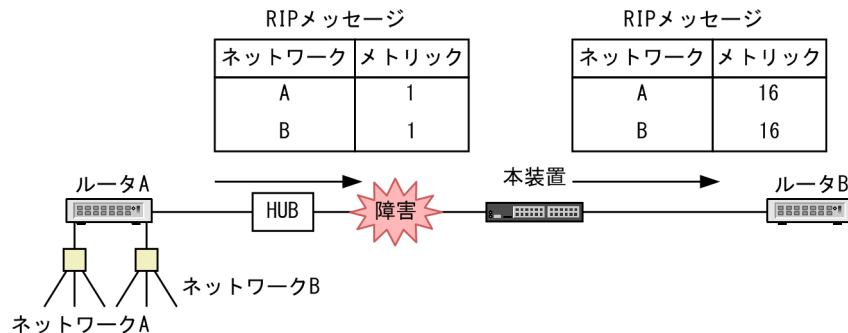
図 9-2 triggered update による経路情報の広告
