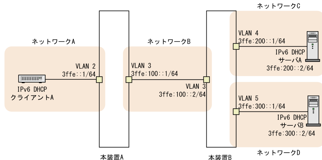
図 21-5 複数の IPv6 DHCP リレーを経由する構成
