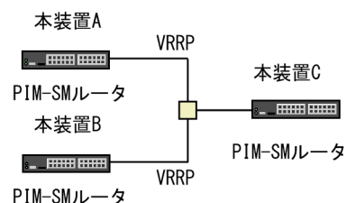
図 14-30 注意が必要な構成（VRRP を設定した場合）
