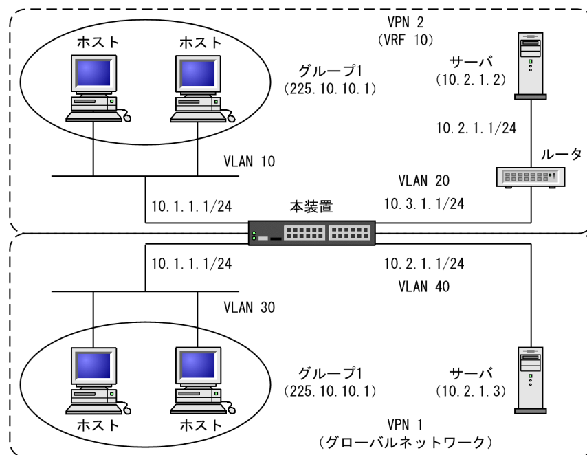
図 15-5 VRF での IGMP 構成例
