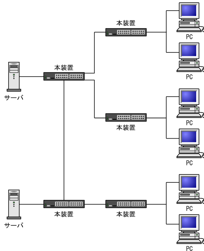
図 14-27 PIM-SSM を使用する構成図
