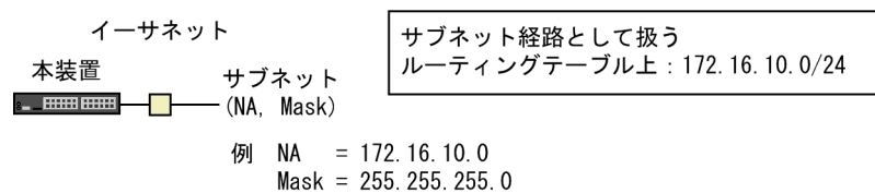
図 7-10 直結経路の取り扱い
