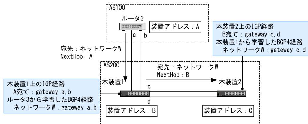
図 12-16 IGP 経路のマルチパス化による BGP4 経路マルチパス化の概念
