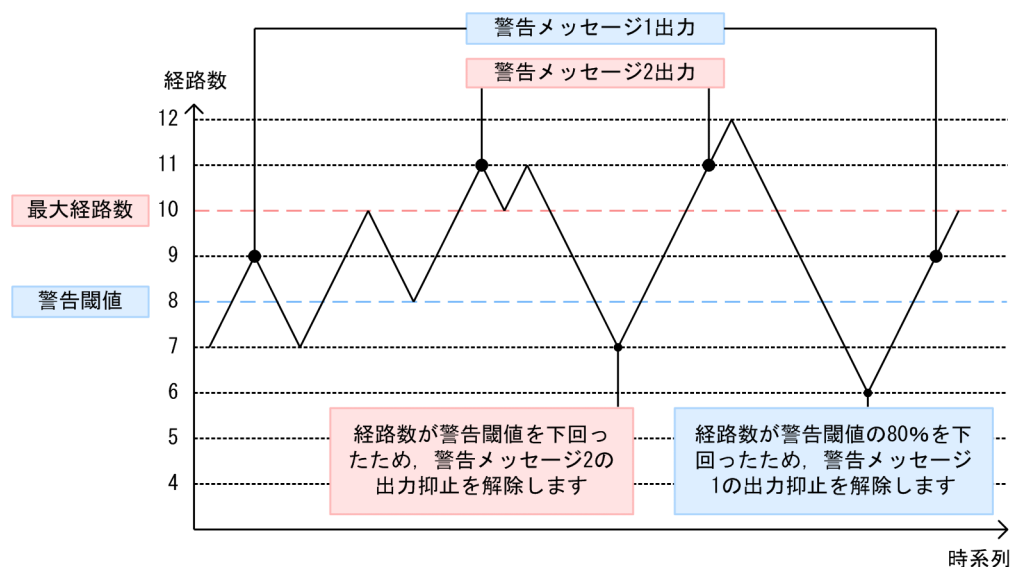
図 23-11 経路数と警告メッセージ出力の関係
