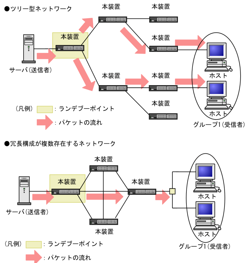
図 14-32 PIM-SM 推奨ネットワーク構成
