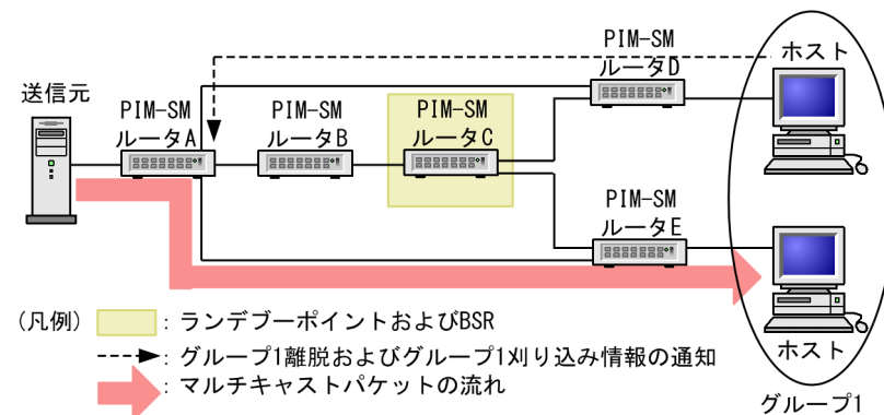
図 30-12 IPv6 マルチキャスト配送ツリーの刈り込み
