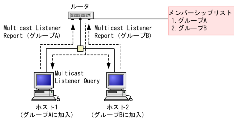
図 30-2 MLDv1 グループ参加・離脱動作
