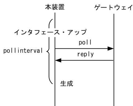
図 24-3 スタティック経路の動的監視による経路生成
