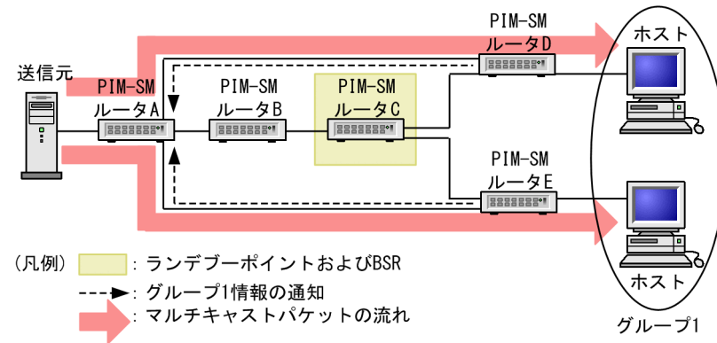
図 30-11 最短パスの IPv6 マルチキャストパケット通信
