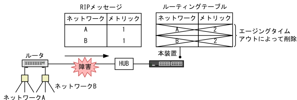
図 9-9 エージングタイムアウトによる経路情報の削除
