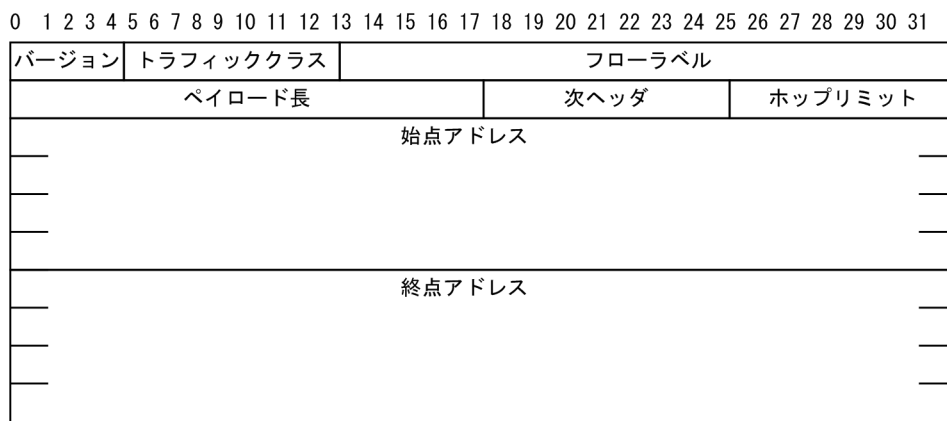
図 17-22 IPv6 ヘッダ形式
