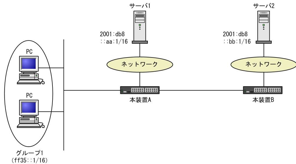
図 31-1 PIM-SSM 構成例
