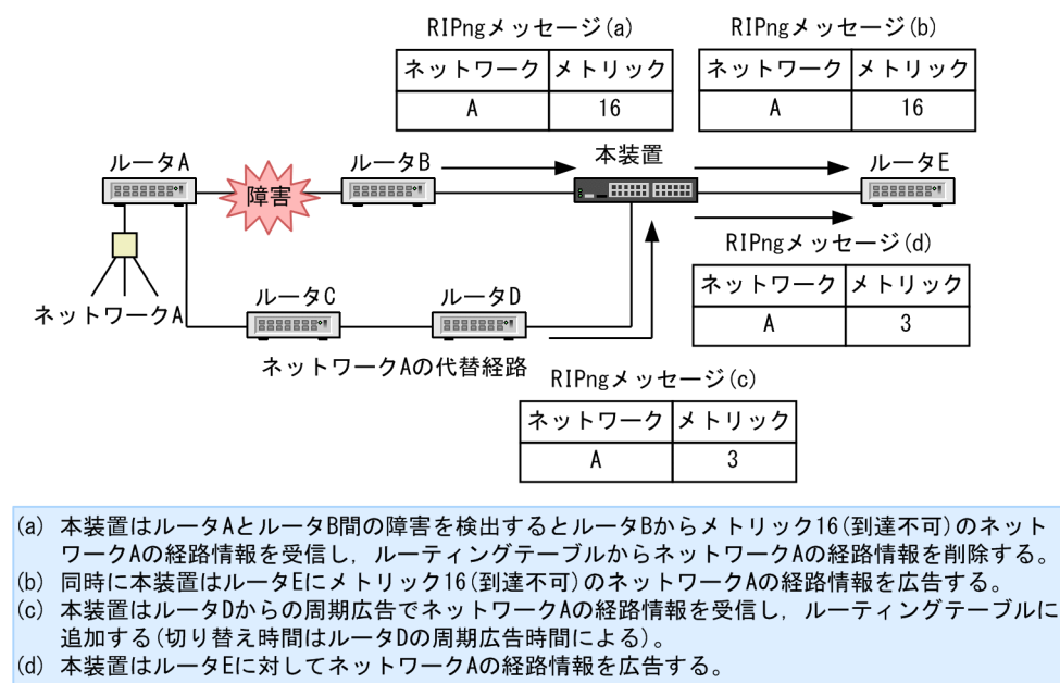
図 25-5 ルートポイズニング期間中の再学習
