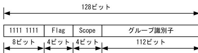
図 30-1 マルチキャストアドレスのフォーマット
