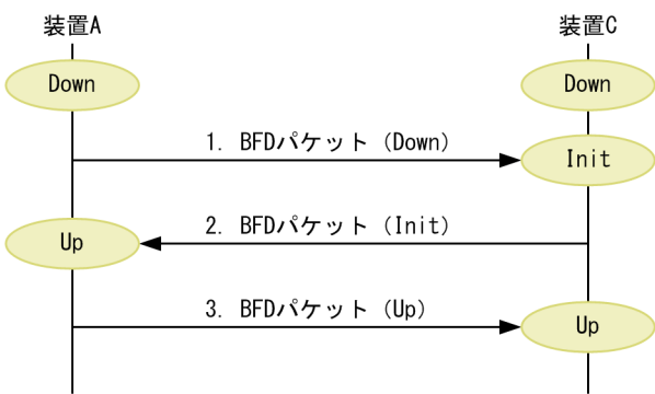
図 33-2 BFD の状態遷移
