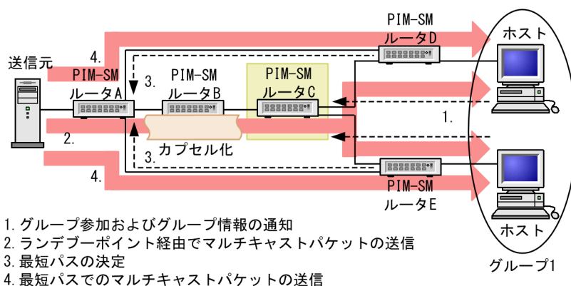
図 14-7 PIM-SM の動作概要
