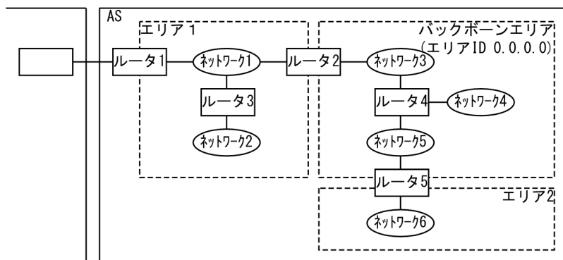
図 27-1 エリア分割を使用した OSPFv3 ネットワークトポロジの例
