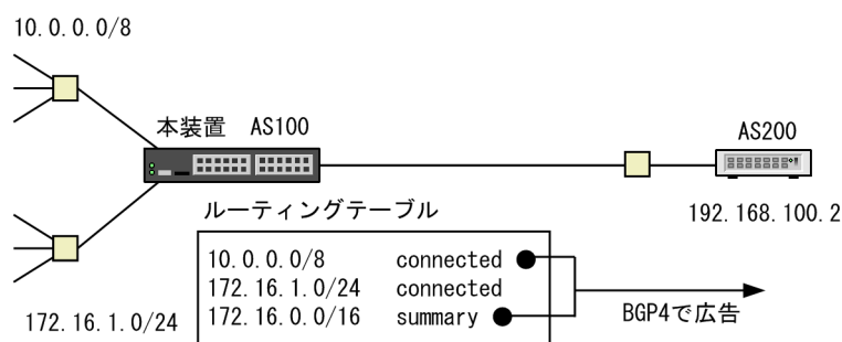
図 7-18 集約経路を BGP4 で広告する構成
