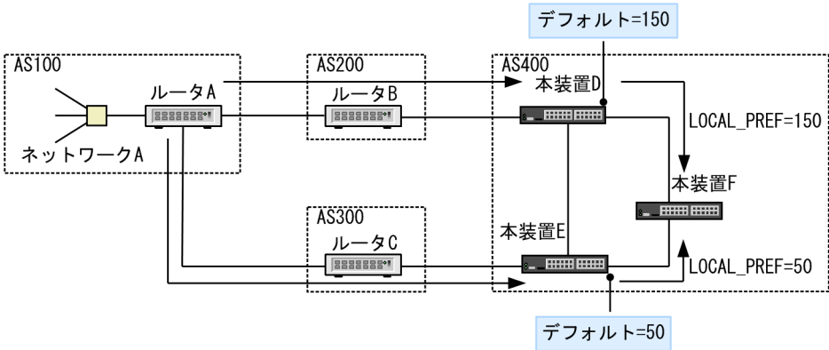
図 12-2 LOCAL_PREF 属性による経路選択
