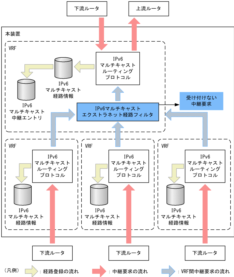
図 32-1 IPv6 マルチキャストエクストラネットの経路フィルタリングの概念図
