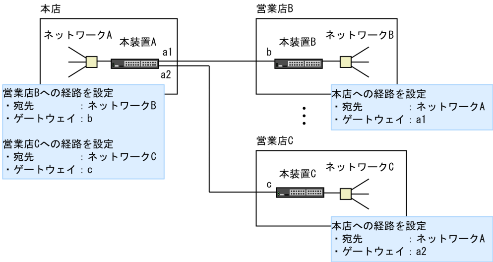
図 24-1 スタティックルーティングのネットワーク構成例
