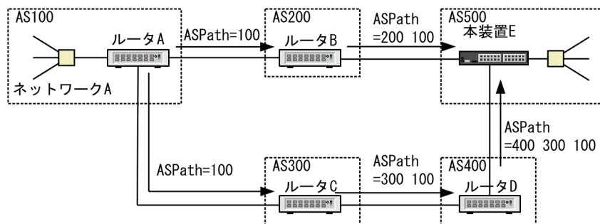
図 28-3 AS_PATH 属性による経路選択
