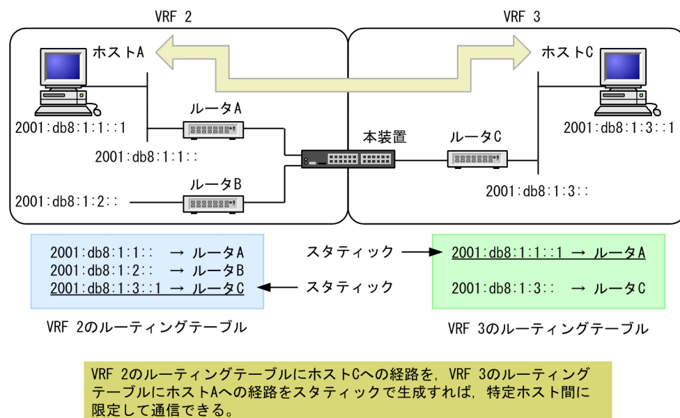
図 23-13 VRF 間にわたるスタティックルーティング
