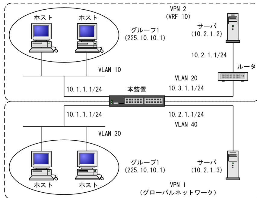
図 15-3 VRF での IPv4 PIM-SM 構成例
