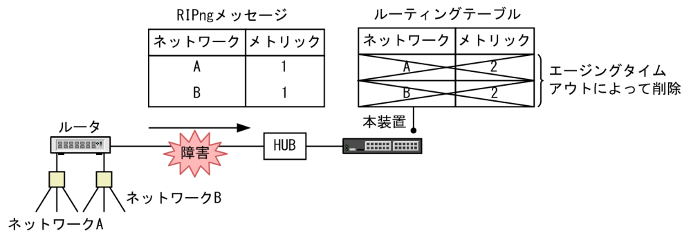
図 25-7 エージングタイムアウトによる経路情報の削除
