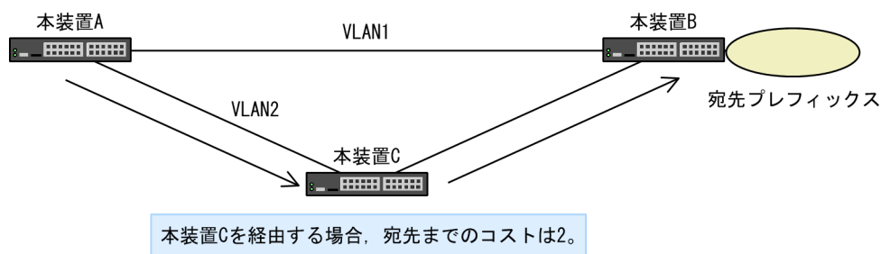
図 26-5 マルチパスの構成
