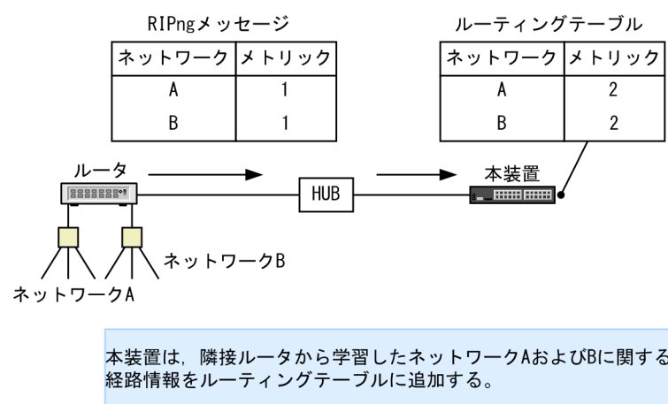
図 25-6 レスポンスパケット受信による経路情報の生成
