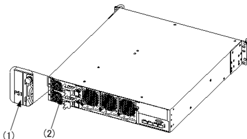
図 4-50 電源機構の搭載位置の確認
