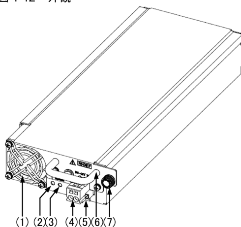
図 1-12 外観
