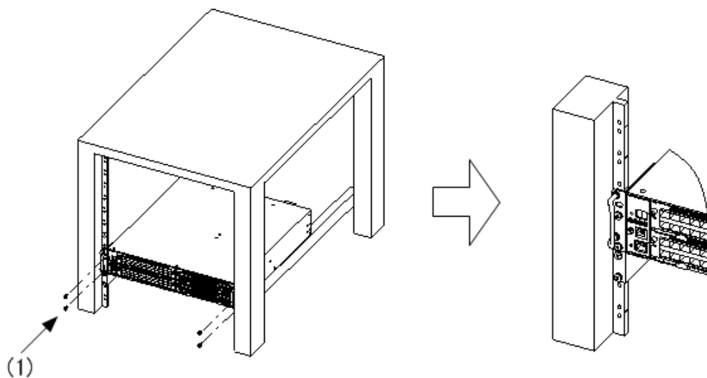
図 4-8 ラックへの固定
