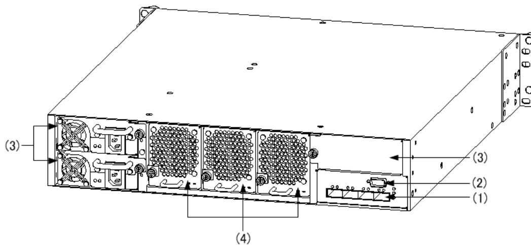
図 1-2 背面外観（AC 電源機構搭載時）
