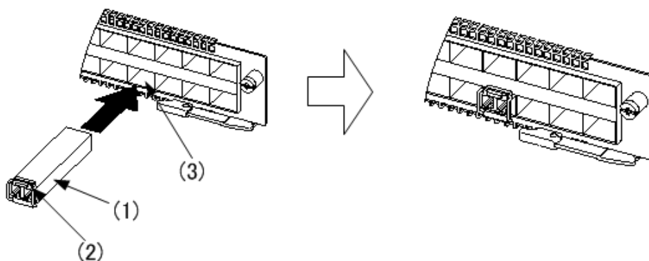
図 4-29 SFP の取り付け（下側のポート）
