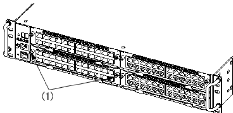
図 5-20 ネットワークインタフェース機構の取り付け -4
