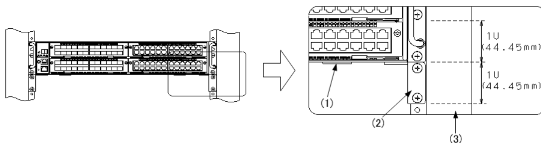
図 4-6 ガイドレールの取り付け位置
