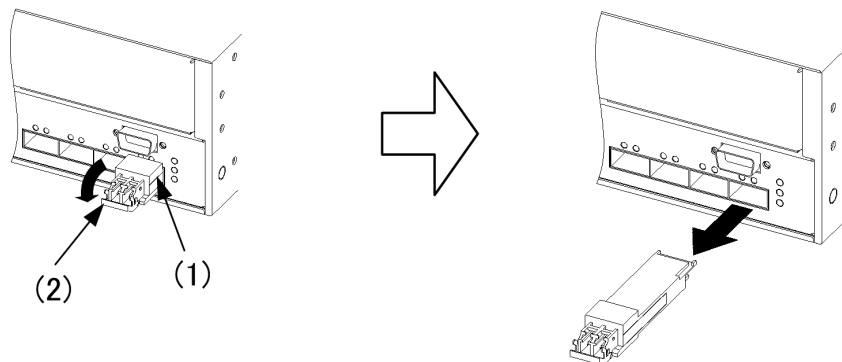
図 4-34 QSFP+ の取り外し（レバータイプの場合）
