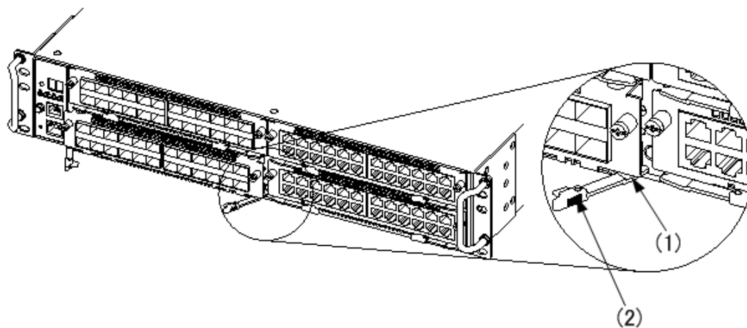
図 5-18 ネットワークインタフェース機構の取り付け -2
