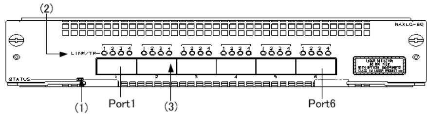
図 1-18 正面外観
