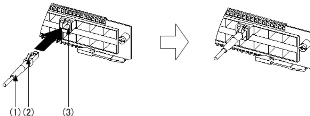
図 4-43 光ファイバケーブル（LC1 芯コネクタ：上側のポート）
