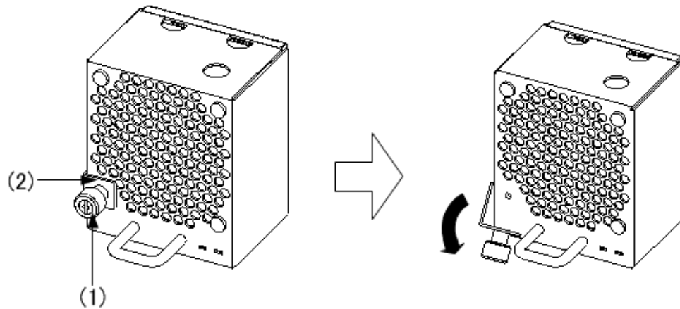
図 5-3 ファンユニットの取り付け -1
