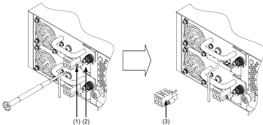
図 4-13 ケーブル用コネクタの取り外し
