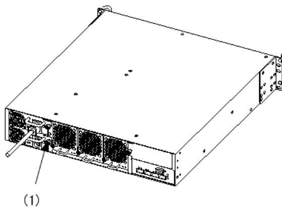
図 5-7 電源機構の取り外し -1
