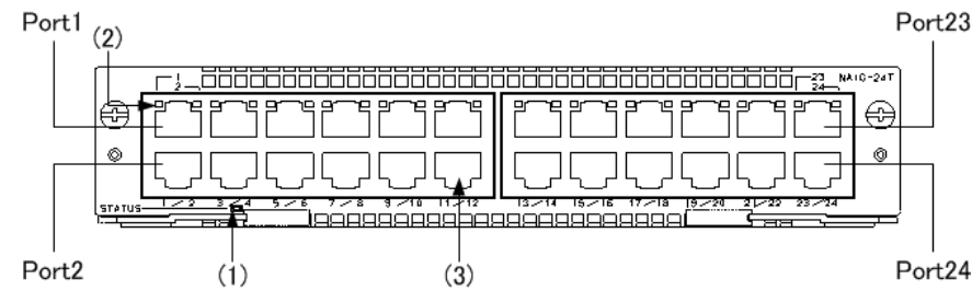
図 1-15 正面外観
