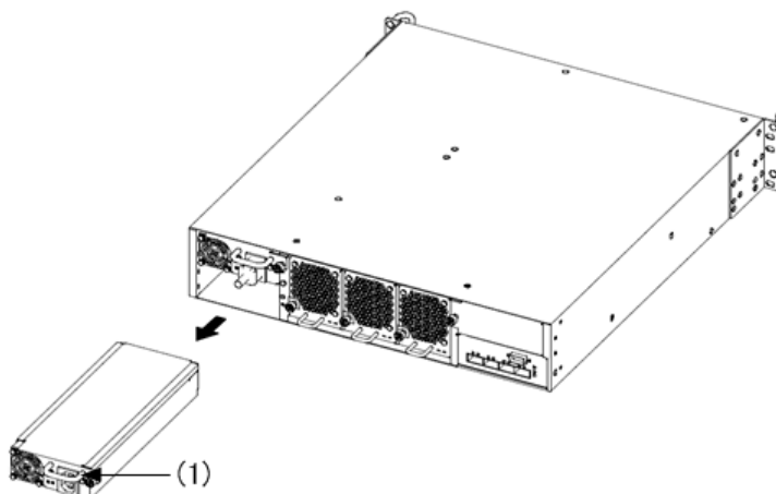
図 5-8 電源機構の取り外し -2
