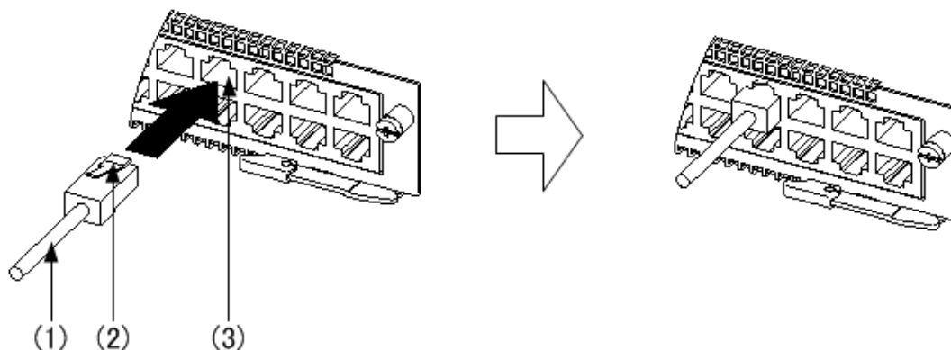
図 4-39 UTP ケーブルの取り付け（上側のポート）
