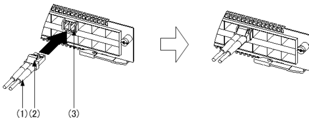
図 4-41 光ファイバケーブル（LC2 芯コネクタ：上側のポート）
