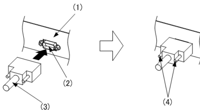
図 4-38 RS-232C ケーブルの取り付け（運用端末側）
