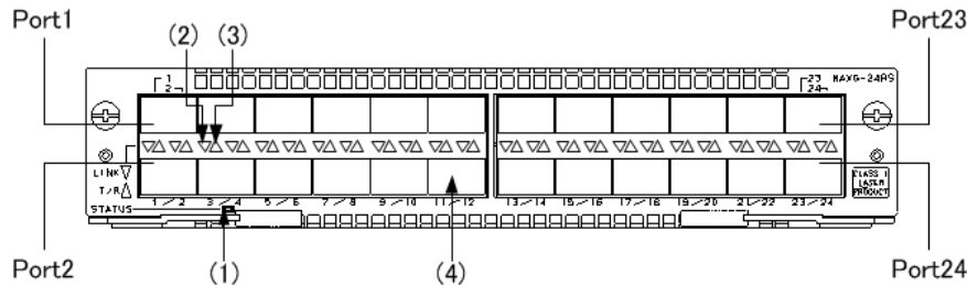
図 1-17 正面外観
