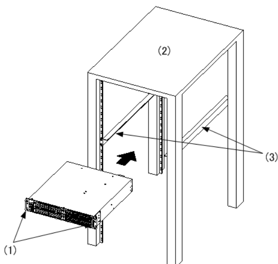
図 4-7 ラックへの搭載
