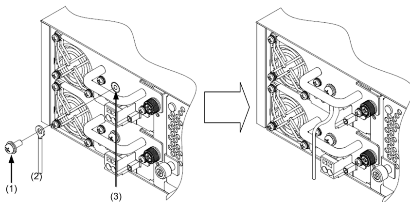
図 4-12 接地用ケーブル用の取り付け
