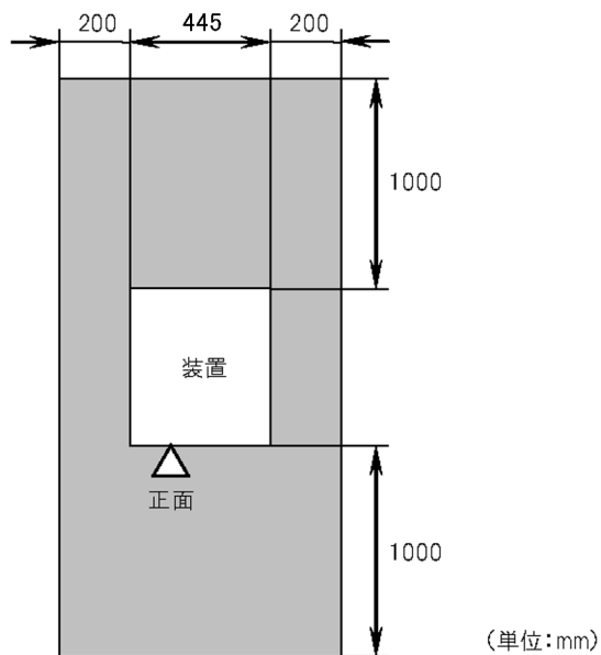
図 2-7 卓上設置時の保守エリア
