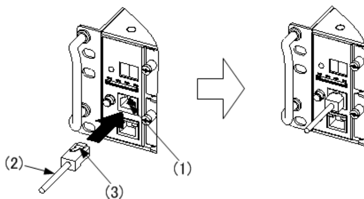
図 4-37 RS-232C ケーブルの取り付け (本装置側)
