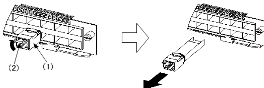
図 4-27 SFP-T の取り外し（下側のポート）
