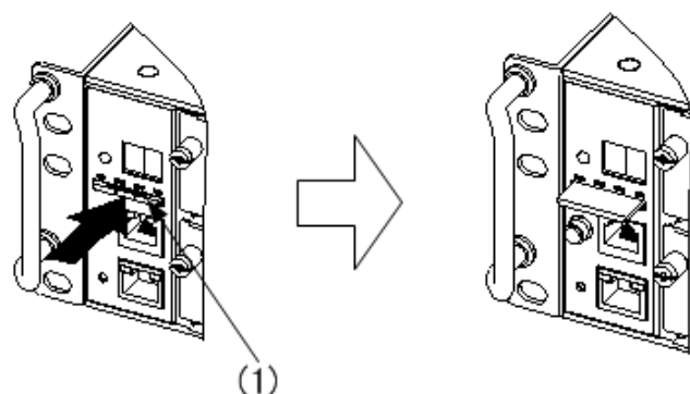
図 4-22 ダミーメモリカードの取り外し方
