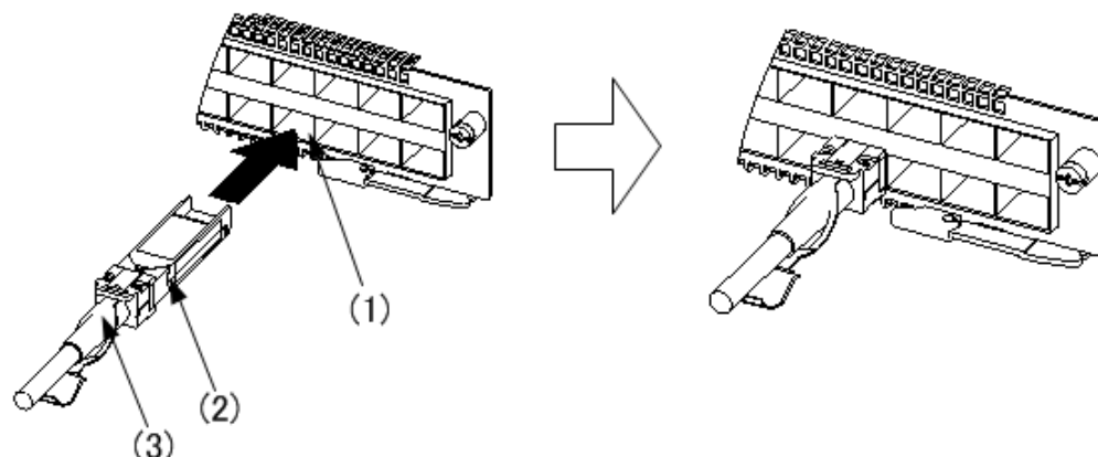
図 4-47 ダイレクトアタッチケーブル（SFP+ 用）の取り付け（下側のポート）
