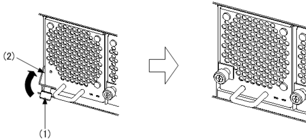
図 5-5 ファンユニットの取り付け -3
