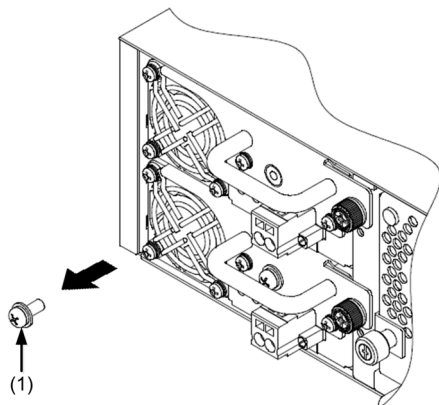
図 4-11 接地端子のネジと取り外し
