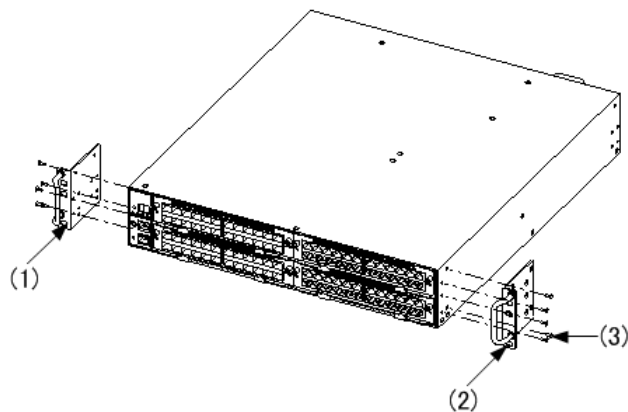
図 4-3 ラック取り付け金具の取り外し
