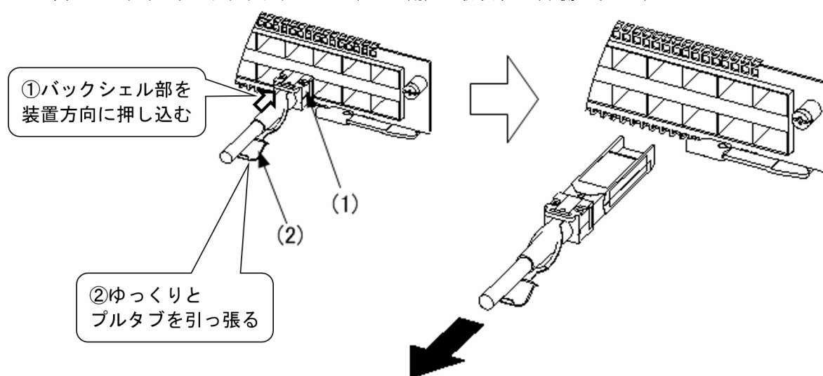
図 4-49 ダイレクトアタッチケーブル（SFP+ 用）の取り外し（下側のポート）
