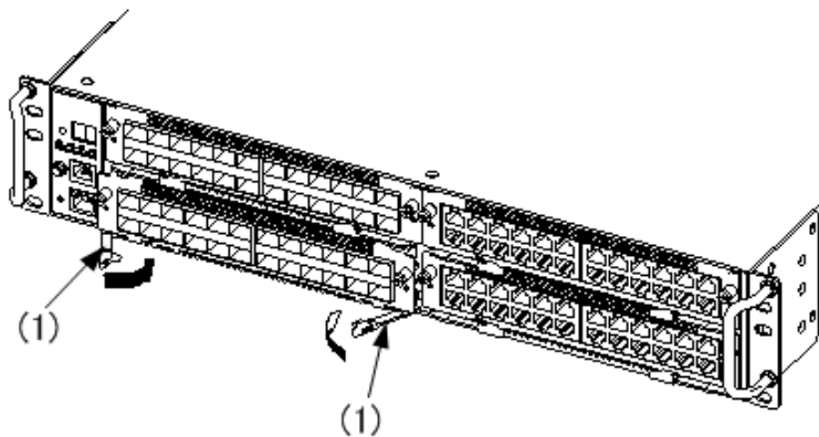
図 5-19 ネットワークインタフェース機構の取り付け -3
