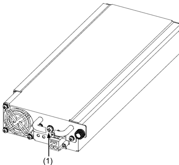
図 4-10 DC 電源機構背面
