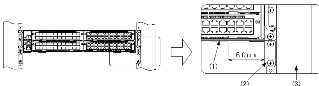
図 2-6 ガイドレールの詳細
