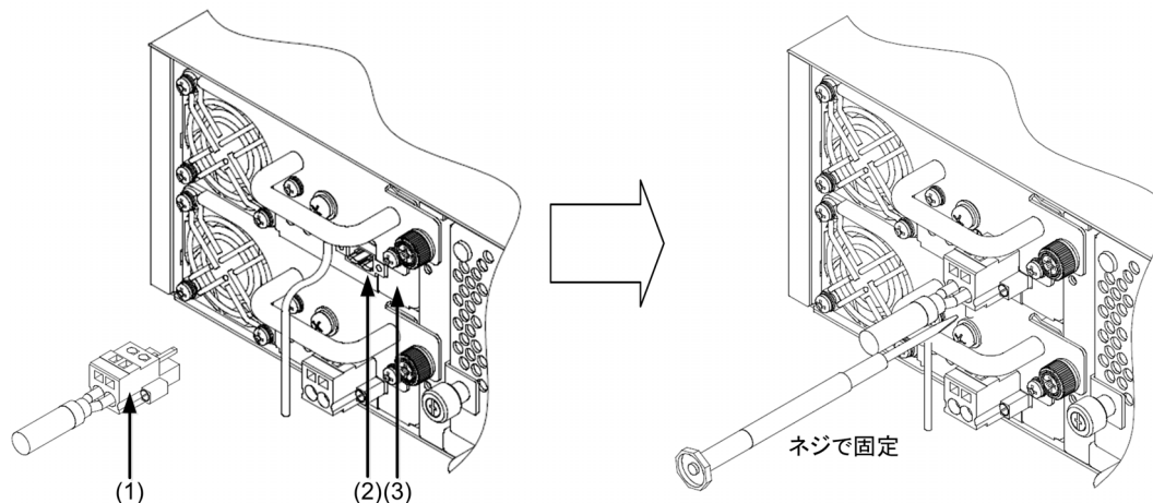
図 4-16 ケーブル用コネクタの取り付け
