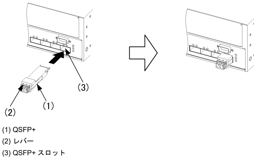
図 4-32 QSFP+ の取り付け（レバータイプの場合）
