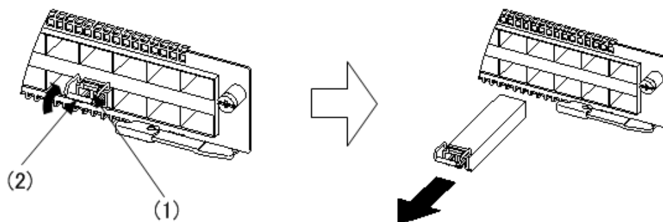
図 4-31 SFP の取り外し（下側のポート）
