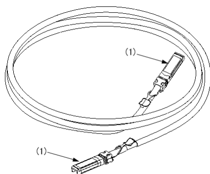
図 1-21 外観
