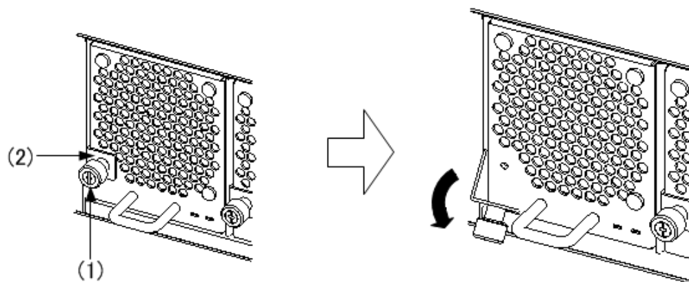
図 5-1 ファンユニットの取り外し -1
