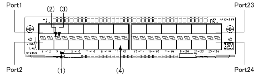
図 1-16 正面外観
