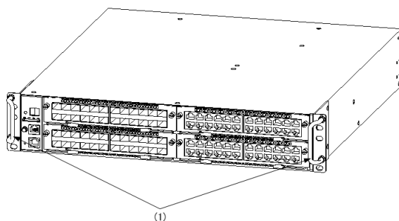
図 2-2 IP8800/S4630 の取っ手の位置（正面側）
