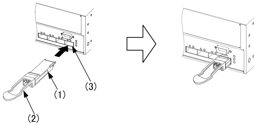
図 4-33 QSFP+ の取り付け（プルタブタイプの場合）
