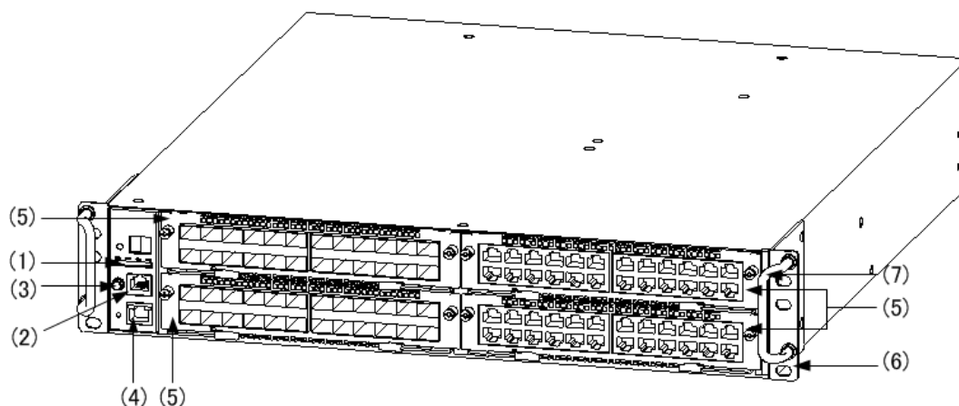
図 1-1 正面外観
