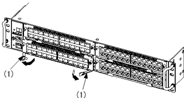
図 5-14 ネットワークインタフェース機構の取り外し -2
