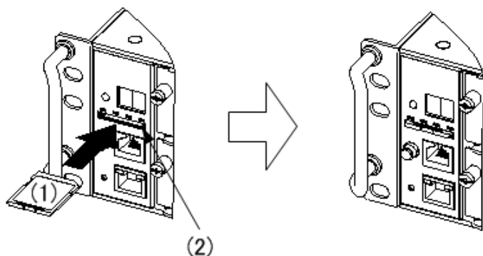
図 4-17 メモリカードの取り付け
