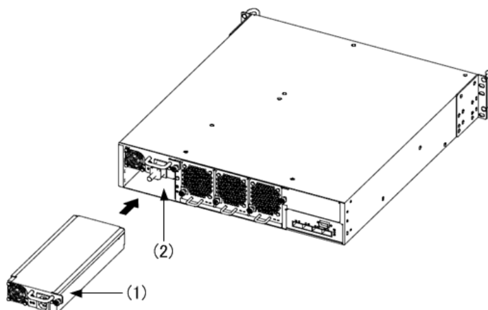
図 5-9 電源機構の取り付け-1
