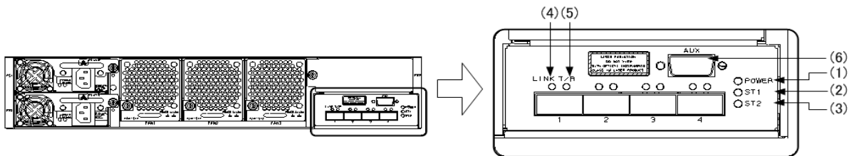
図 1-4 背面パネルレイアウト
