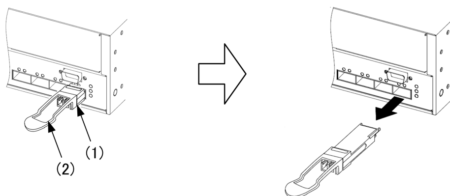
図 4-35 QSFP+ の取り外し（プルタブタイプの場合）
