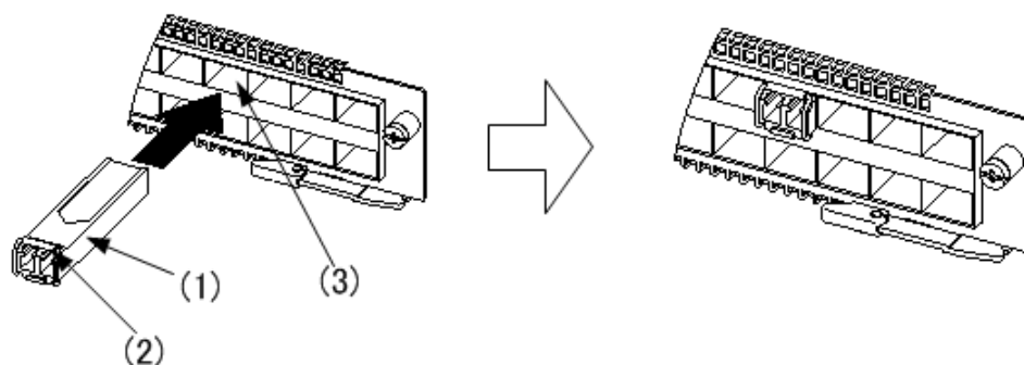
図 4-28 SFP の取り付け（上側のポート）
