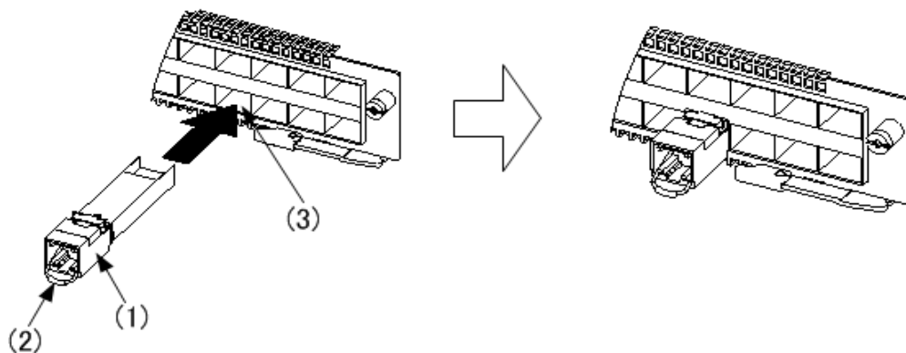
図 4-25 SFP-T の取り付け（下側のポート）
