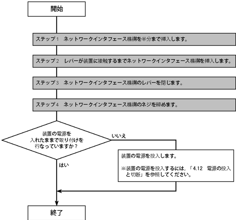
図 5-16 取り付けの操作の流れ
