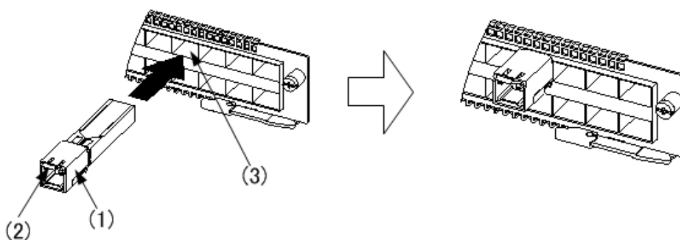
図 4-24 SFP-T の取り付け（上側のポート）
