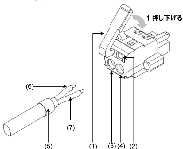
図 4-14 電源ケーブルの取り付け -1
