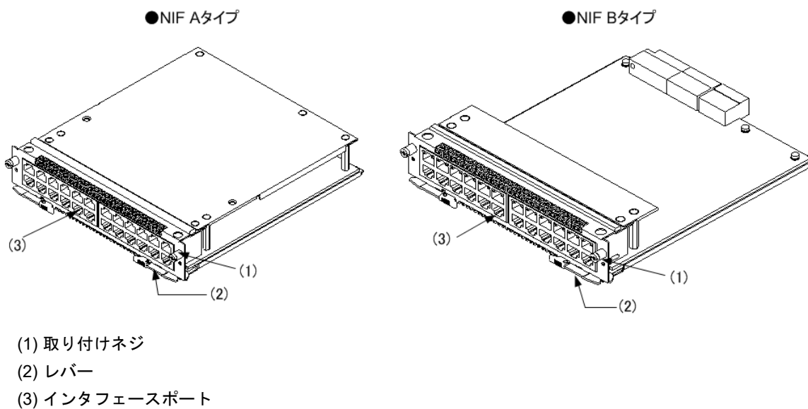
図 1-14 外観
