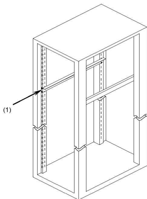
図 4-5 ガイドレールの取り付け
