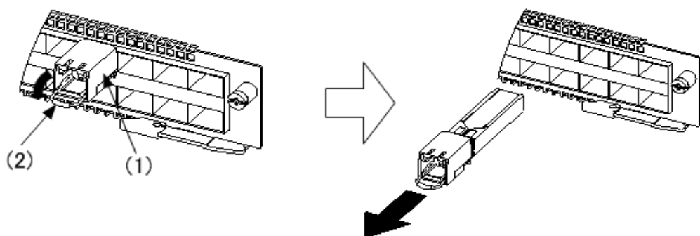
図 4-26 SFP-T の取り外し（上側のポート）
