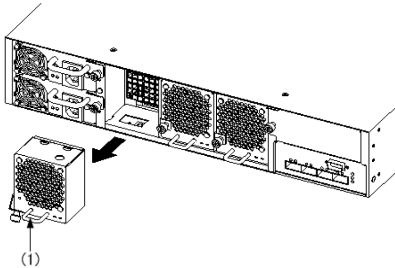
図 5-2 ファンユニットの取り外し -2
