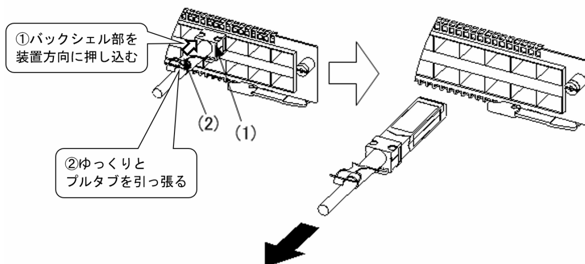
図 4-48 ダイレクトアタッチケーブル（SFP+ 用）の取り外し（上側のポート）
