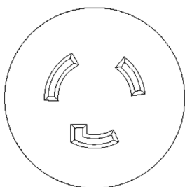
図 2-4 接地形 2 極引掛形コンセント (250V 20A)
