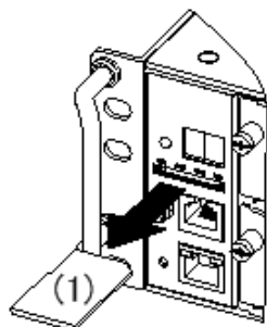
図 4-20 メモ리카ードの取り出し
