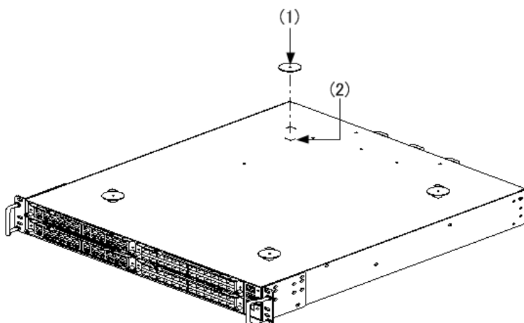
図 4-1 ゴム足の取り付け
