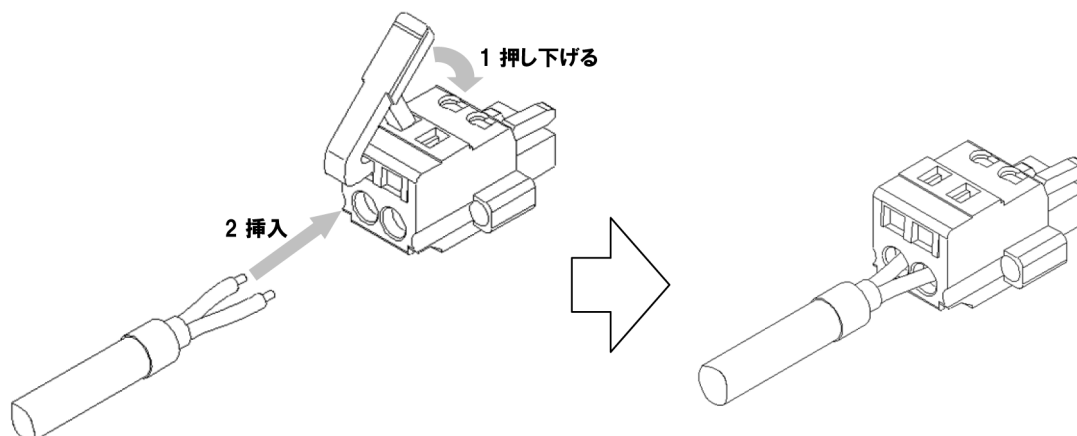
図 4-15 電源ケーブルの取り付け -2
