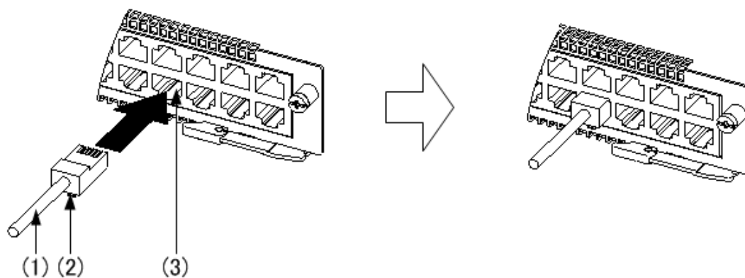
図 4-40 UTP ケーブルの取り付け（下側のポート）
