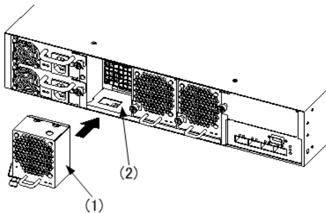
図 5-4 ファンユニットの取り付け -2
