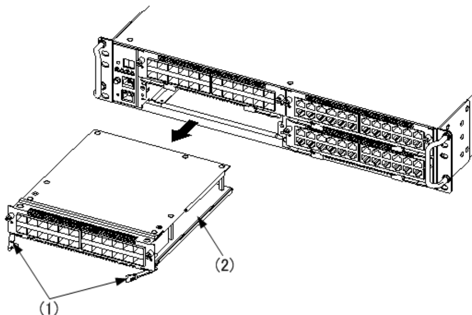
図 5-15 ネットワークインタフェース機構の取り外し -3
