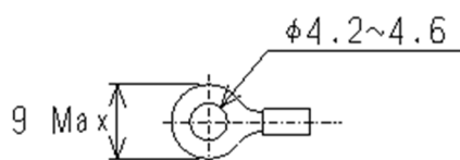
図 2-5 接地用ケーブルの端子
