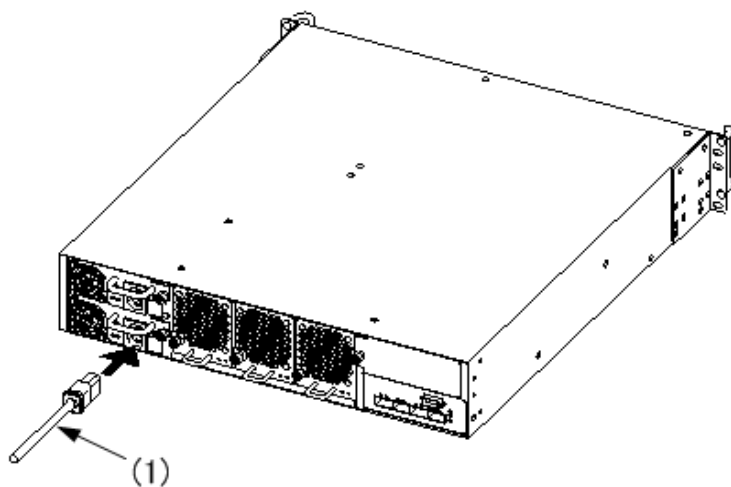
図 4-51 電源ケーブルの接続
