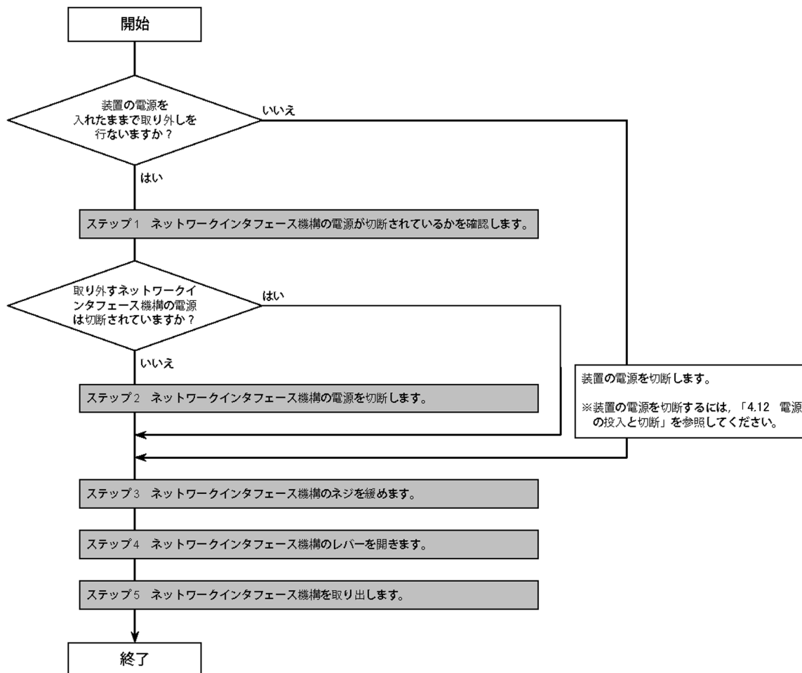
図 5-11 取り外しの操作の流れ
