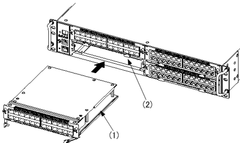
図 5-17 ネットワークインタフェース機構の取り付け -1
