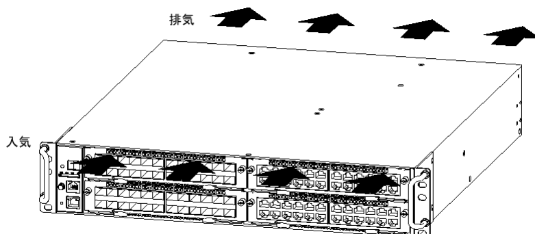
図 2-9 IP8800/S4630
