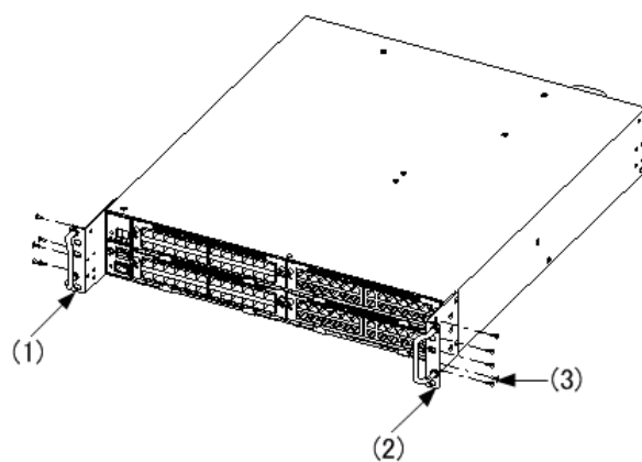
図 4-4 ラック取り付け金具の取り付け
