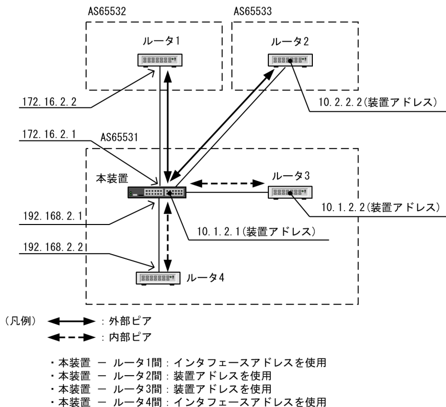
図 13-9 接続構成例
