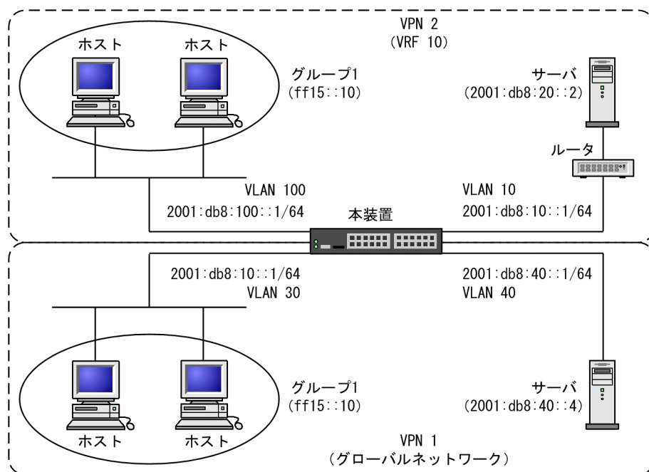
図 32-2 VRF での IPv6 PIM-SM 構成例
