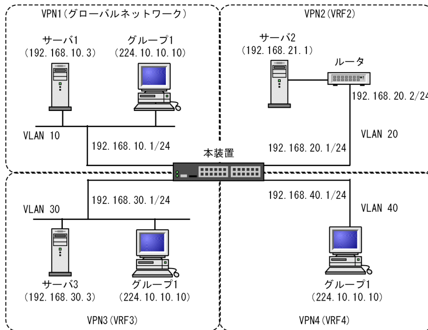
図 17-2 IPv4 マルチキャストエクストラネットの構成例
