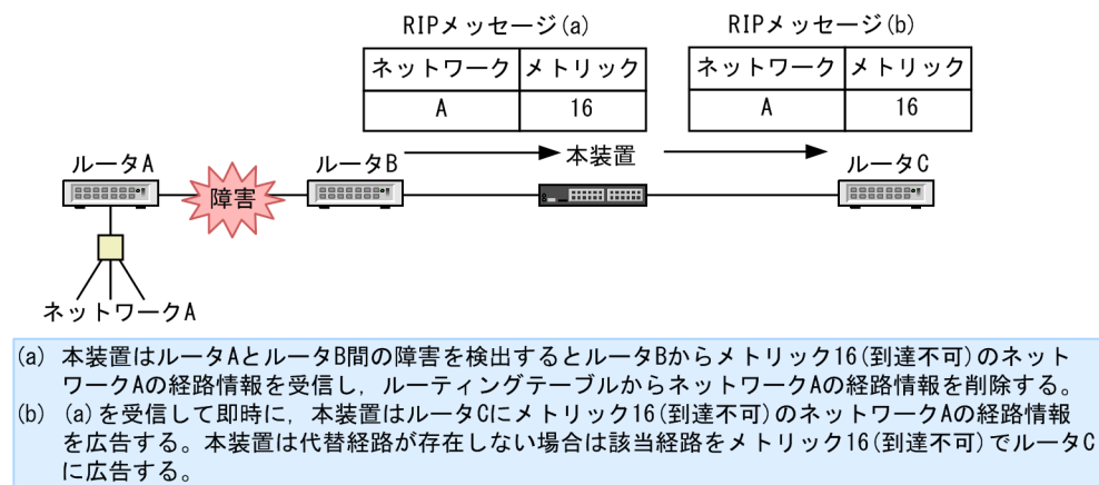
図 10-4 ルートポイズニング
