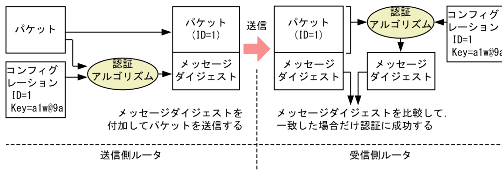
図 10-13 暗号認証のデータフロー
