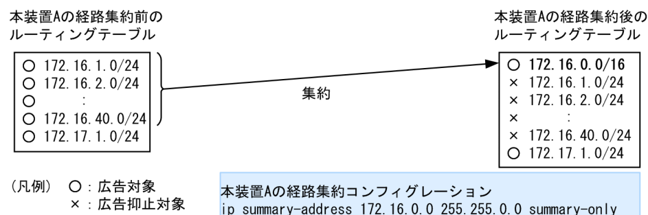
図 8-17 経路集約のコンフィグレーション例と経路集約前後の経路
