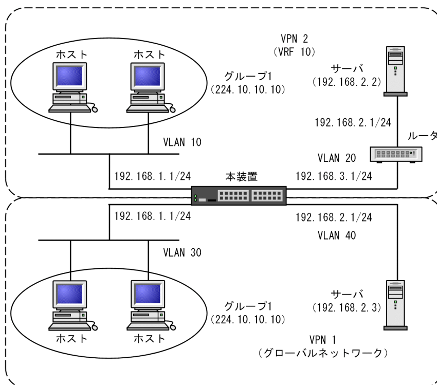
図 16-6 VRF での PIM-SSM 構成例 (IPv4 マルチキャストエクストラネット)
