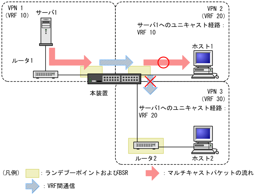
図 15-24 IPv4 マルチキャストエクストラネット使用時に装置内で VRF 中継を禁止している例
