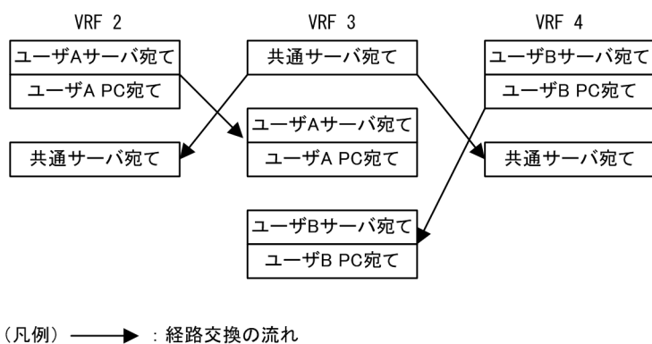
図 35-7 本装置の経路情報
