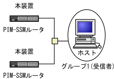
図 31-34 注意が必要な構成（複数ルータとホストの接続）
