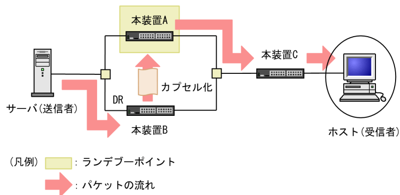
図 15-33 注意が必要な構成（複数ルータと送信者の接続）
