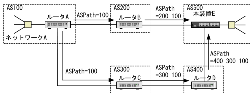
図 13-3 AS_PATH 属性による経路選択
