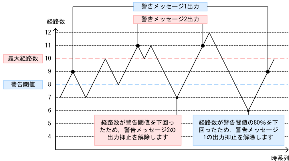
図 24-11 経路数と警告メッセージ出力の関係
