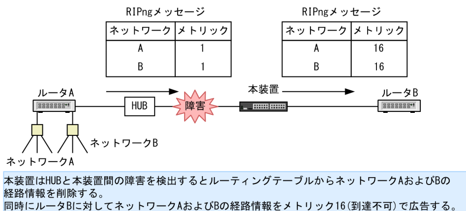
図 26-2 triggered update による経路情報の広告
