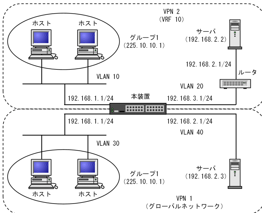
図 16-5 VRF での IGMP 構成例
