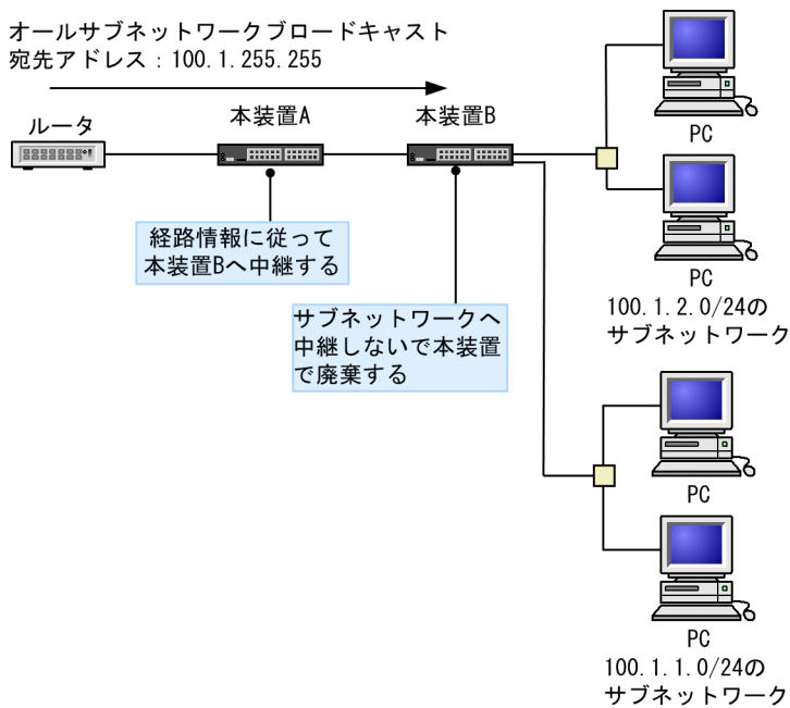
図 1-9 オールサブネットワークブロードキャスト
