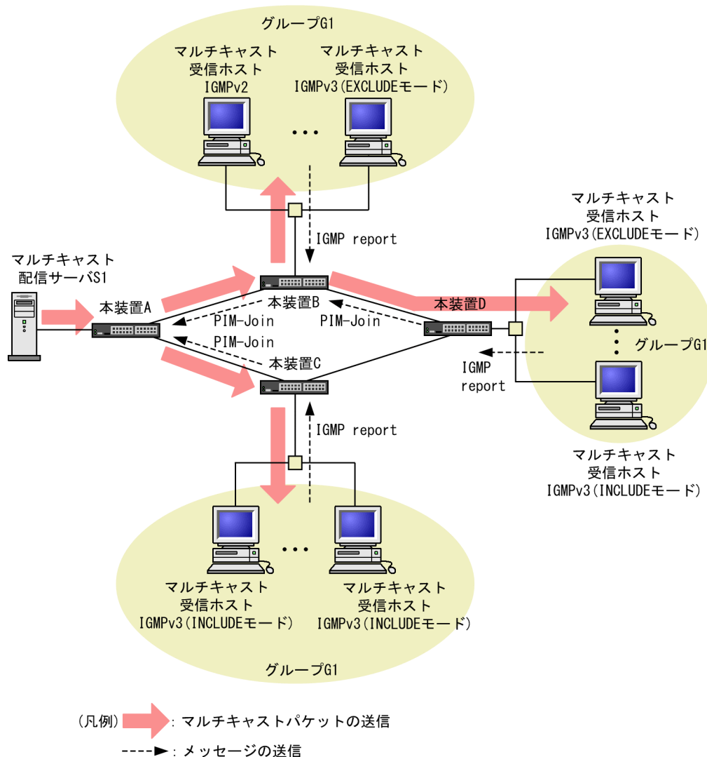
図 15-18 PIM-SSM の動作概要
