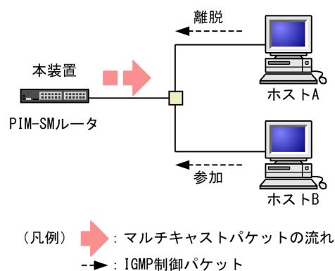
図 15-29 注意が必要な構成（ルータと複数ホストの接続）
