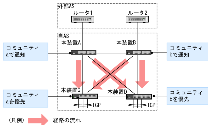
図 13-15 学習経路フィルタリングと COMMUNITIES 属性の使用例
