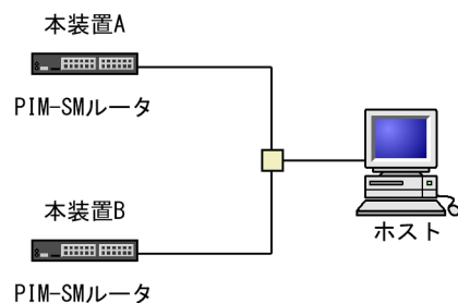
図 15-28 注意が必要な構成（複数ルータとホストの接続）
