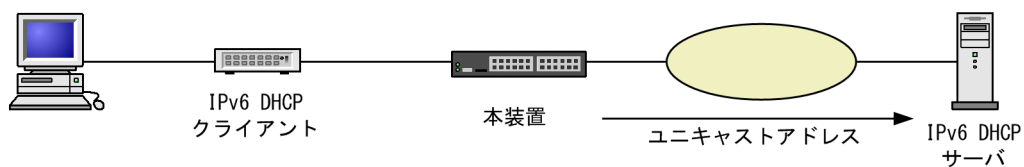
図 22-1 IPv6 DHCP リレーの接続構成
