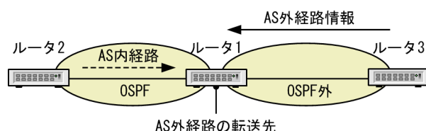
図 11-4 システム構成例（AS 境界ルータを目標とする場合）
