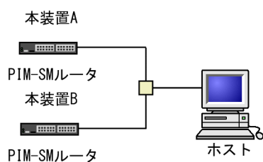
図 31-28 注意が必要な構成 (複数ルータとホストの接続)
