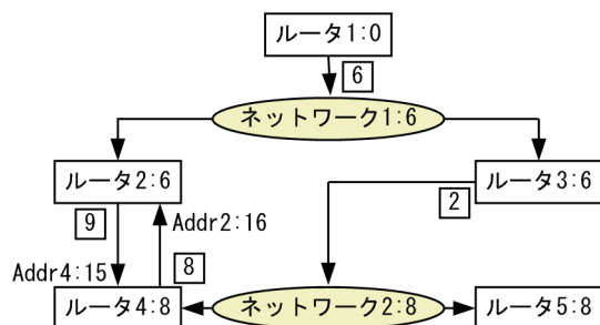
図 11-2 ルータ 1 を根とする最短木
