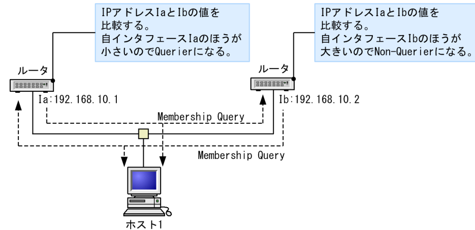
図 15-5 Querier と Non-Querier の決定
