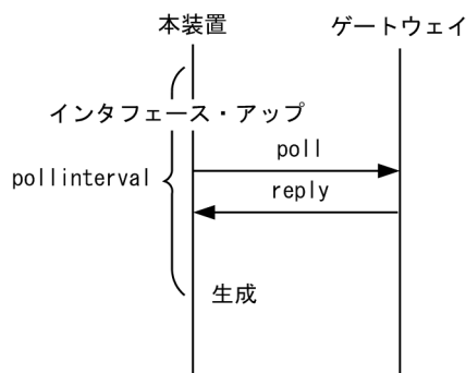
図 9-3 スタティック経路の動的監視による経路生成
