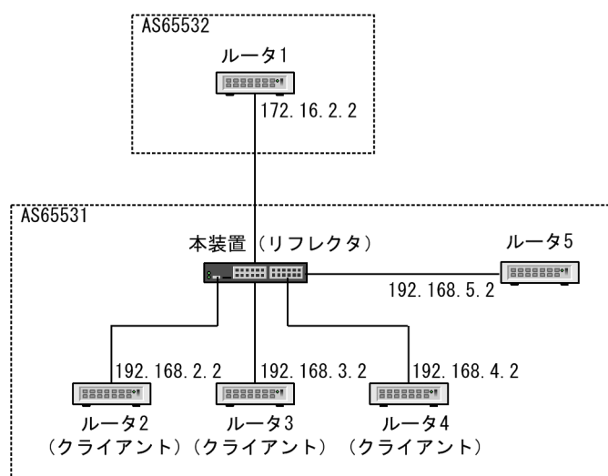
図 13-30 ルート・リフレクション構成例
