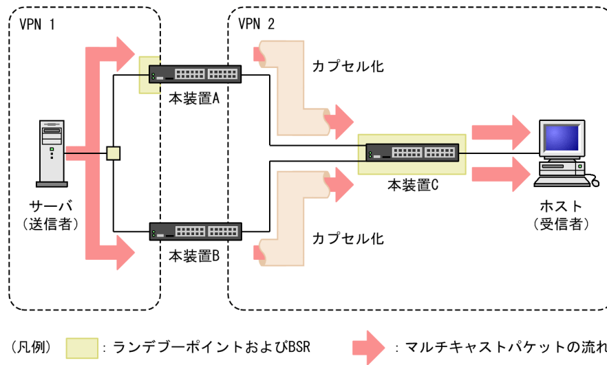
図 31-35 注意が必要な構成 (2 台以上の VRF 境界ルータで冗長構成を構築する場合)
