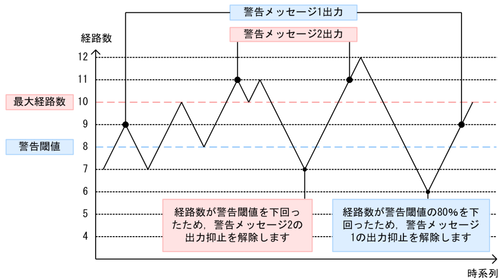
図 8-23 経路数と警告メッセージ出力の関係
