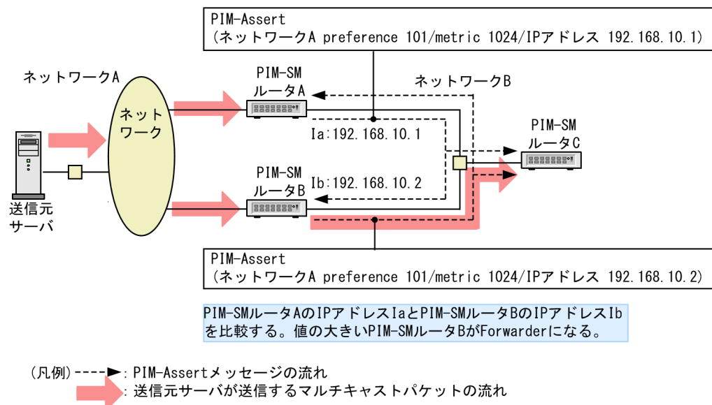
図 15-14 Forwarder の決定
