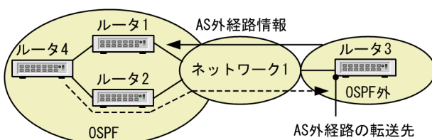
図 11-5 システム構成例（フォワーディングアドレスを目標とする場合）
