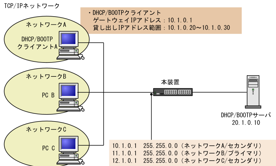
図 5-2 マルチホーム構成
