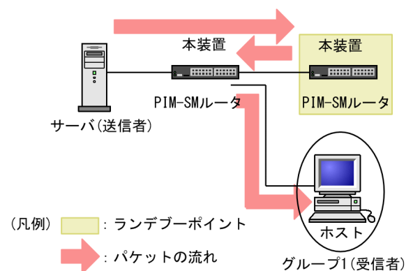
図 15-34 不適応な構成（送信者とランデブーポイントの間に受信者が存在する場合）
