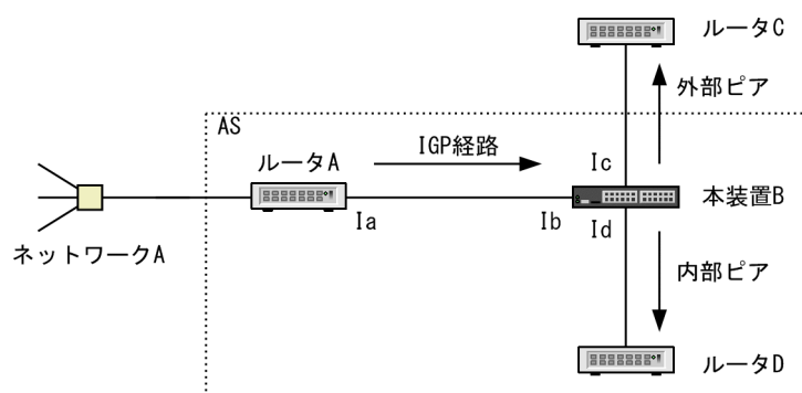
図 13-8 IGP 経路を BGP4 で広告する場合に通知する経路情報の NEXT_HOP 属性の設定例
