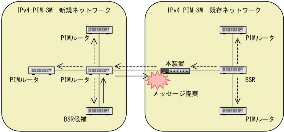
図 15-17 ブートストラップメッセージ受信抑止機能の動作
