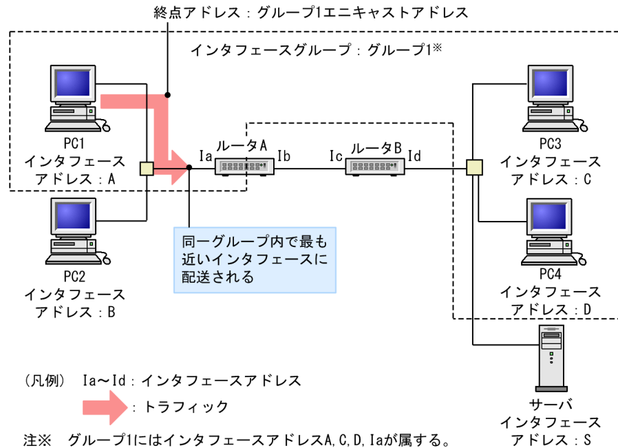
図 18-2 エニキャストアドレス通信
