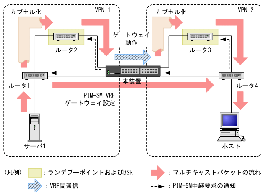
図 15-23 PIM-SM VRF ゲートウェイの動作概要
