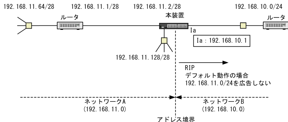
図 10-12 直結経路を広告しない構成例
