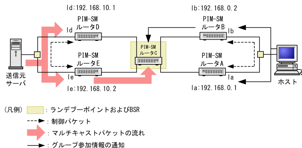
図 15-15 DR の動作
