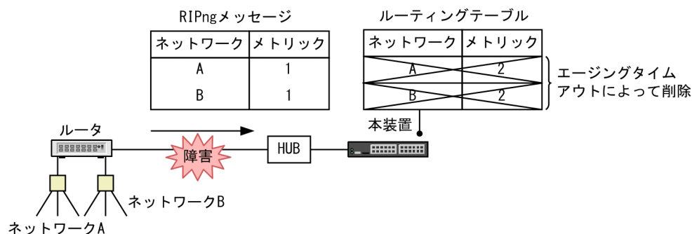
図 26-7 エージングタイムアウトによる経路情報の削除
