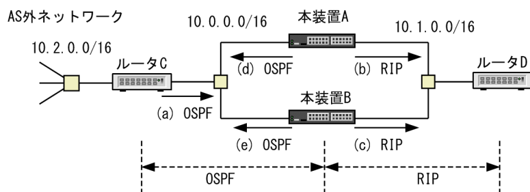
図 8-8 ネットワーク構成例
