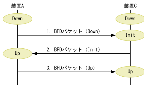
図 34-2 BFD の状態遷移
