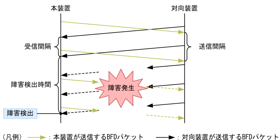
図 34-4 BFD セッションでの障害検出
