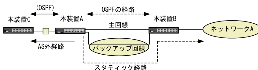
図 11-3 バックアップ回線を使用した構成での AS 外経路の導入例
