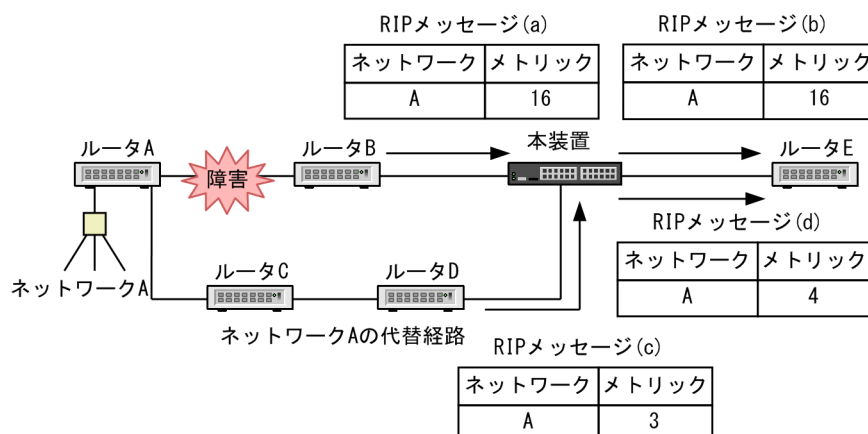
図 10-5 ルートポイズニング期間中の再学習
