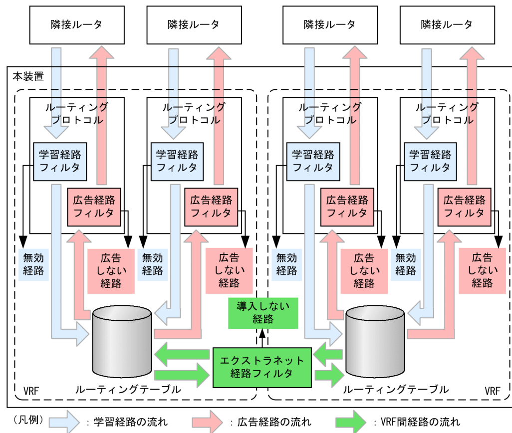
図 14-2 エクストラネットの経路フィルタリングの概念図
