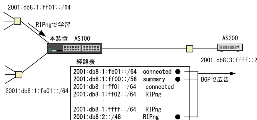
図 24-8 集約経路を BGP4+で広告する構成
