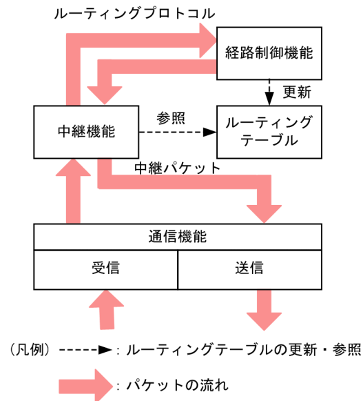
図 18-20 IPv6 ルーティング機能の概要
