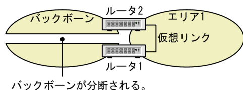
図 12-5 バックボーン分断に対する予備経路
