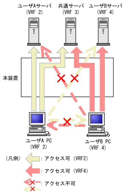
図 35-6 経路交換によるエクストラネット
