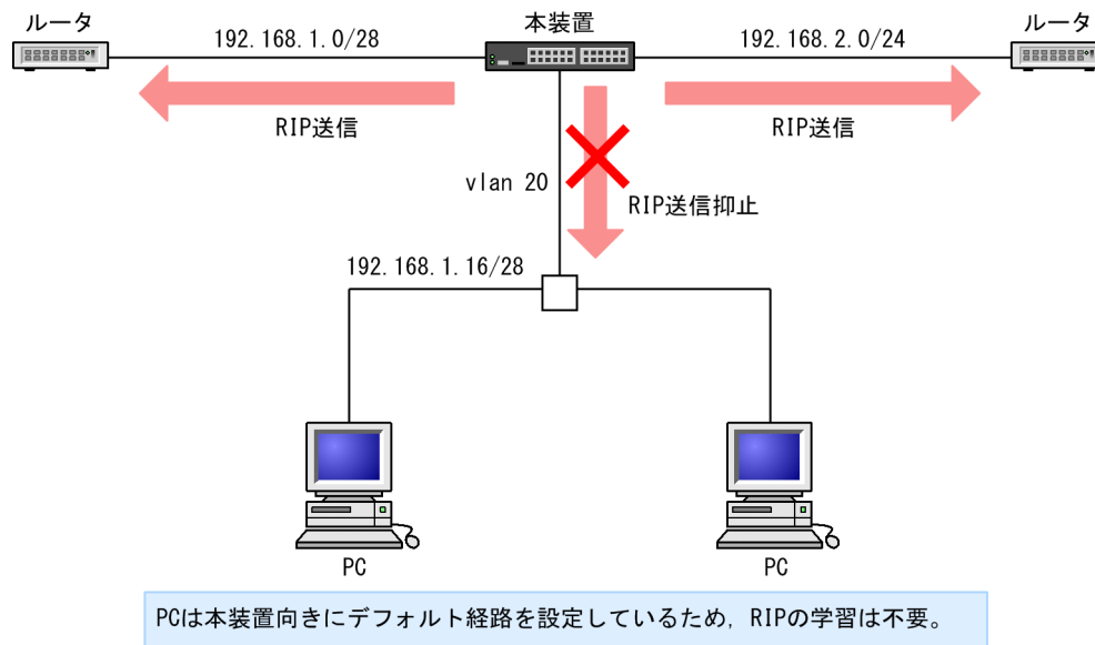
図 10-14 RIP パケットの送信抑止
