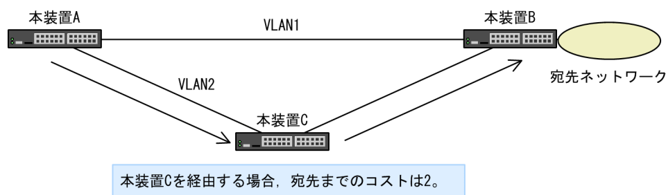
図 11-7 マルチパスの構成
