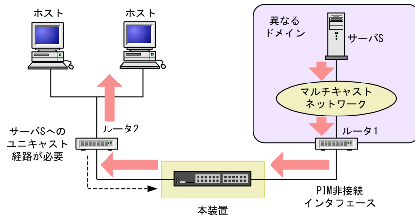
図 31-30 注意が必要な構成 (PIM 非接続インタフェース経由の中継)
