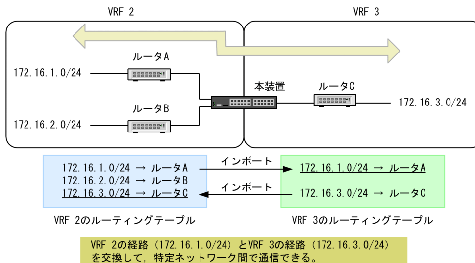
図 8-24 VRF 間の経路交換
