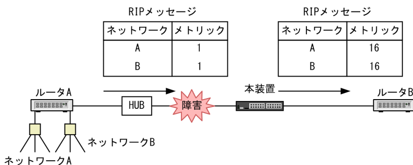
図 10-2 triggered update による経路情報の広告
