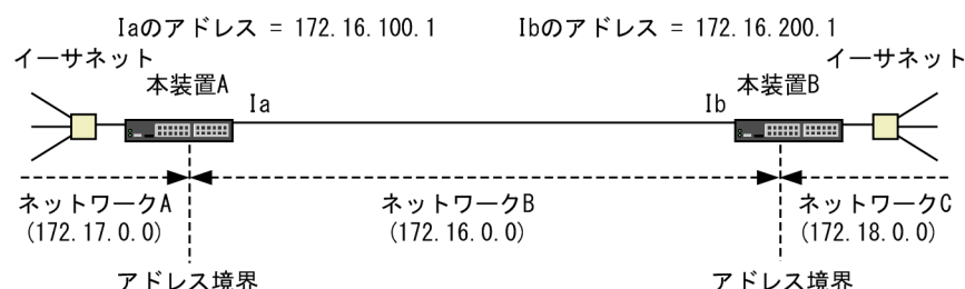
図 8-11 通常のアドレス境界設計例
