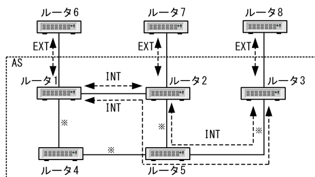
図 29-1 内部ピアと外部ピア
