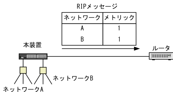
図 10-1 周期的な経路情報広告
