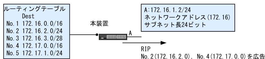
図 10-11 RIP で広告するナチュラルマスク経路およびサブネットマスク経路情報
