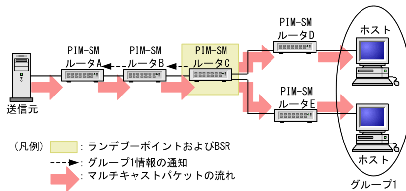
図 15-11 ランデブーポイント経由のマルチキャストパケット通信（デカプセル化）
