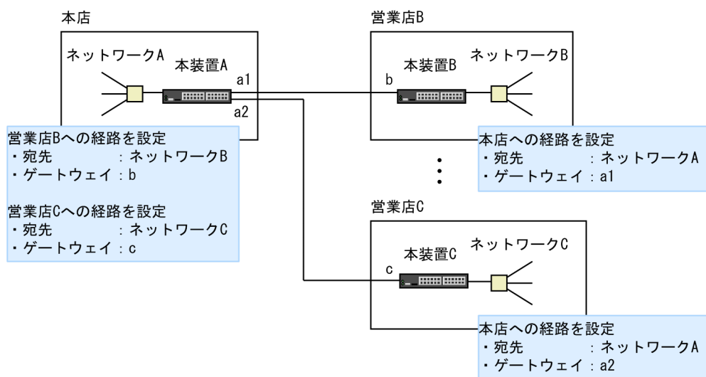
図 9-1 スタティックルーティングのネットワーク構成例
