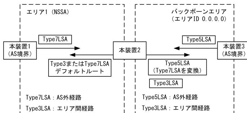
図 12-2 NSSA とバックボーンの間での経路交換
