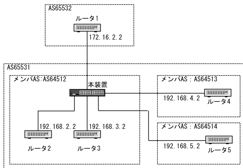
図 13-31 コンフェデレーション構成例
