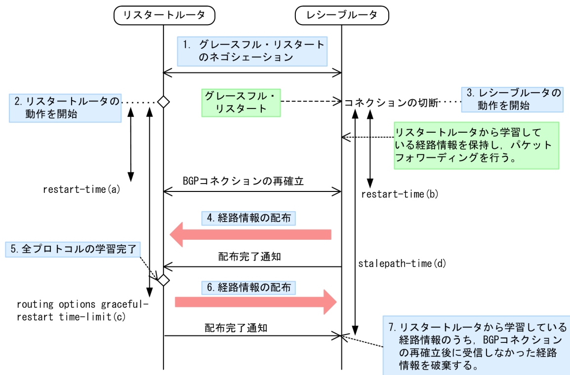
図 13-29 グレースフル・リスタートのシーケンス
