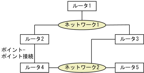
図 11-1 ネットワーク構成例
