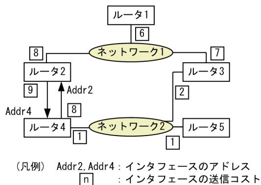
図 27-2 トポロジとコストの設定例
