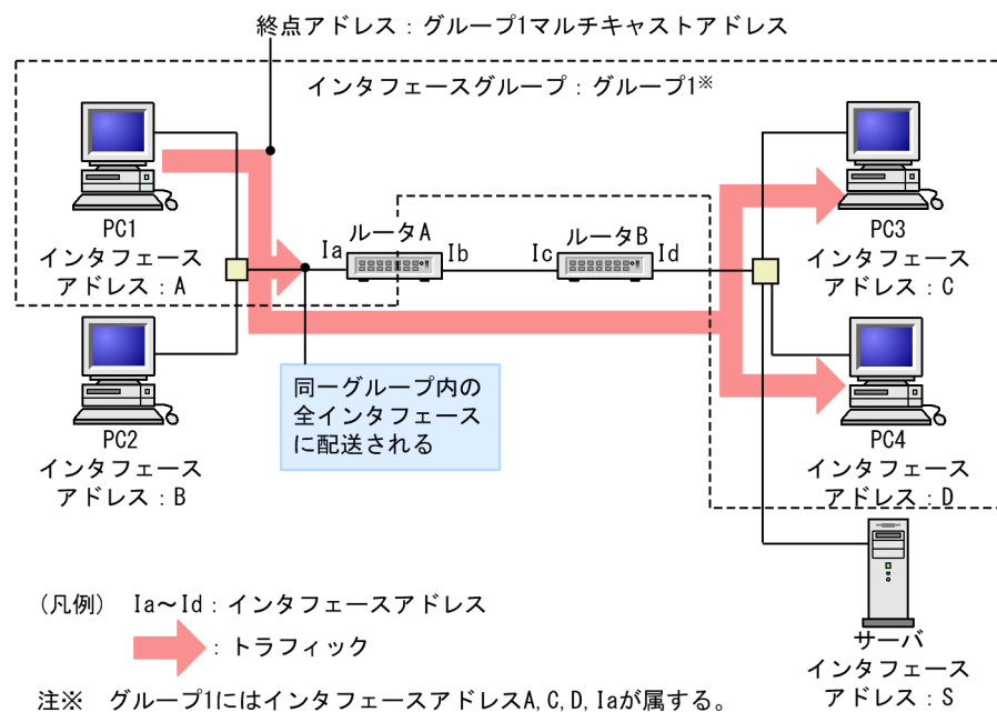
図 18-3 マルチキャストアドレス通信
