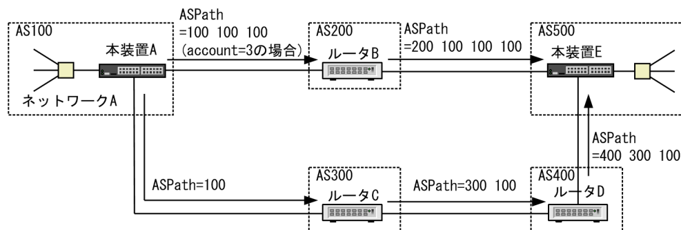
図 13-4 set as-path prepend count コマンドの使用例
