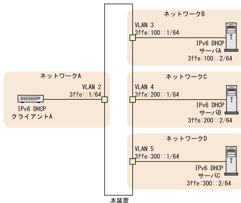
図 22-3 1 台の IPv6 DHCP リレーを経由するユニキャスト送信時の構成
