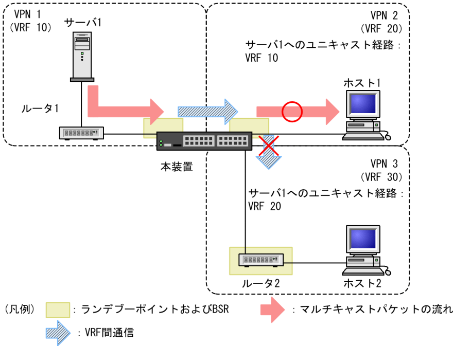
図 31-23 IPv6 マルチキャストエクストラネット使用時に装置内で VRF 中継を禁止している例
