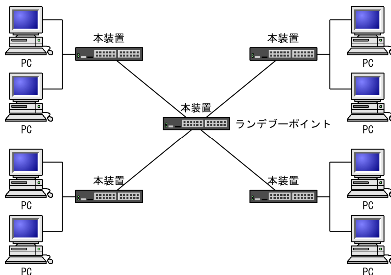
図 15-26 PIM-SM を使用する構成図
