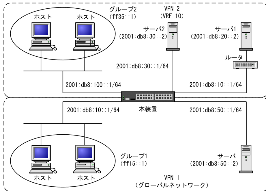
図 32-3 VRF での IPv6 PIM-SSM 構成例
