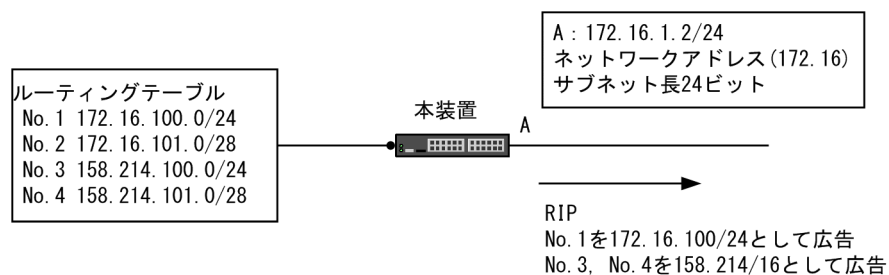
図 10-6 RIP-1 使用時の広告経路自動集約化
