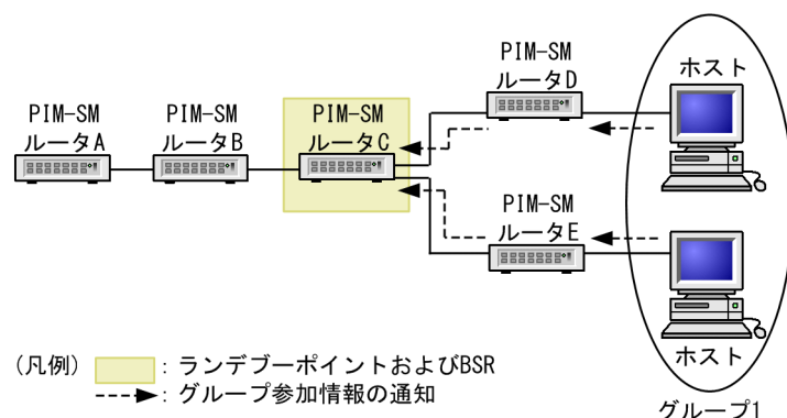
図 15-9 ランデブーポイントへのグループ参加情報の通知
