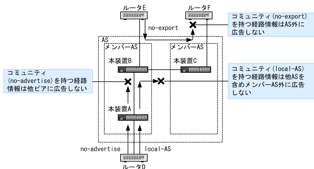
図 13-27 COMMUNITIES 属性を持つ経路情報の広告範囲
