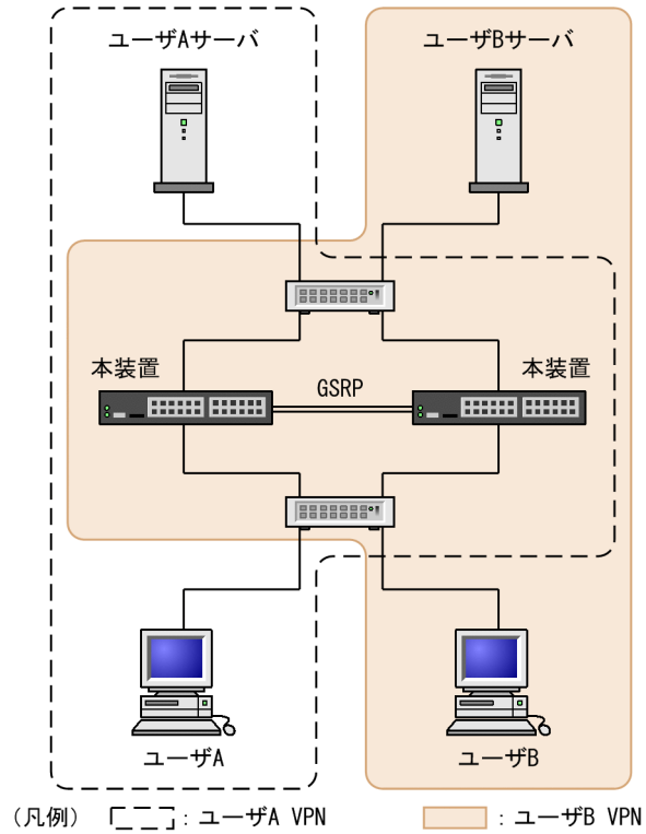
図 35-8 GSRP を使用したネットワーク・パーティション
