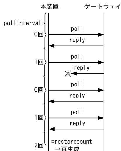
図 9-5 スタティック経路の動的監視による経路再生成 (restorecount =2 の場合)
