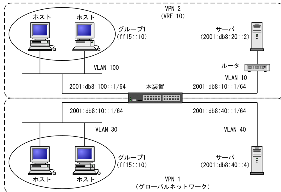
図 32-5 VRF での PIM-SSM 構成例 (IPv6 マルチキャストエクストラネット)
