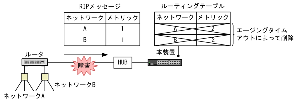
図 10-9 エージングタイムアウトによる経路情報の削除
