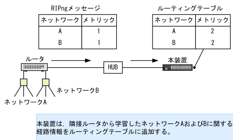
図 26-6 レスポンスパケット受信による経路情報の生成
