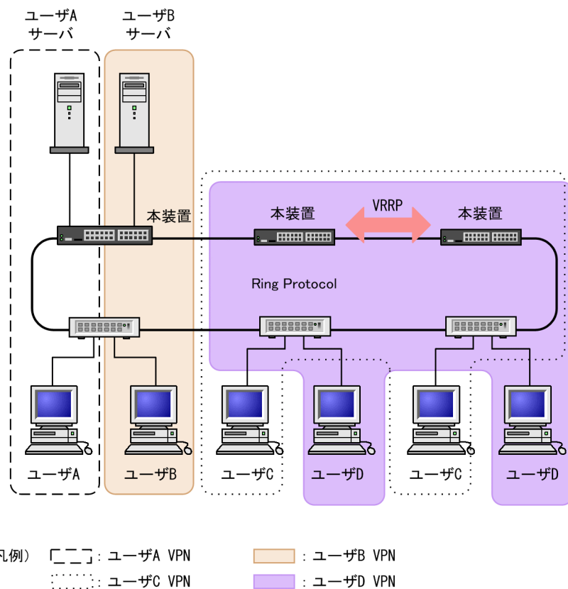
図 35-4 レイヤ 3 集約装置の増設
