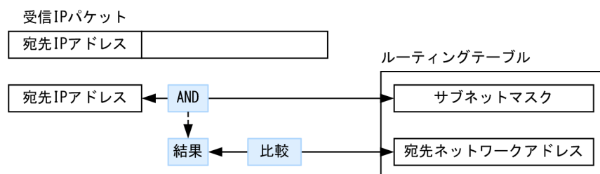
図 1-4 ルーティングテーブルの検索
