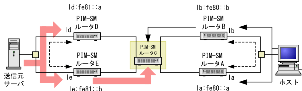
図 31-15 DR の動作
