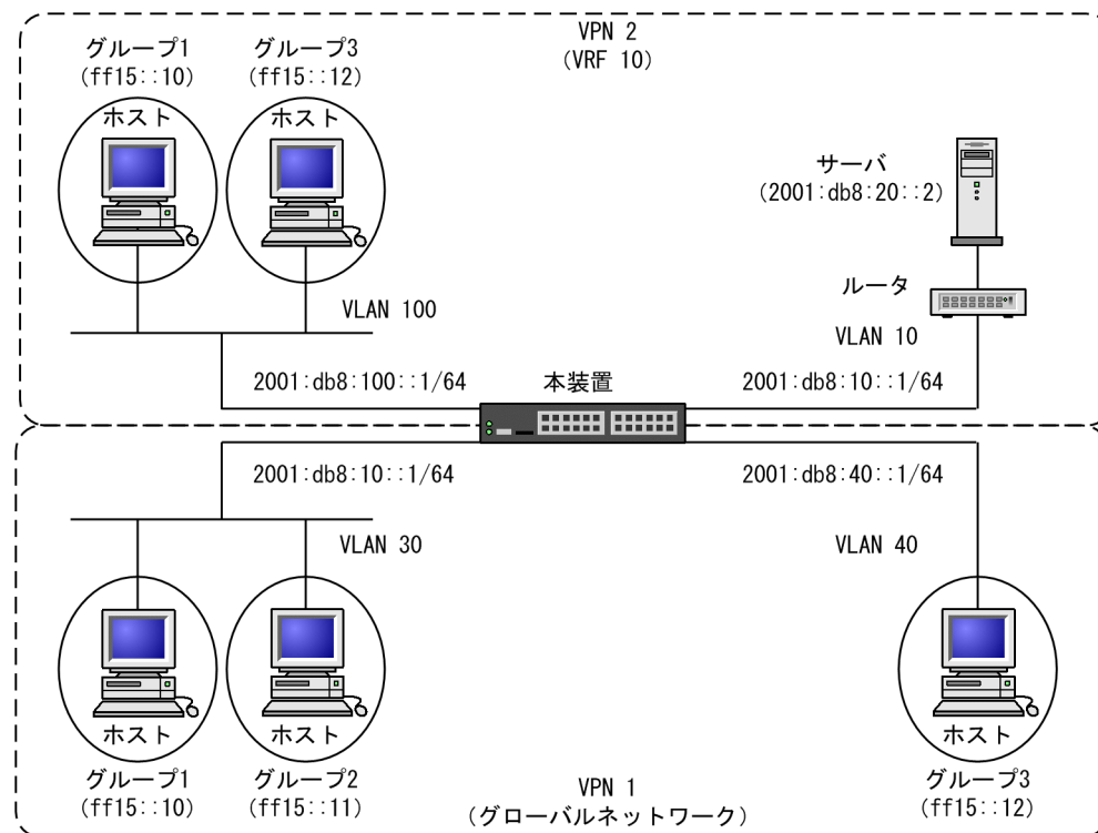
図 32-6 VRF での PIM-SM 構成例 (PIM-SM VRF ゲートウェイ)
