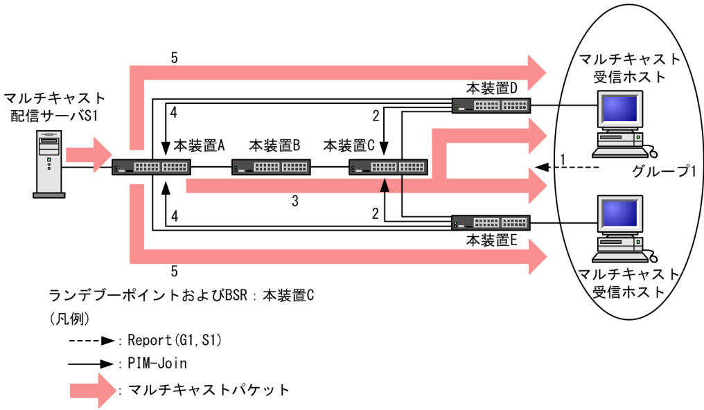
図 15-20 IGMPv3 使用時の IPv4 PIM-SM 動作概要
