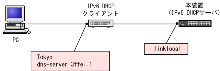
図 23-3 クライアントにオプション情報を配布する構成
