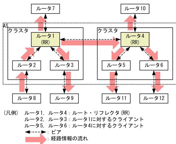
図 13-23 クラスタ内に一つのルート・リフレクタを置く例
