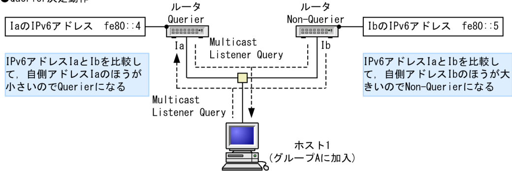
図 31-4 Querier と Non-Querier の決定
