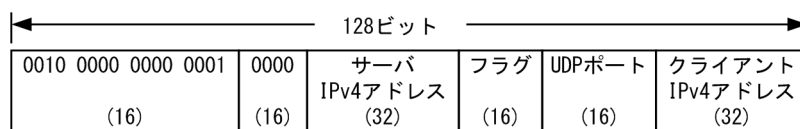
図 18-17 Teredo IPv6 アドレス
