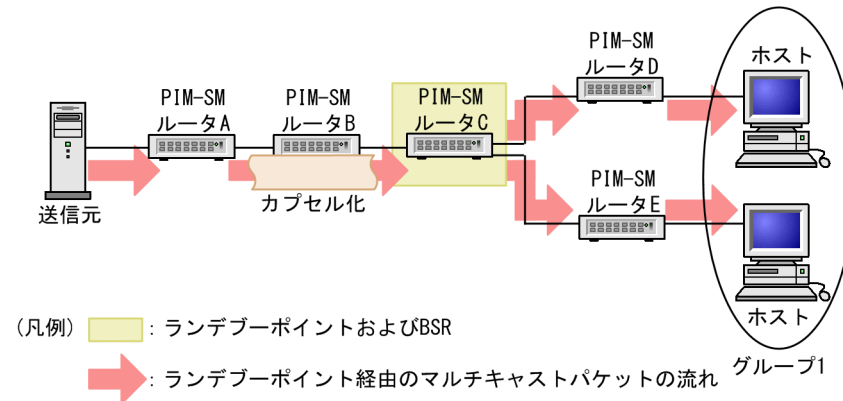
図 15-10 ランデブーポイント経由のマルチキャストパケット通信（カプセル化）
