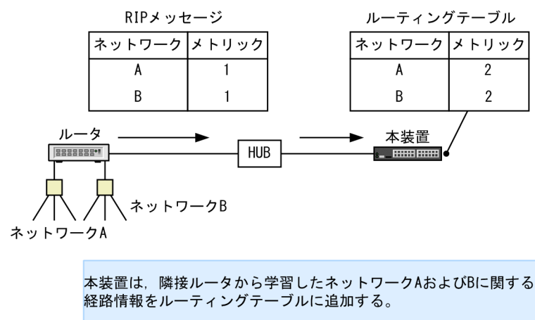
図 10-8 レスポンスパケット受信による経路情報の生成
