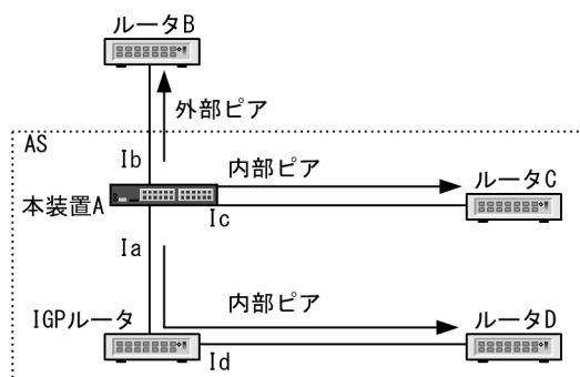
図 13-7 BGP4 ピアから学習した経路を広告する場合に通知する経路情報の NEXT_HOP 属性の設定例
