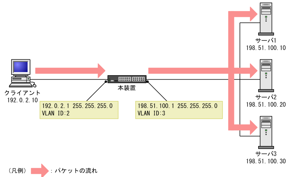
図 7-2 転送先がサブネットブロードキャストアドレスの場合
