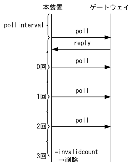
図 9-4 スタティック経路の動的監視による経路削除 (invalidcount=3 の場合)
