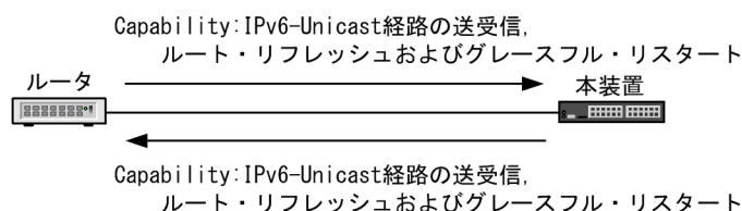
図 29-14 ネゴシエーションの動作概念
