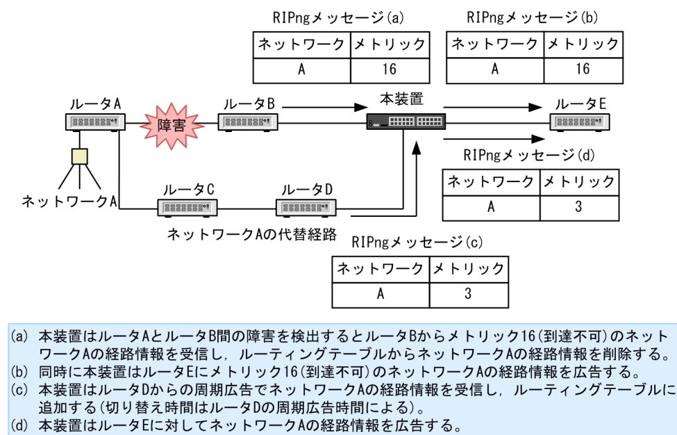
図 26-5 ルートポイズニング期間中の再学習
