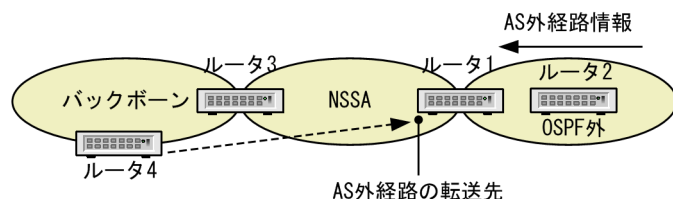
図 11-6 システム構成例（任意のインタフェースを目標とする場合）
