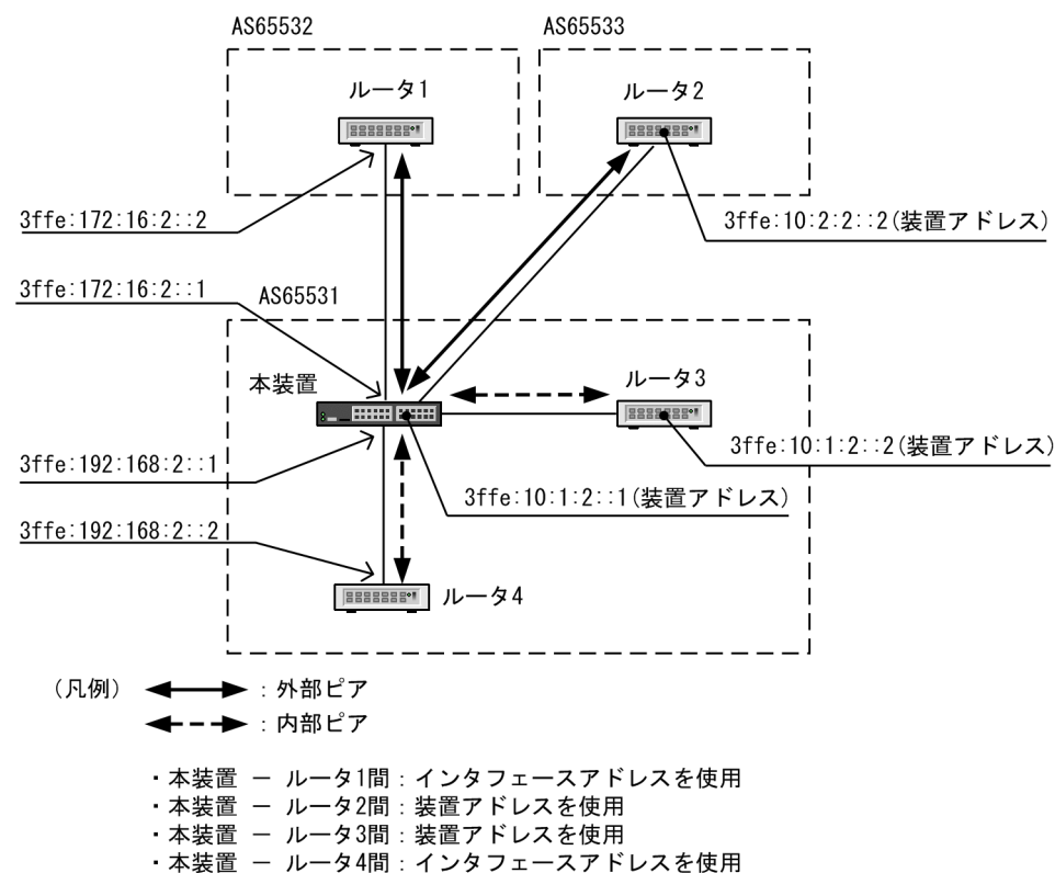
図 29-9 接続構成例
