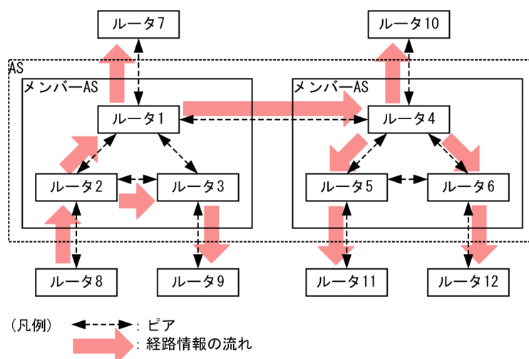
図 13-25 コンフェデレーション構成での経路情報の流れ
