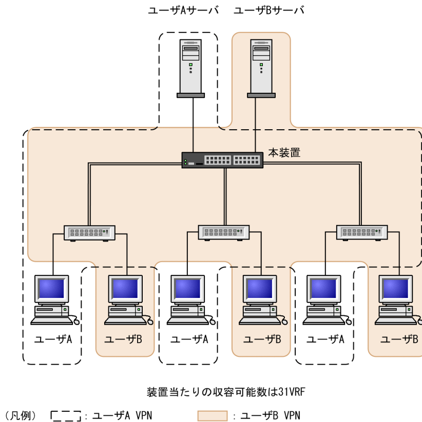
図 35-5 レイヤ 2 プロトコルを使用しない構築
