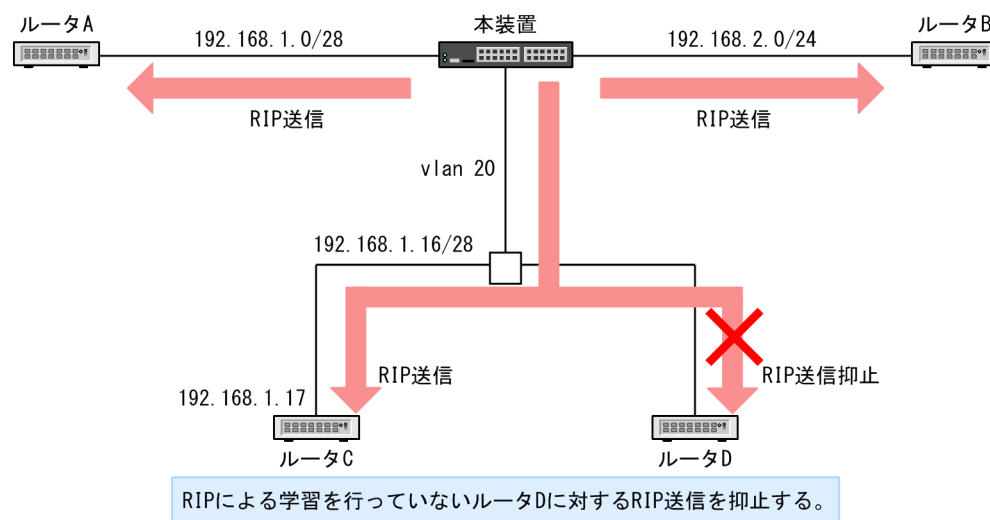
図 10-15 RIP パケット送信相手の限定
