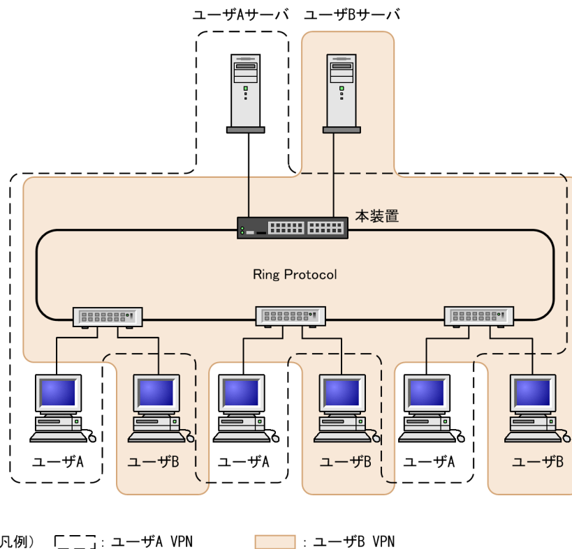
図 35-3 Ring Protocol を使用したネットワーク・パーティション
