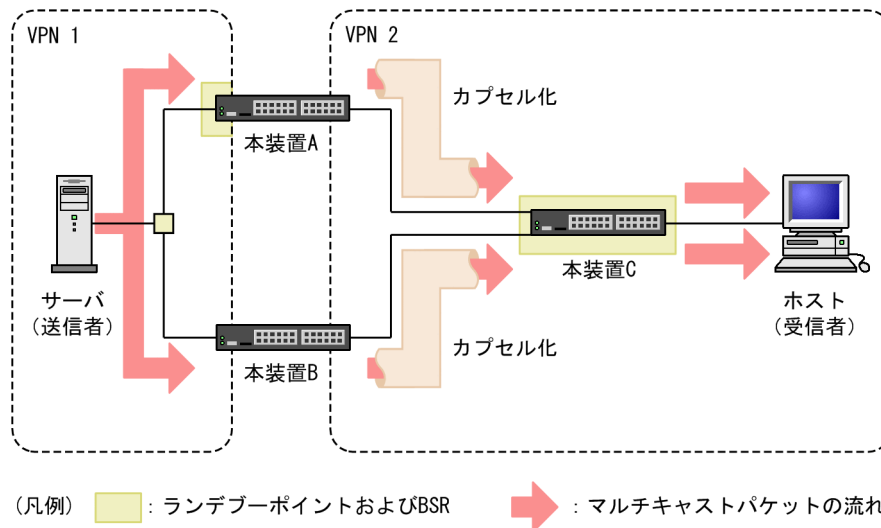
図 15-36 注意が必要な構成（2 台以上の VRF 境界ルータで冗長構成を構築する場合）
