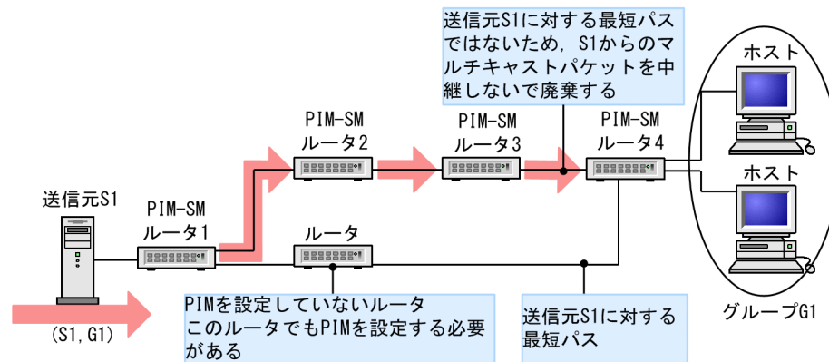
図 15-16 冗長経路時の注意
