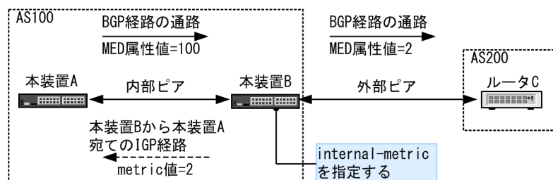
図 13-6 set metric-type internal の使用例
