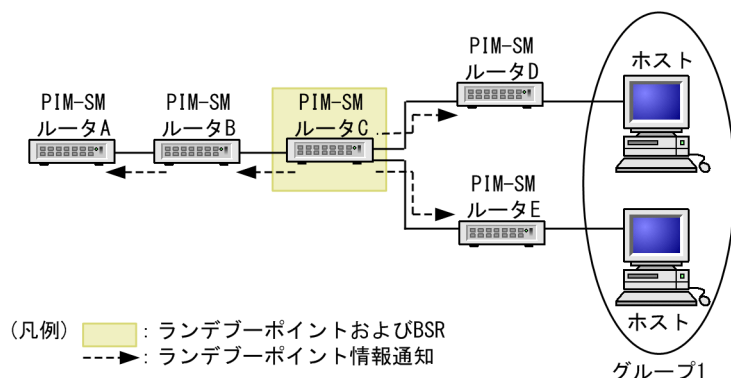
図 15-8 ランデブーポイントおよびブートストラップルータ (BSR) の役割
