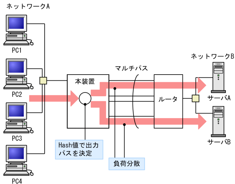
図 8-12 マルチパスを使用した負荷分散（隣接ルータが単一の場合）
