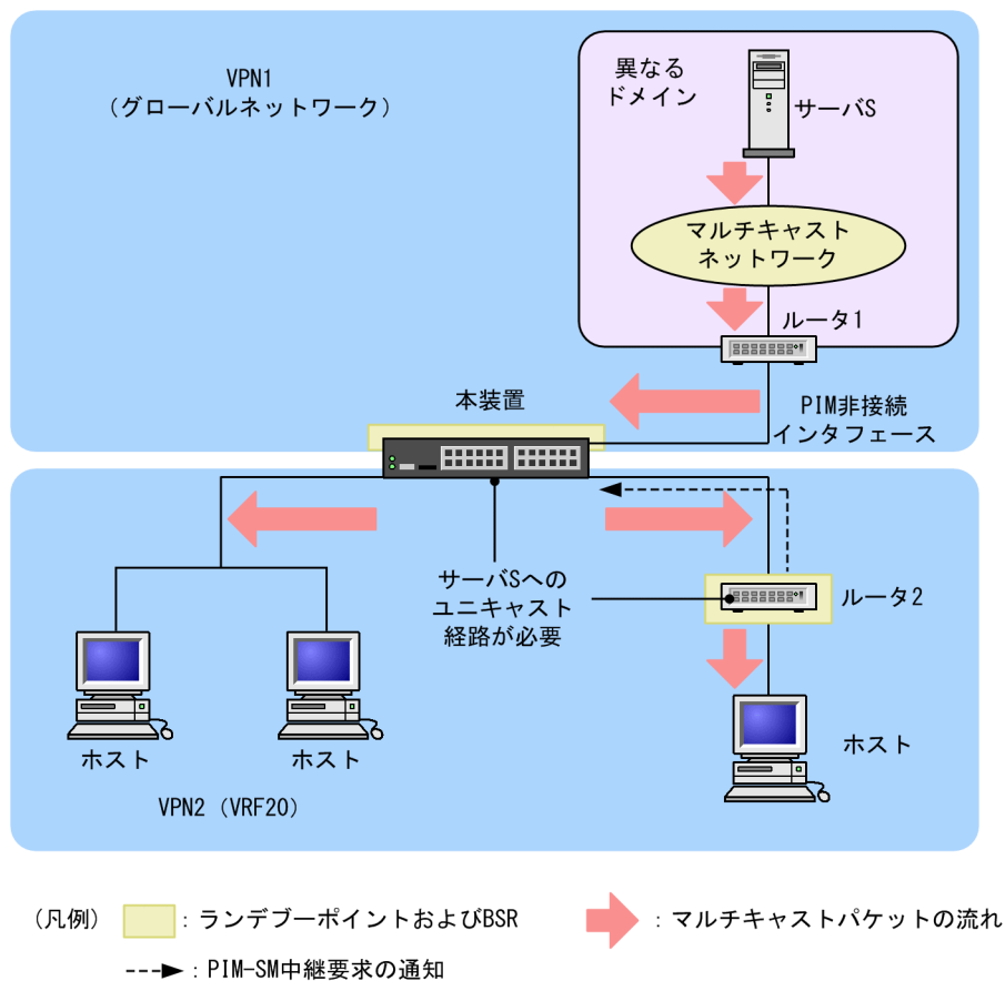
図 31-31 注意が必要な構成（エクストラネットでの PIM 非接続インタフェース経由の中継）
