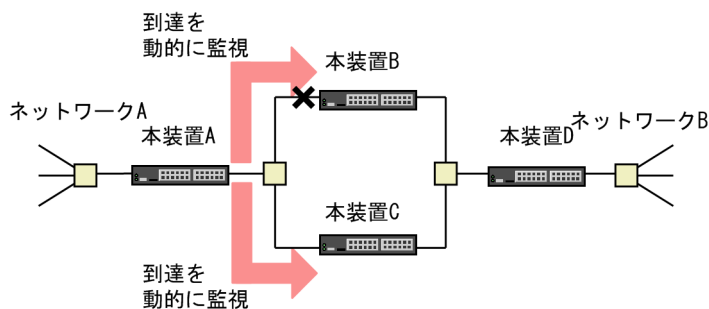
図 9-2 スタティック経路の動的監視の例
