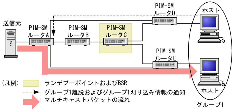
図 15-13 マルチキャスト配送ツリーの刈り込み
