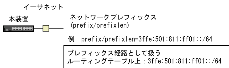
図 24-3 直結経路の取り扱い（ブロードキャスト型の場合）
