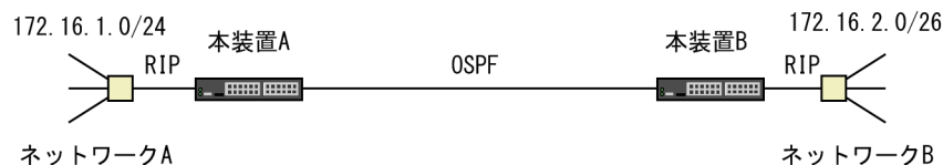
図 8-2 異なるサブネットマスク長のサブネット間の接続
