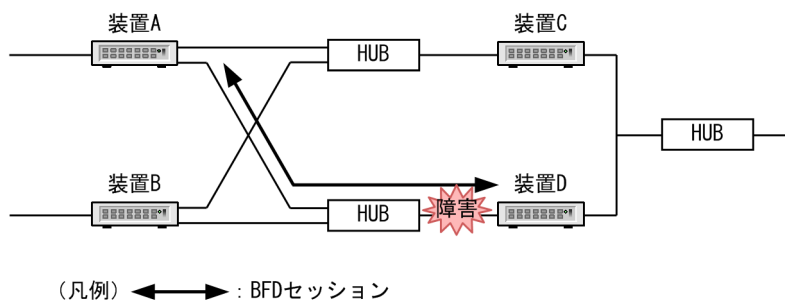
図 34-3 BFD セッションでの障害発生
