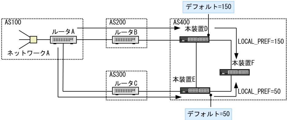
図 13-2 LOCAL_PREF 属性による経路選択
