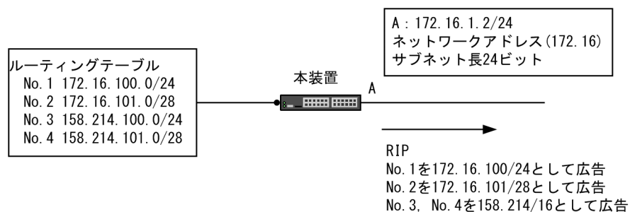
図 10-7 RIP-2 使用時の広告経路自動集約化
