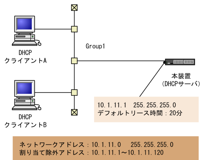
図 6-1 クライアントーサーバ構成（動的 IP アドレス配布時）
