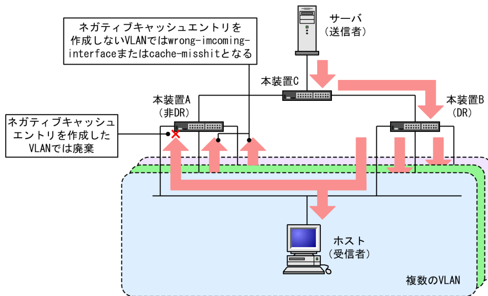
図 15-31 複数 VLAN 設定時のマルチキャストパケット廃棄処理
