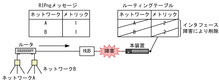
図 26-8 インタフェース障害による経路情報の削除
