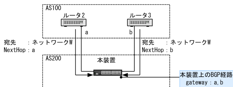
図 13-17 複数のピアから学習した BGP4 経路マルチパス化の概念
