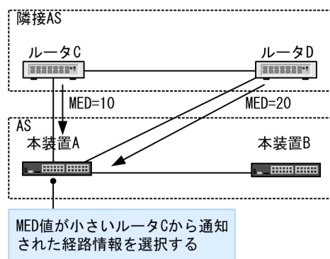
図 29-5 MED 属性による経路選択
