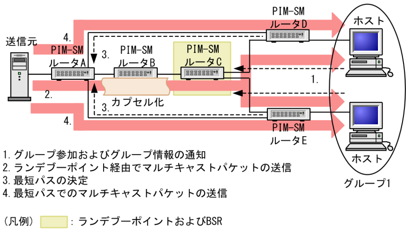
図 15-7 PIM-SM の動作概要
