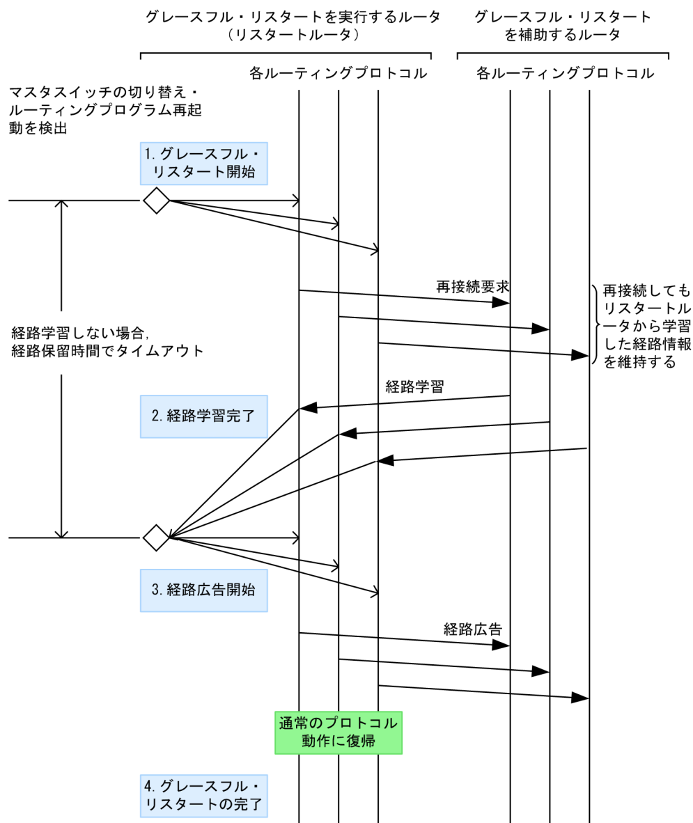
図 8-22 グレースフル・リスタート手順
