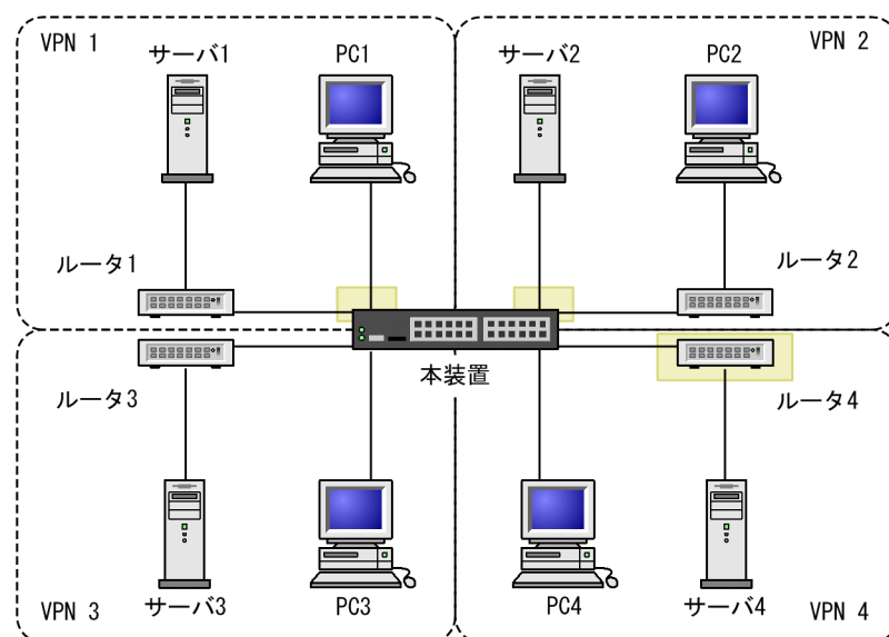
図 31-20 VRF での IPv6 マルチキャスト
