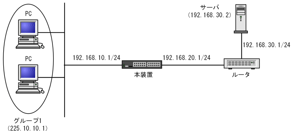
図 16-1 PIM-SM 構成例
