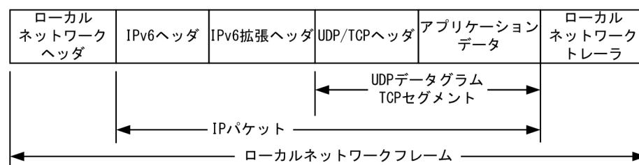
図 18-21 IPv6 パケットフォーマット
