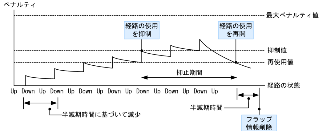
図 13-22 ルート・フラップ・ダンプニングの動作概念
