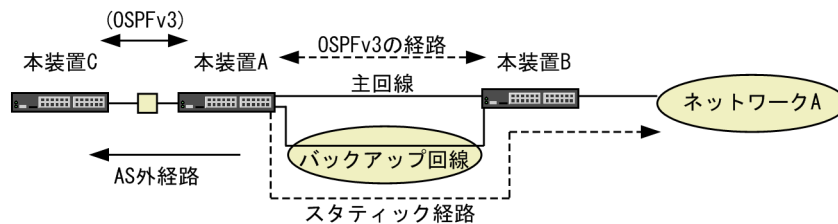
図 27-4 バックアップ回線を使用した構成での AS 外経路の導入例
