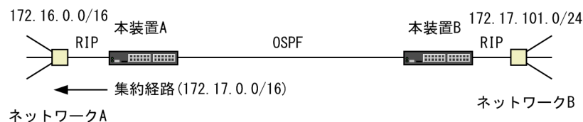
図 8-7 集約経路の広告の例
