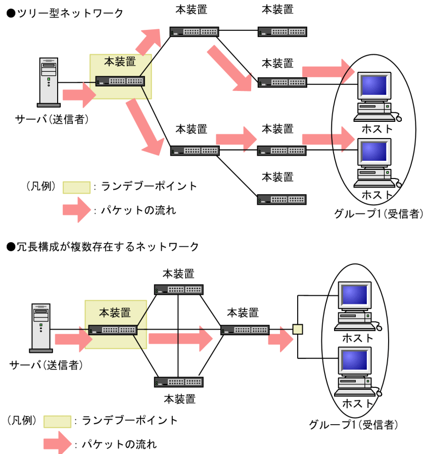
図 15-32 PIM-SM 推奨ネットワーク構成
