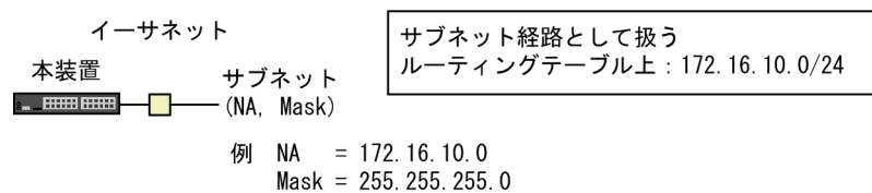
図 8-10 直結経路の取り扱い
