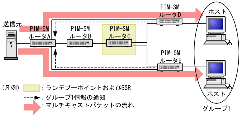
図 15-12 最短パスのマルチキャストパケット通信
