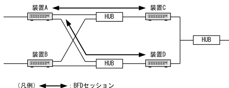
図 34-1 BFD の基本動作
