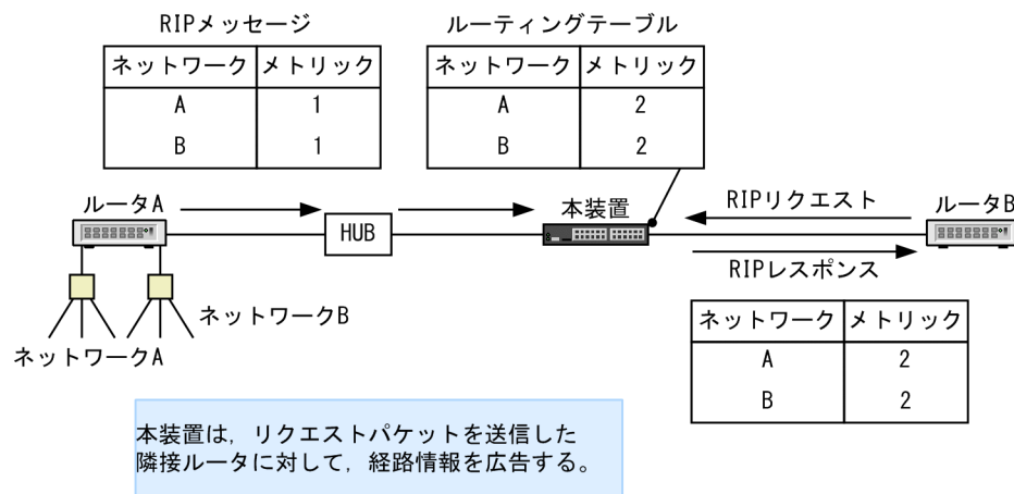
図 10-3 リクエストパケット受信による経路情報の広告
