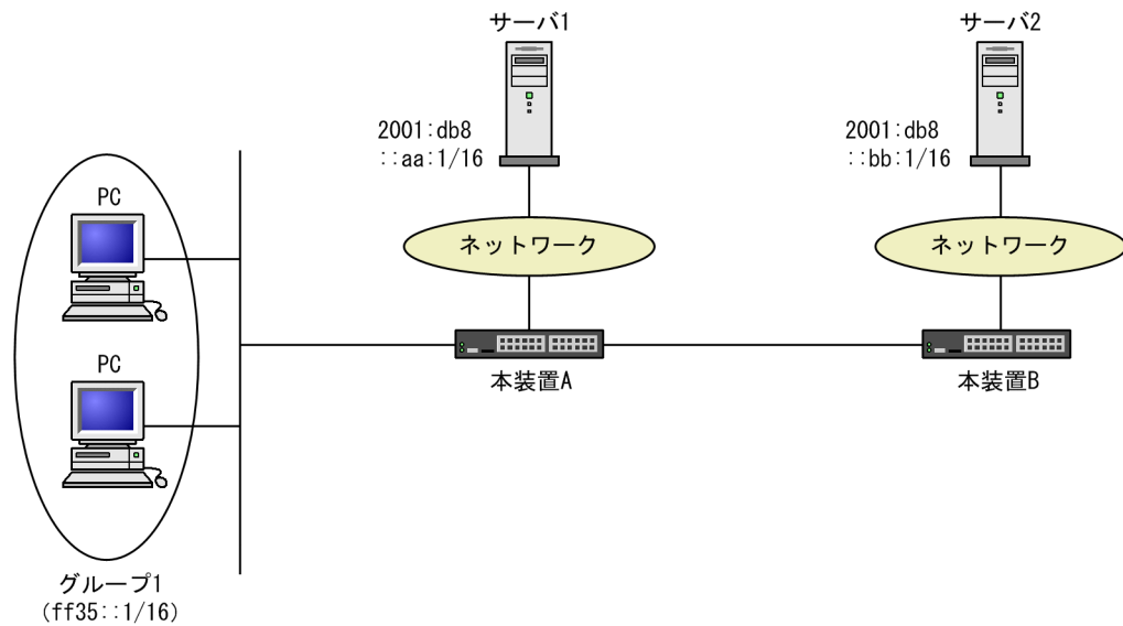
図 32-1 PIM-SSM 構成例
