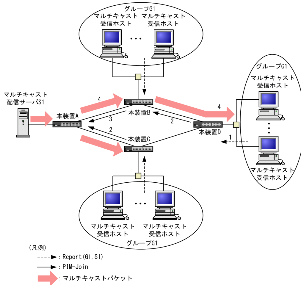
図 15-19 IGMPv3 使用時の IPv4 PIM-SSM 動作概要
