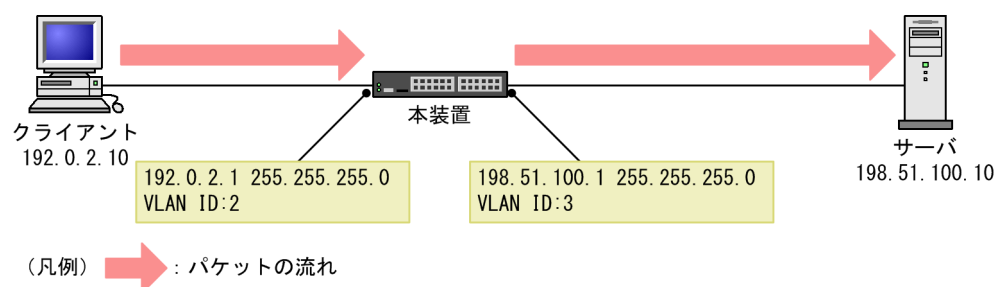
図 7-1 転送先がユニキャストアドレスの場合
