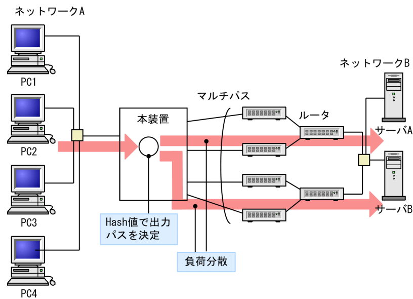
図 8-13 マルチパスを使用した負荷分散（隣接ルータが複数の場合）
