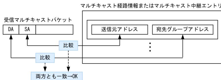
図 15-6 マルチキャスト経路情報またはマルチキャスト中継エントリの検索方法
