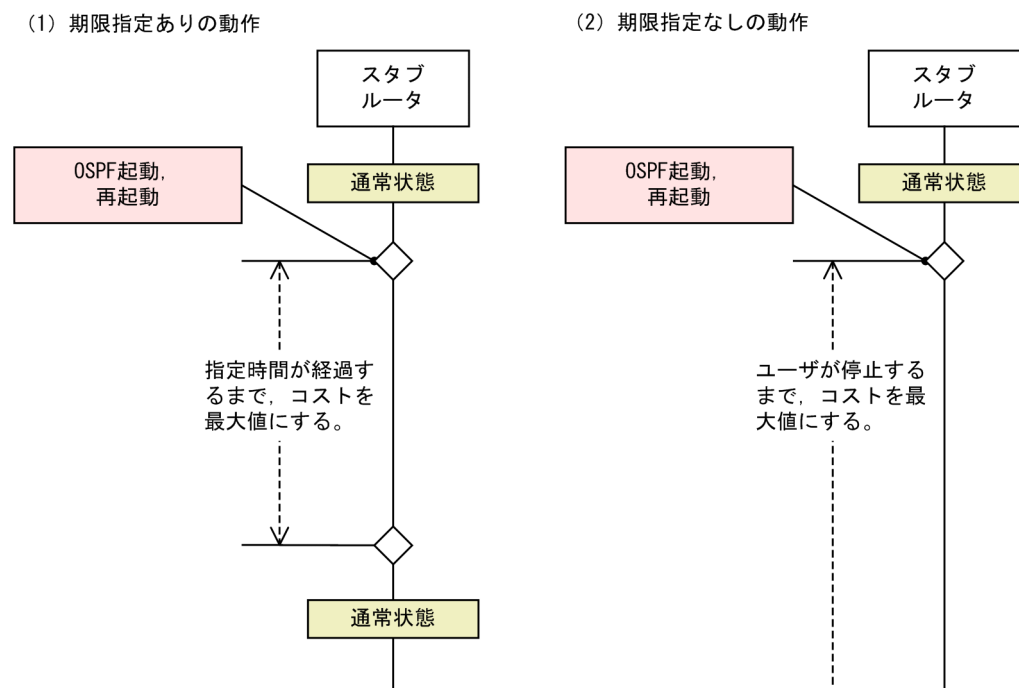
図 12-8 スタブルータの動作
