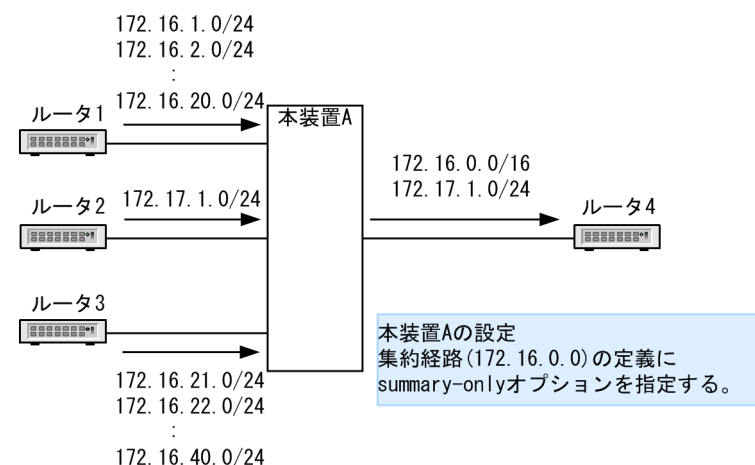
図 8-16 集約元経路の広告抑止の適用例
