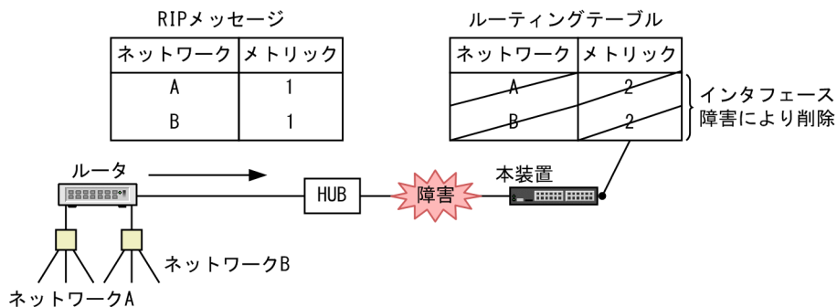
図 10-10 インタフェース障害による経路情報の削除
