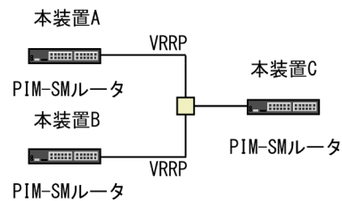
図 31-29 注意が必要な構成 (VRRP を設定した場合)
