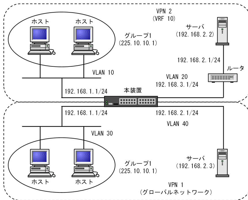
図 16-3 VRF での IPv4 PIM-SM 構成例
