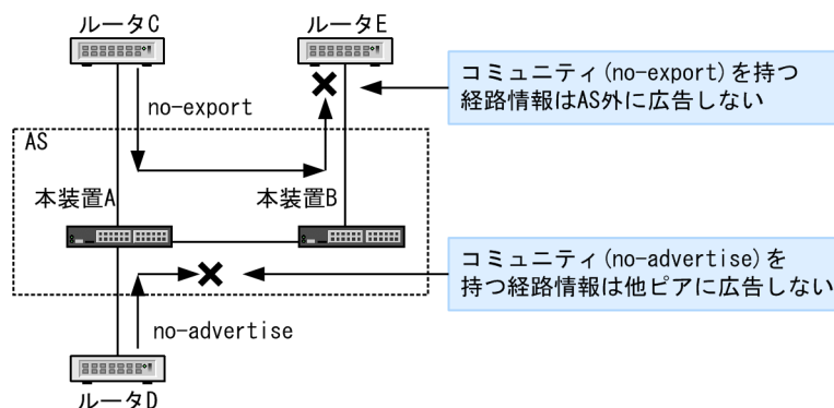
図 13-14 COMMUNITIES 属性を持つ経路情報の広告範囲
