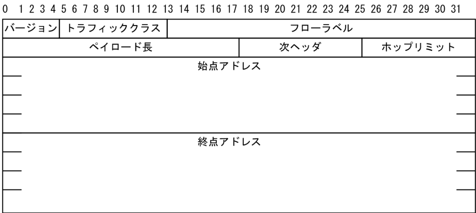
図 18-22 IPv6 ヘッダ形式
