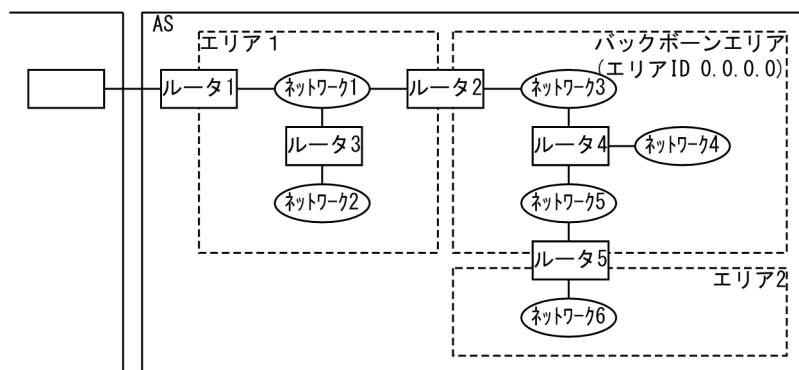
図 12-1 エリア分割を使用した OSPF ネットワークトポロジの例
