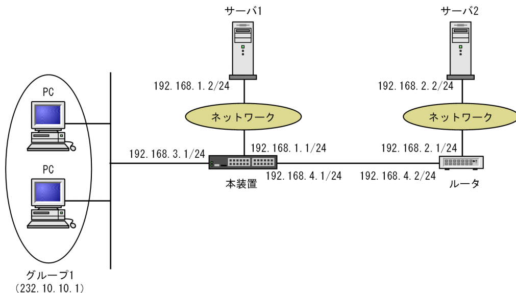
図 16-2 PIM-SSM 構成例
