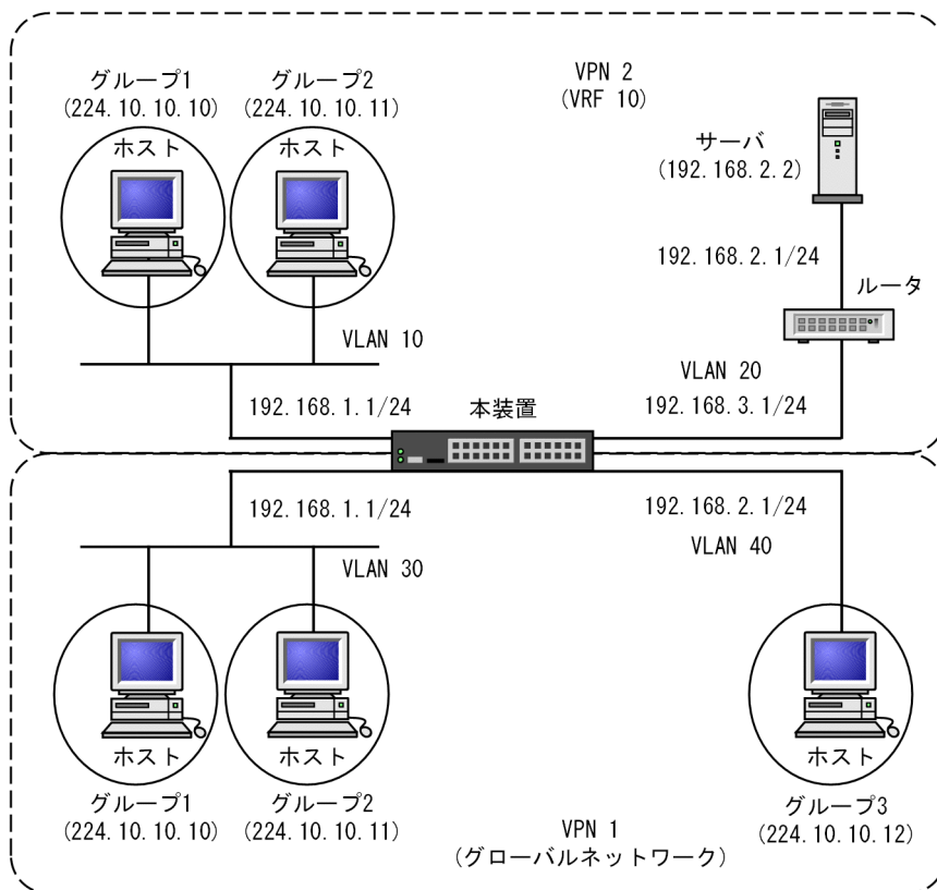
図 16-7 VRF での PIM-SM 構成例（PIM-SM VRF ゲートウェイ）
