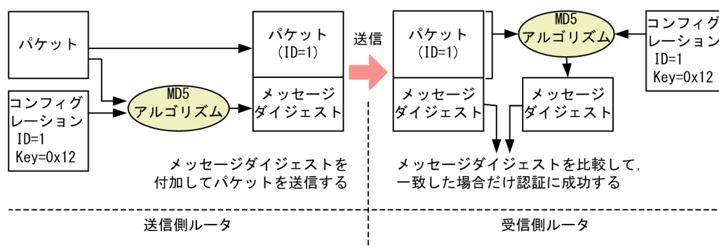
図 12-6 MD5 認証のデータフロー
