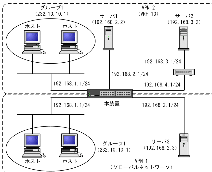
図 16-4 VRF での IPv4 PIM-SSM 構成例
