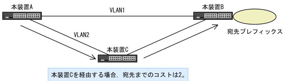
図 27-5 マルチパスの構成
