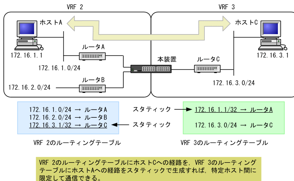
図 8-25 VRF 間にわたるスタティックルーティング
