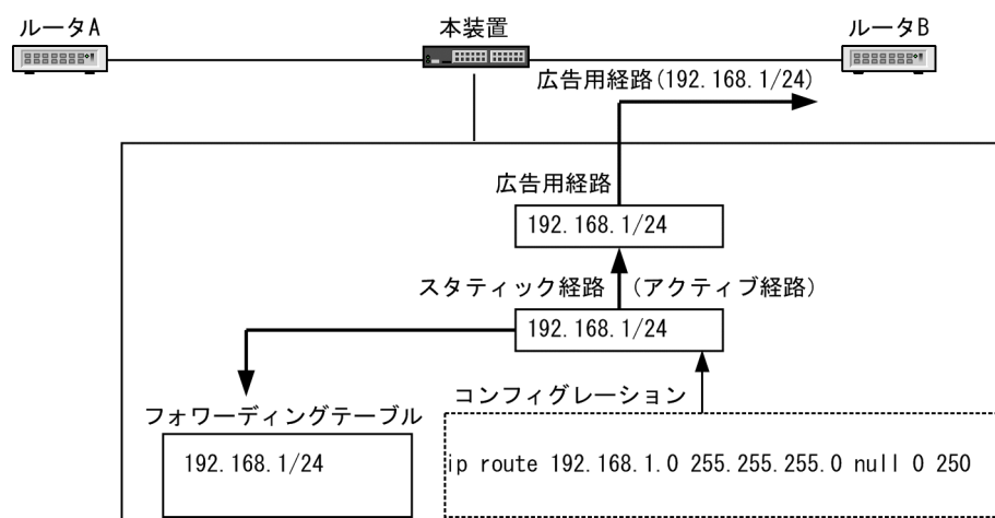
図 13-21 広告用経路生成と広告（BGP4 経路が削除された場合）
