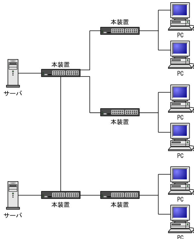
図 15-27 PIM-SSM を使用する構成図
