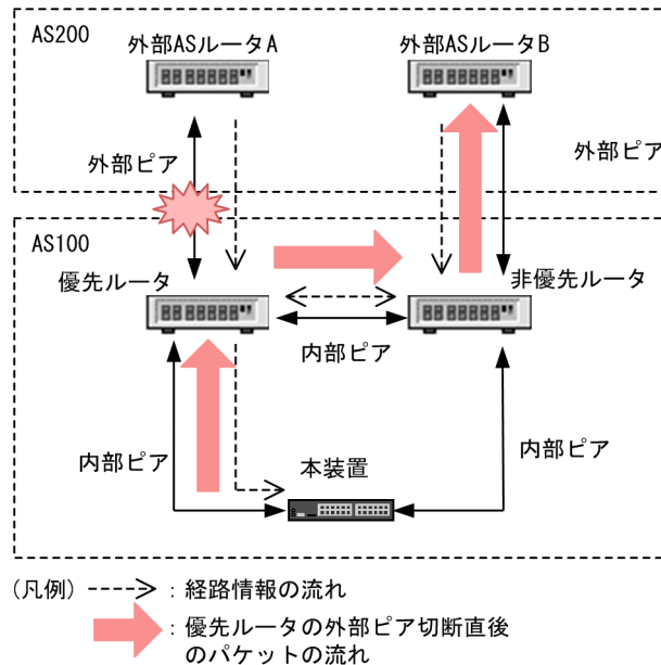
図 8-21 経路削除保留機能の適用例
