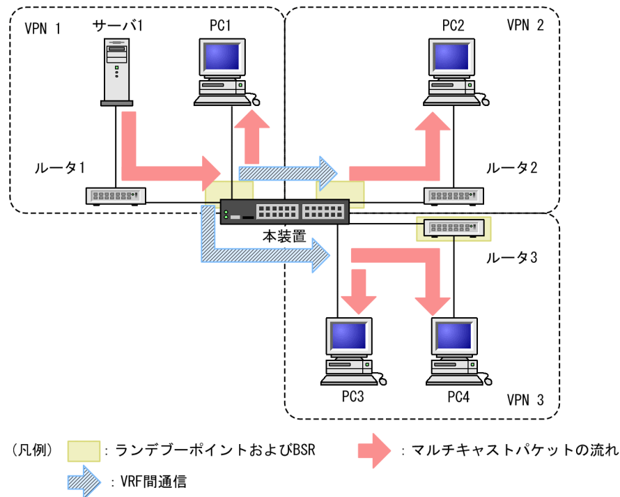
図 15-22 IPv4 マルチキャストエクストラネットの動作概要
