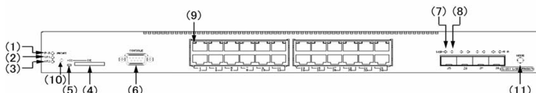
図 1-1 正面パネルレイアウト
