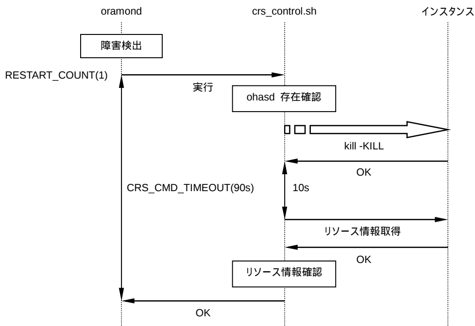
図 4-30 インスタンス監視時の Oracle Clusterware / Oracle Restart リトライ判定シェルスクリプトの動作
