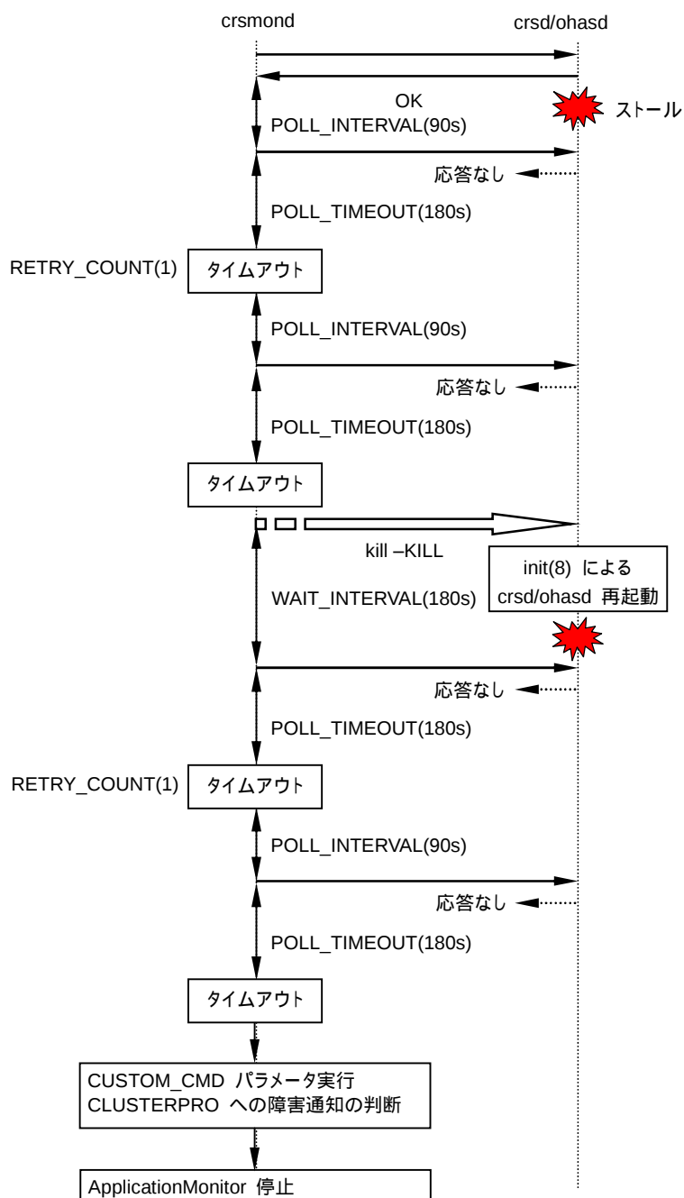
図 4-38 crsd/ohasd 監視タイムアウト時の動作
