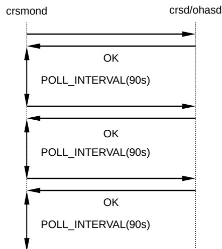
図 4-34 Oracle Clusterware / Oracle Restart 監視時の動作
