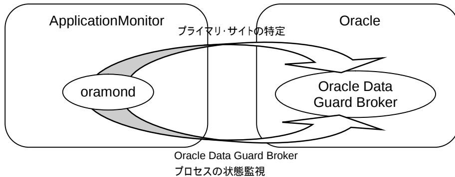
図 4-24 スタンバイ・インスタスの Oracle Data Guard Broker プロセスの状態監視時の概要
