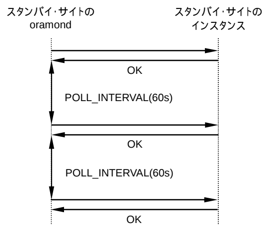
図 4-25 スタンバイ・インスタスの Oracle Data Guard Broker プロセスの状態監視時の動作(一定時間経過による監視)
