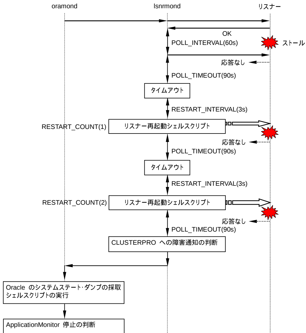
図 4-14 リスナー監視タイムアウト時の動作 (ApplicationMonitor によるリスナー再起動が失敗した場合)
