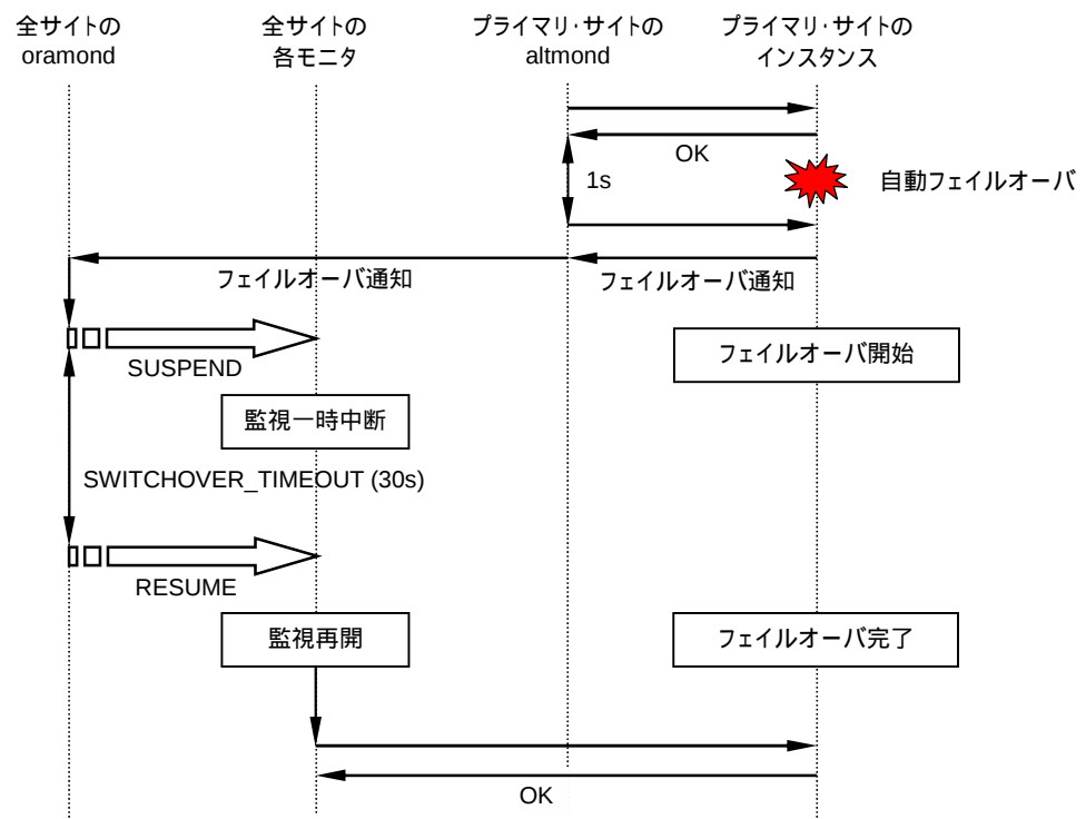
図 4-32 Oracle Data Guard Broker による自動フェイルオーバー時の監視動作
