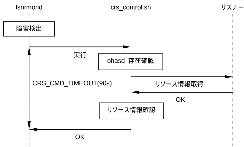
図 4-31 リスナー監視時の Oracle Clusterware / Oracle Restart リトライ判定シェルスクリプトの動作
