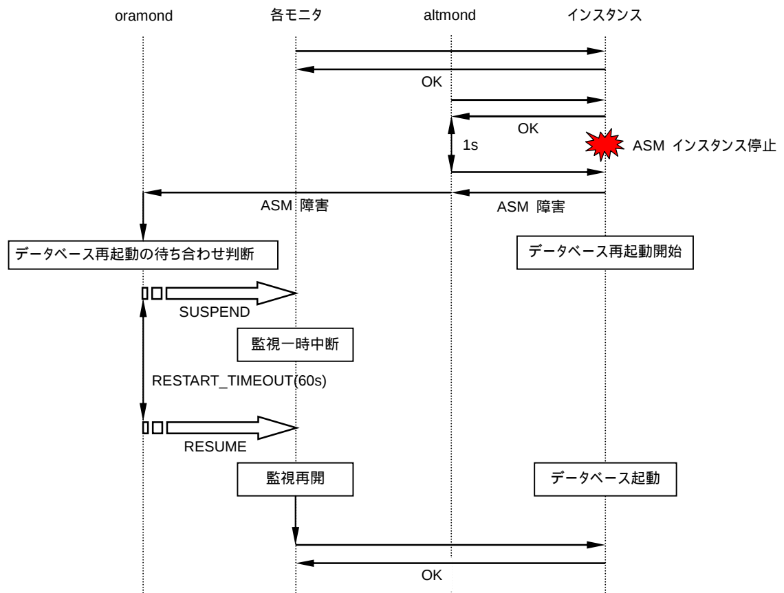
図 4-33 ASM インスタンス停止に伴うデータベースの再起動時の監視動作
