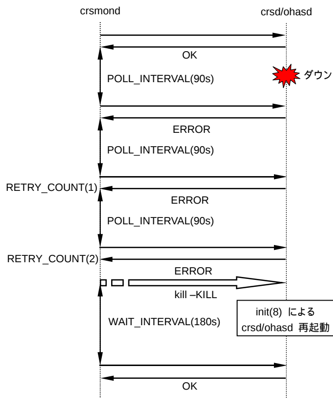
図 4-36 crsd/ohasd 監視エラー時の動作 (init(8) によって crsd/ohasd が再起動された場合)
