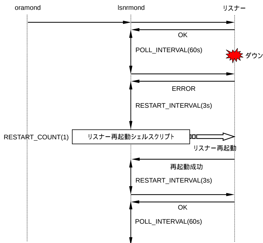
図 4-10 リスナー監視エラー時の動作 (ApplicationMonitor によってリスナーが再起動した場合)
