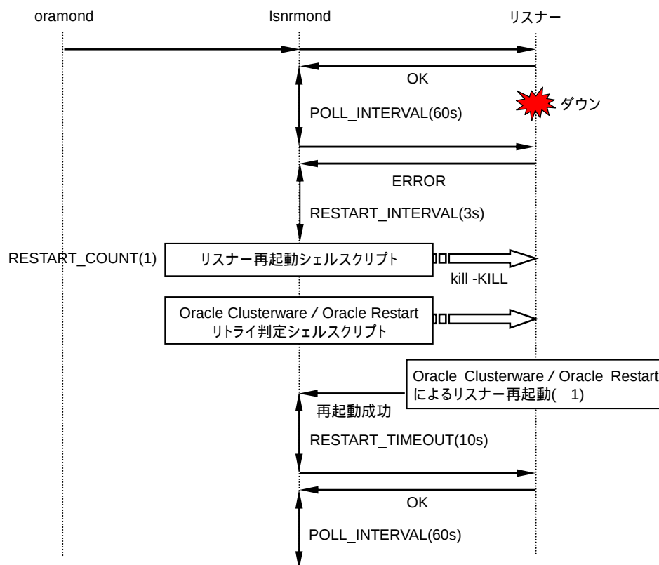
図 4-12 リスナー監視エラー時の動作 (Oracle Clusterware / Oracle Restart によってリスナーが再起動された場合)
