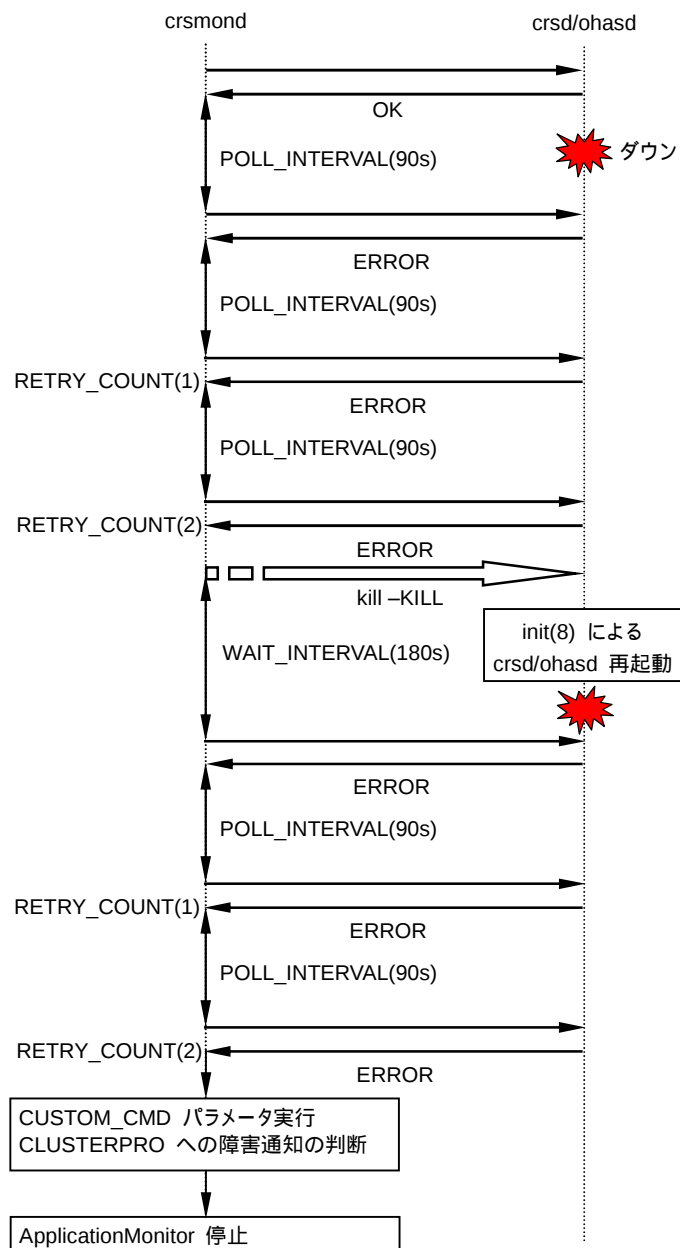
図 4-37 crsd/ohasd 監視エラー時の動作(init(8) によって crsd/ohasd が再起動されなかった場合)
