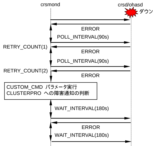
図 4-35 CRS 監視モニタ起動エラー時の動作
