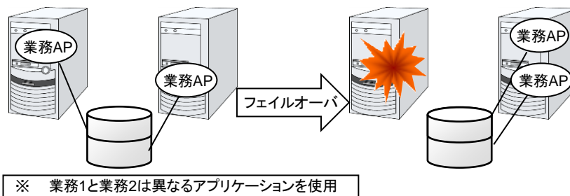
図 2-7 異種アプリケーション双方向スタンバイクラスタ
