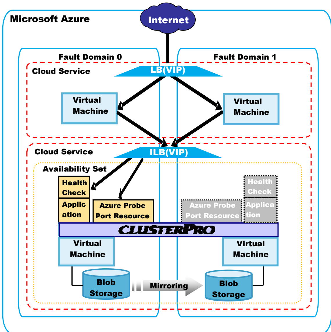
Microsoft Azure 内部負荷分散の場合
