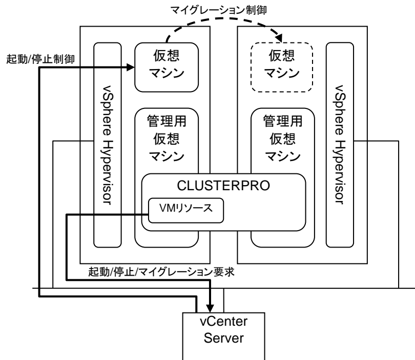
図 2： 管理用の仮想マシン上の OS に CLUSTERPRO をインストールした場合の構成図 (vSphere のみ)
