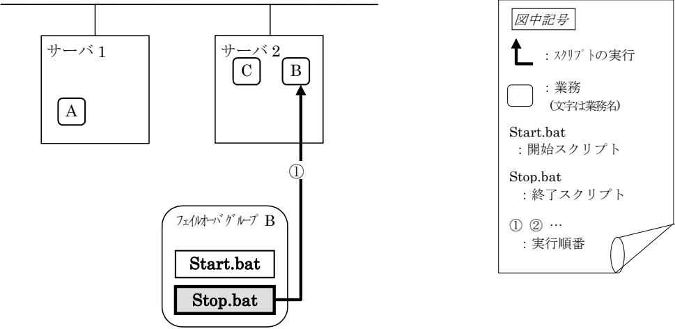
Stop.bat
