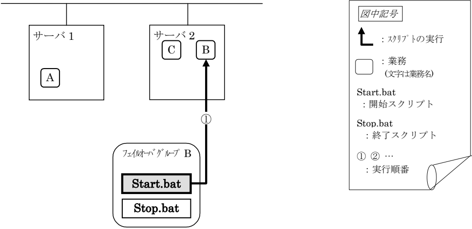
Start.bat
