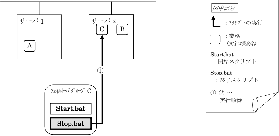
Stop.bat
